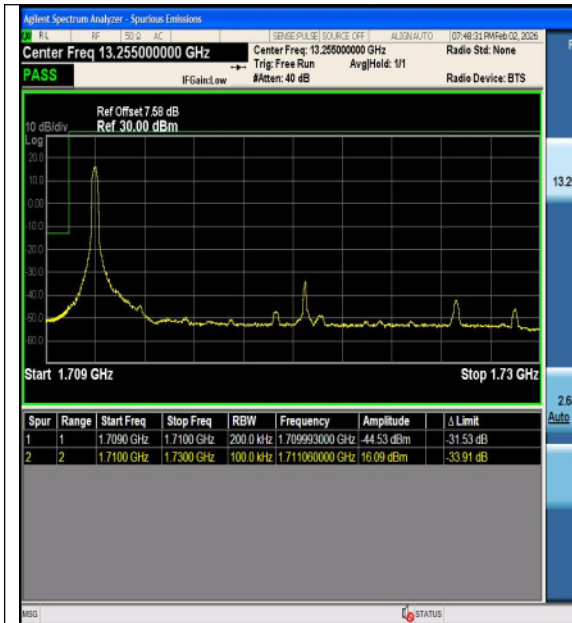
Band4-20MHz-QPSK-20050-100RB#0-PASS
