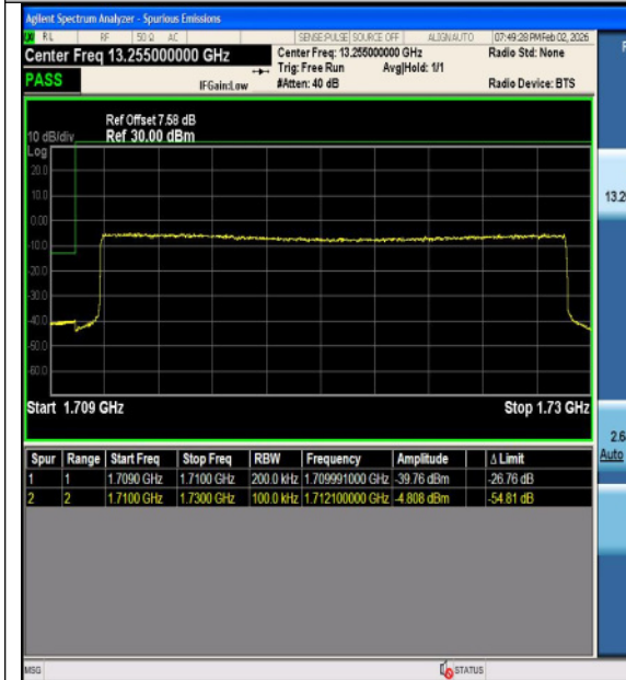
Band4-20MHz-16QAM-20050-1RB#99-PASS
