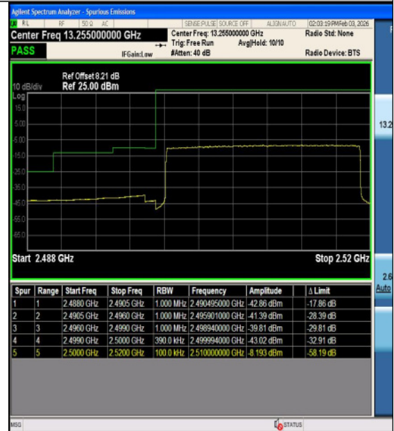
Band7-20MHz-QPSK-21350-1RB#99-PASS
