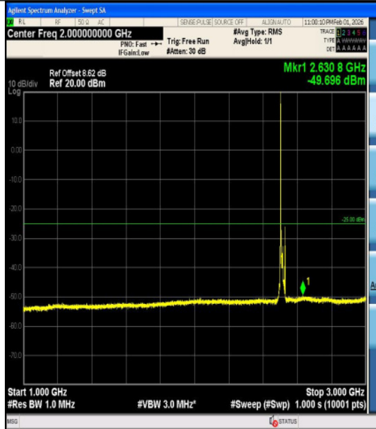
Band7-15MHz-QPSK-20825-1RB#0-18000~270 00-PASS
