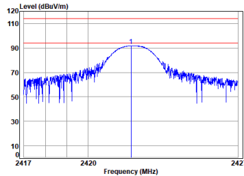
2.4G_SRD_LOW_TX_Horizontal
