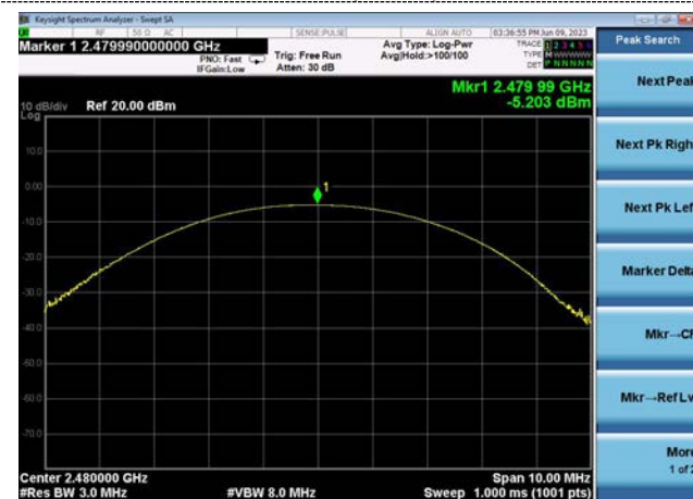
GFSK(CH78)
