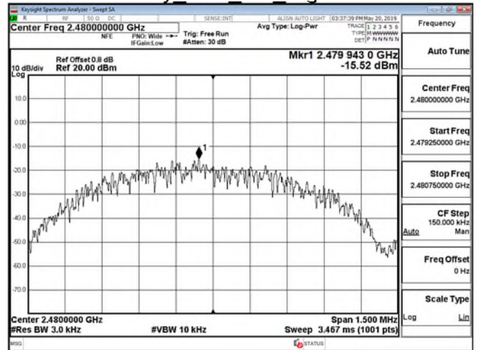
Power Density BLE 1M HighCH39-2480
