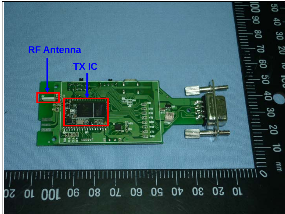
Antenna
