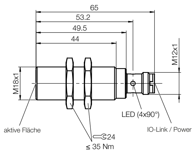
Bild 4-3: Abmessungen und Aufbau BIS M-4A6...
