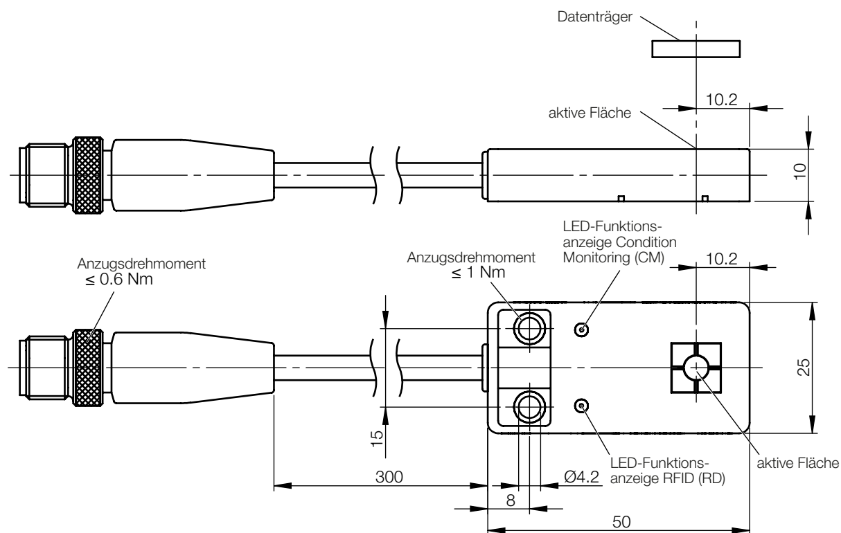
Bild 4-5: Abmessungen und Aufbau BIS M-4A9...
