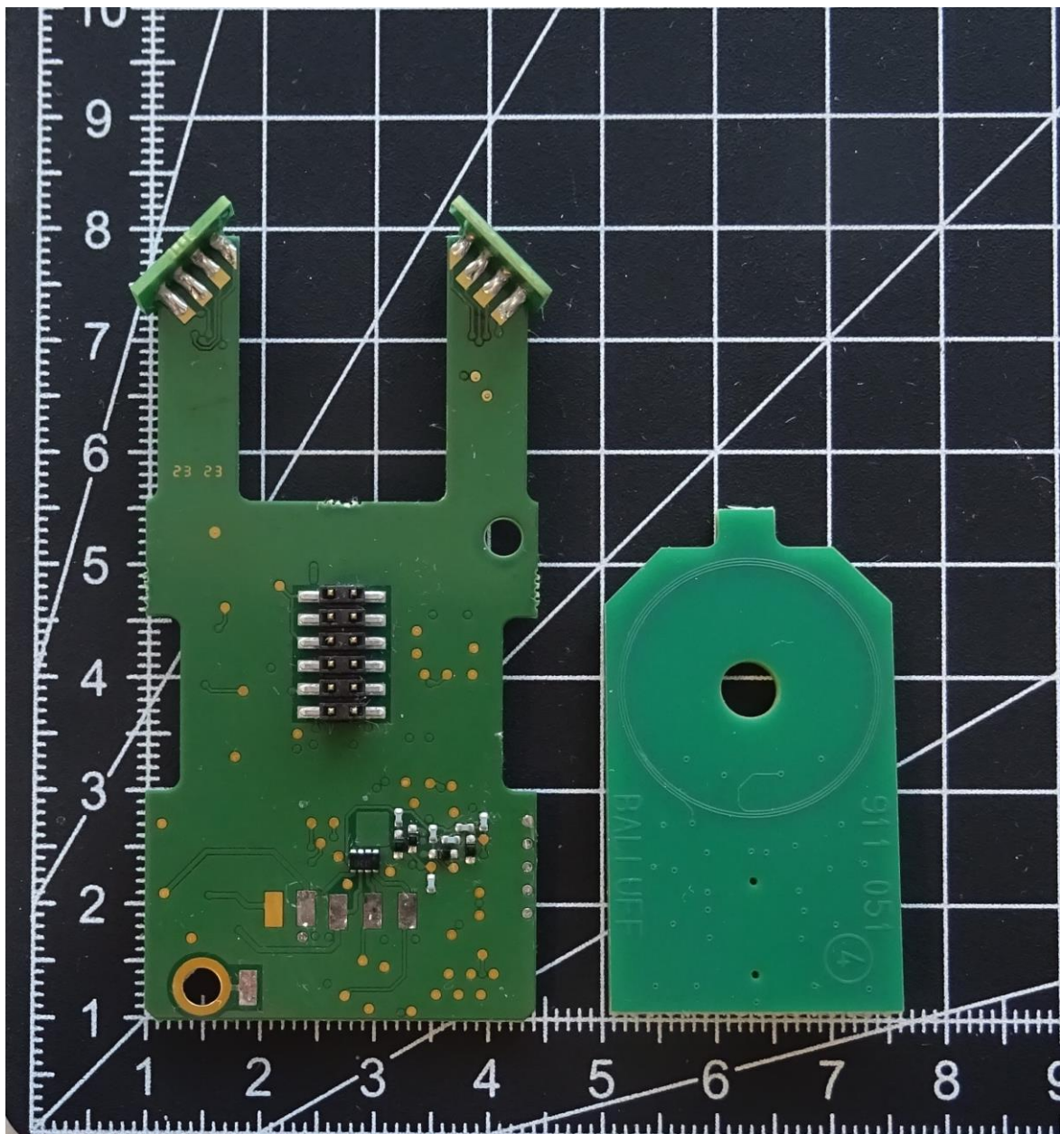
BIS M-408-082-401-07-S4 antenna type B
