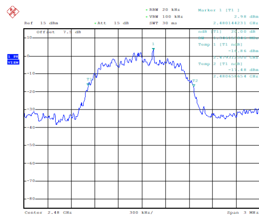
20dB Bandwidth: \pi/4 DQPSK, Ch78
