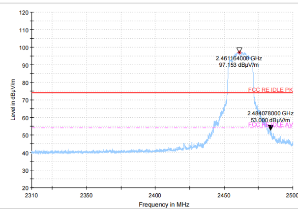
AV detector
