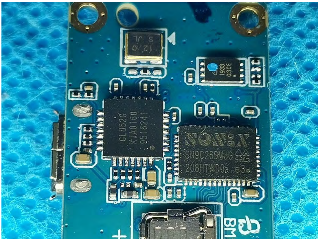
Chip13
