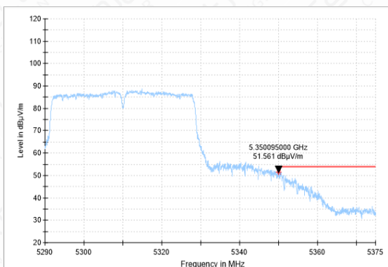
Bandedge-11AC(40M)-CH62-AV
