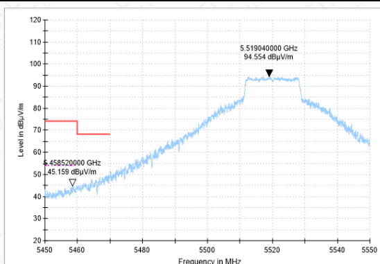
Bandedge-11A-CH104-AV
