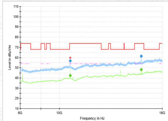
RSE-11N-CH64-8GHz-18GHz
