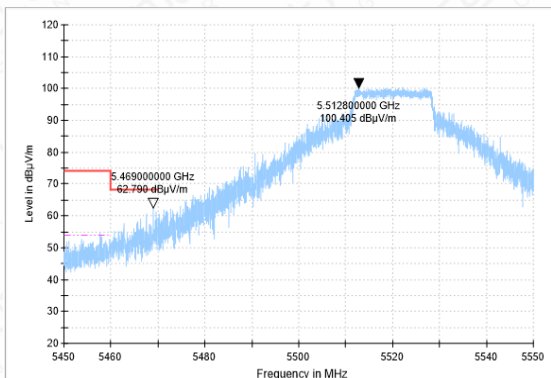
Bandedge-11A-CH104-PK
