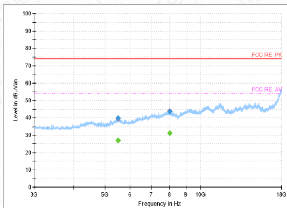
RSE-DH5-CH78-3GHz-18GHz
