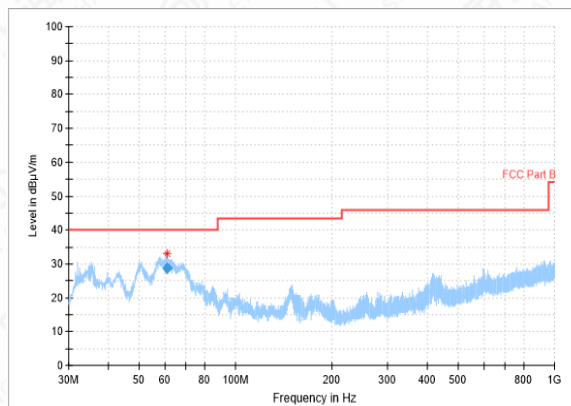
RSE-2DH5-CH78-30MHz-1GHz
