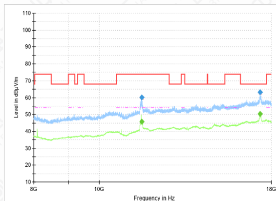
RSE-11AC(80M)-CH155-8GHz-18GHz
