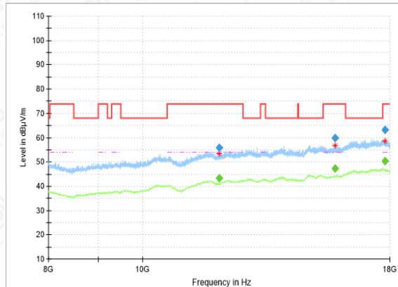
RSE-11AC(80M)-CH155-8GHz-18GHz
