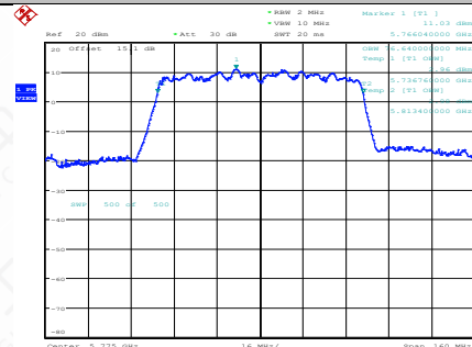
11AC80SISO-Ant1-5775
