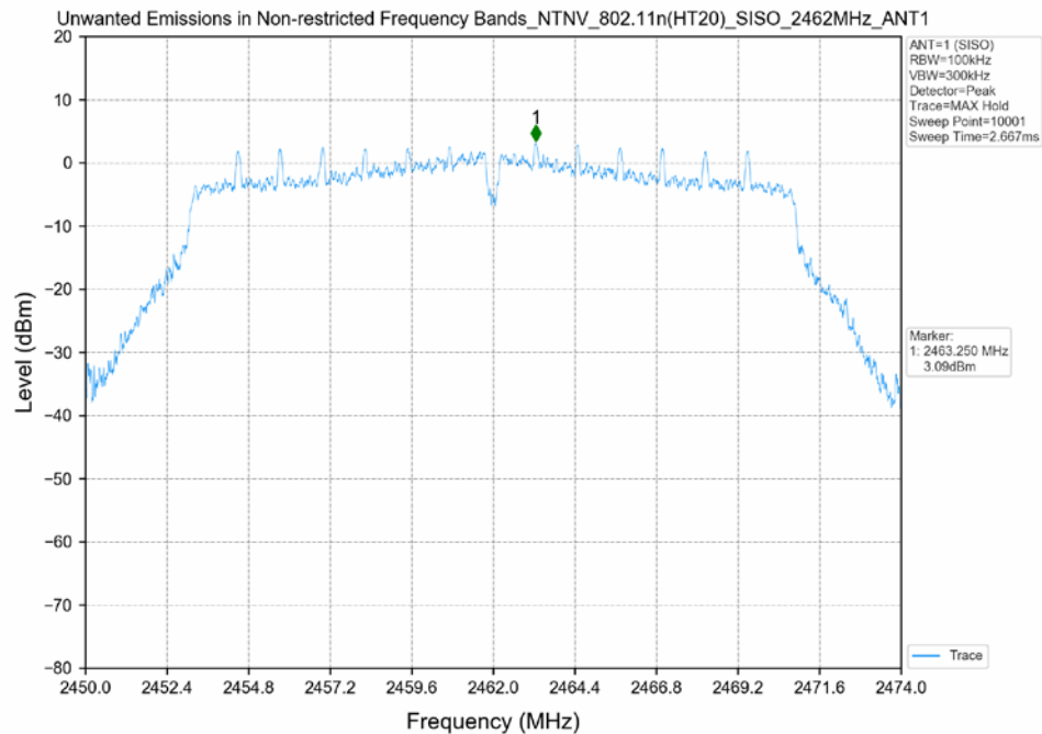
802.11n(HT20)_SISO_ANT1_REF
