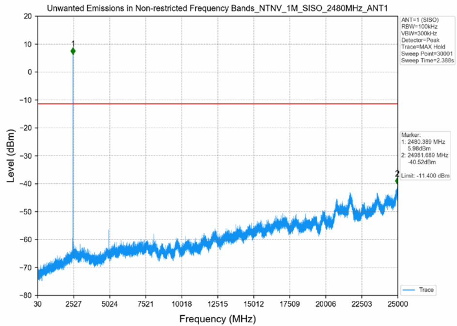
1M_2480MHz_SISO_ANT1
