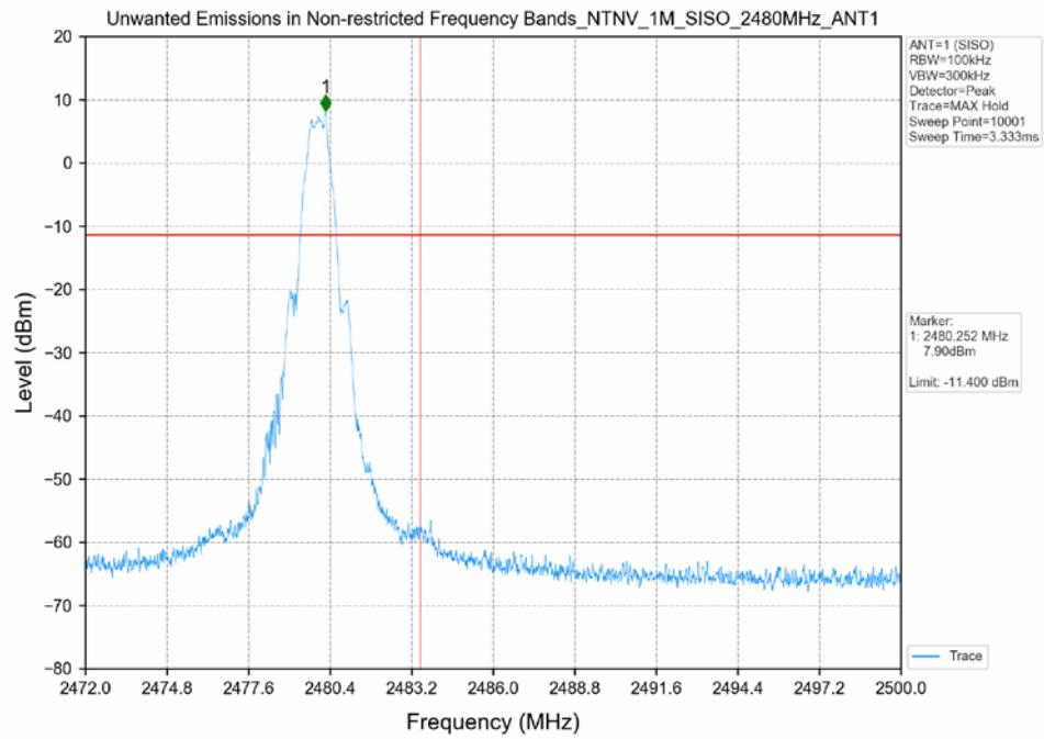
1M_2480MHz_SISO_ANT1
