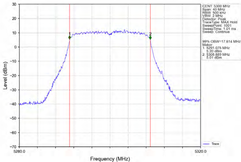
802.11n(HT20)_MCH_5300MHz_Ant2_NTNV
