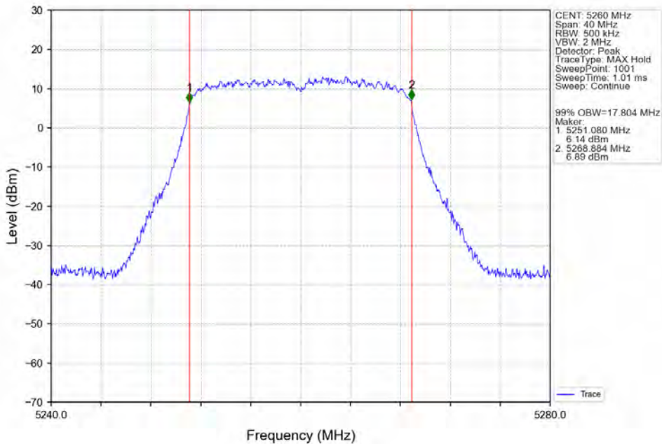
802.11n(HT20)_LCH_5260MHz_Ant2_NTNV
