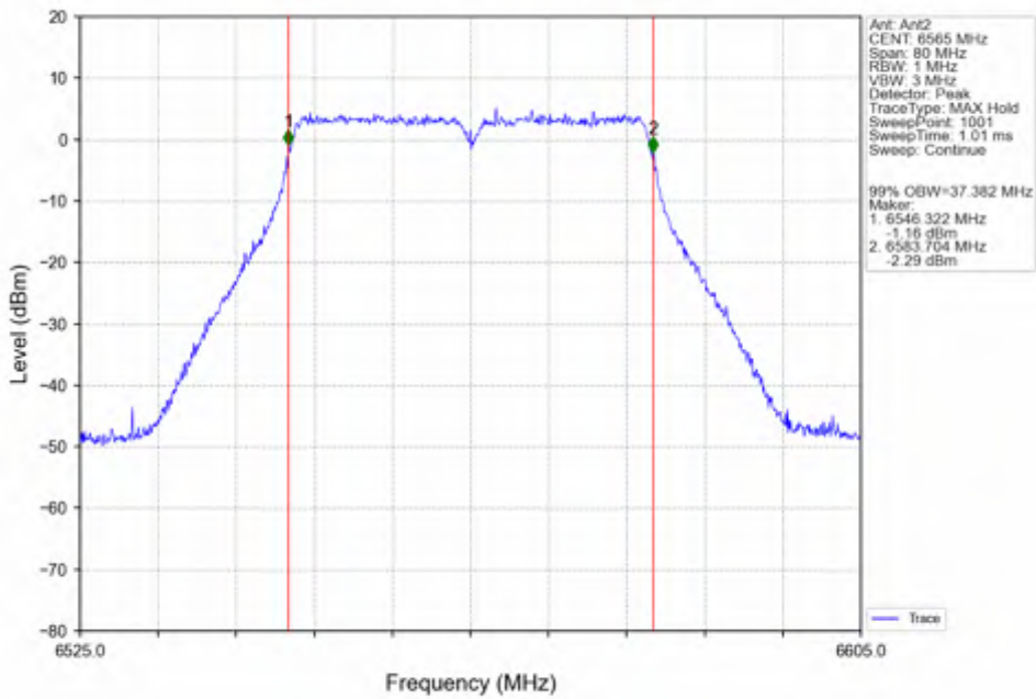
802.11n(HT40) LCH_6565MHz_Ant2_NTNV
