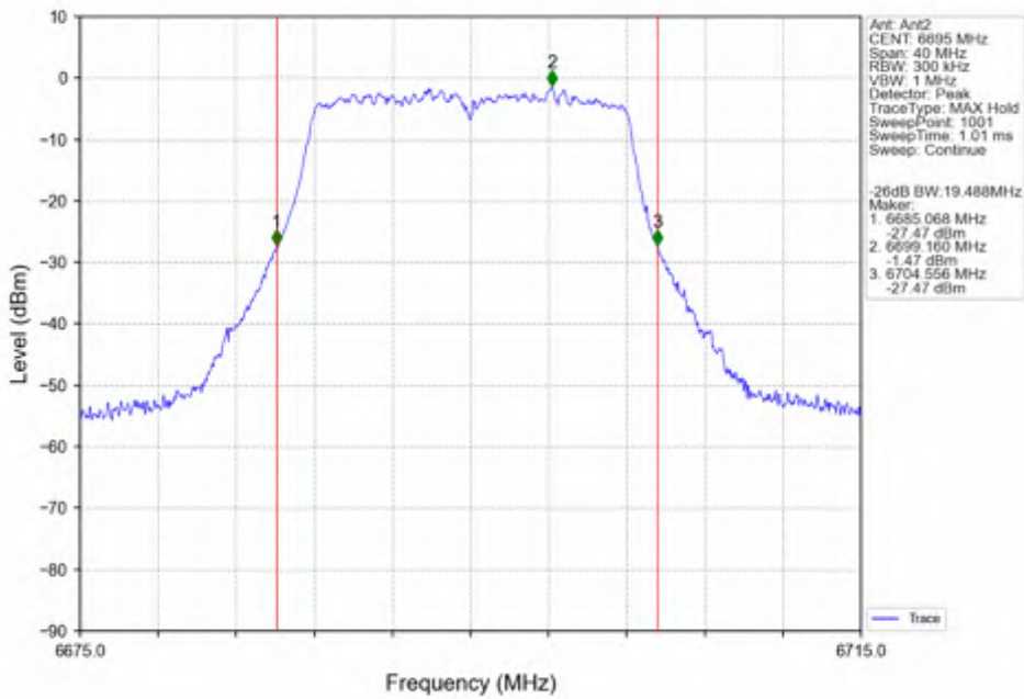
802.11a_MCH_6695MHz_Ant2_NTNV
