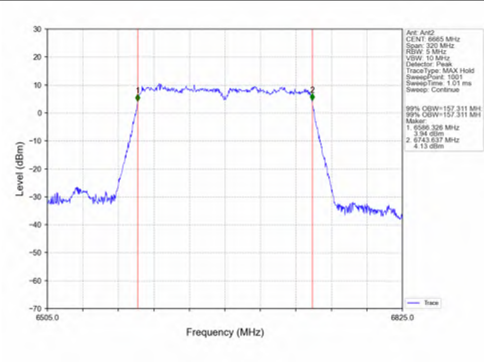
802.11ac(VHT160) MCH_6665MHz_Ant2_NTNV
