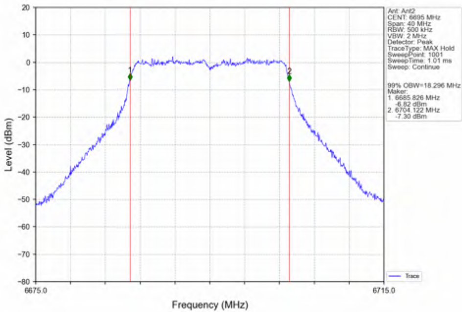
802.11n(HT20)_MCH_6695MHz_Ant2_NTNV
