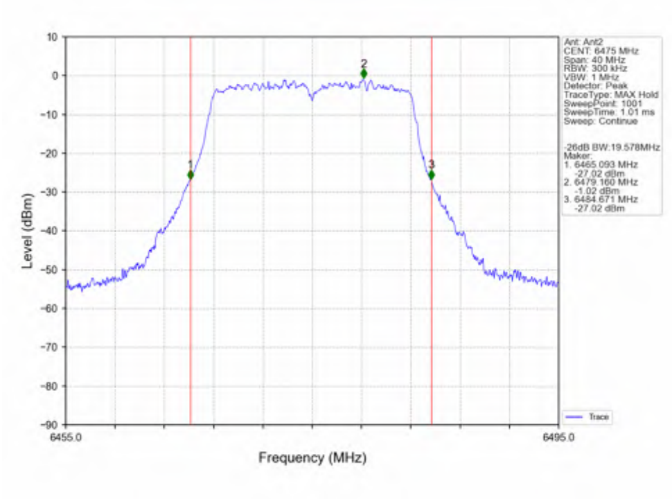
802.11a_MCH_6475MHz_Ant2_NTNV
