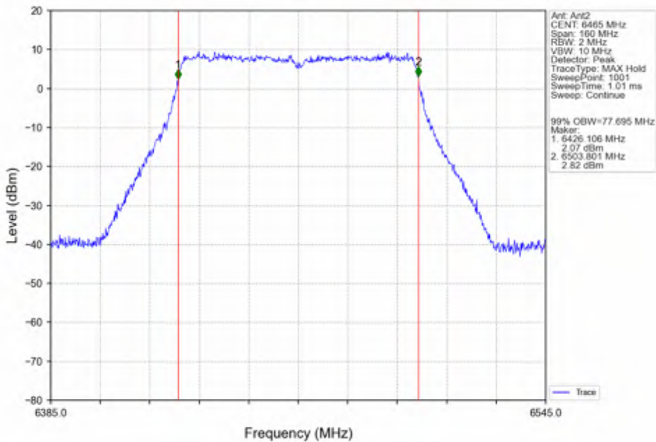
802.11ac(VHT80)_LCH_6465MHz_Ant2_NTNV
