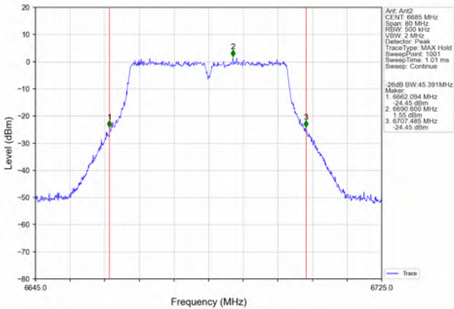
802.11n(HT40)_MCH_6685MHz_Ant2_NTNV
