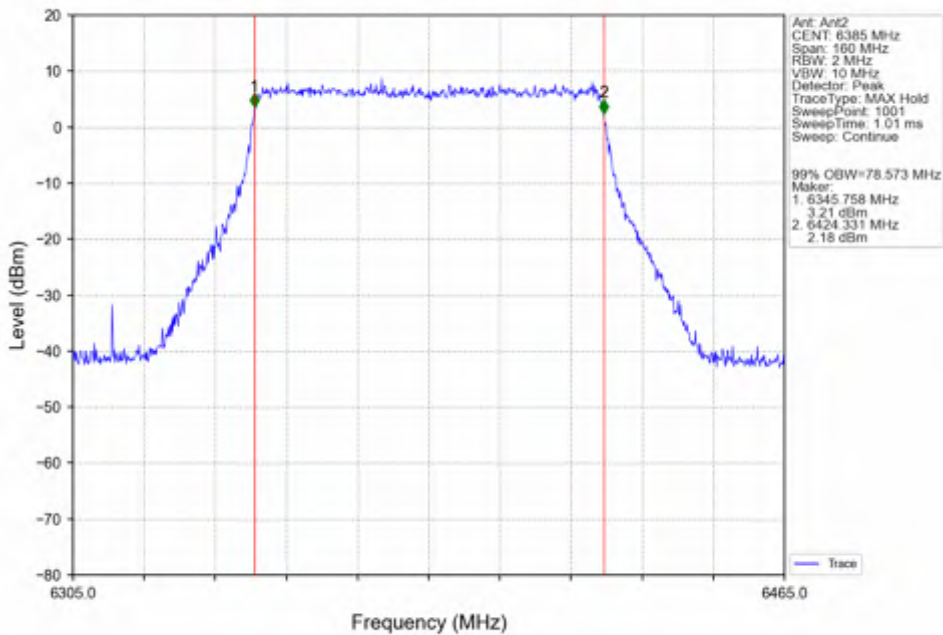
802.11ax(HEW80) HCH_6385MHz_SU / Ant2_NTNV
