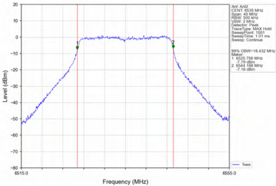
802.11ac(VHT20) LCH_6535MHz_Ant2_NTNV
