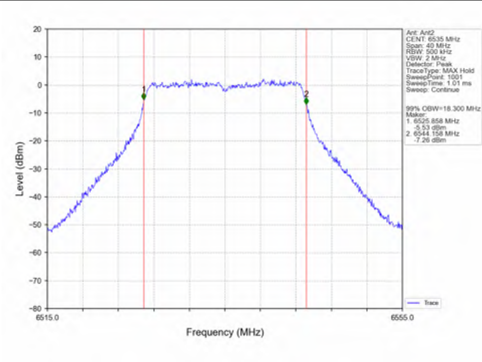
802.11n(HT20) LCH_6535MHz_Ant2_NTNV
