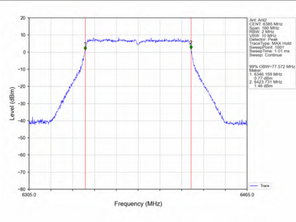
802.11ac(VHT80)_HCH_6385MHz_Ant2_NTNV
