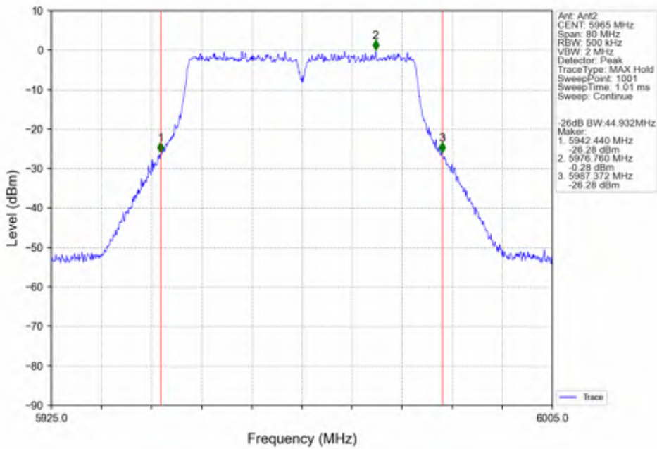
802.11ac(VHT40) LCH_5965MHz_Ant2_NTNV
