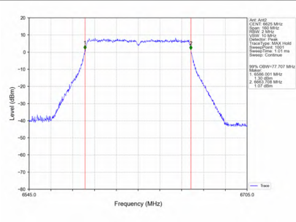
802.11ac(VHT80) LCH_6625MHz_Ant2_NTNV
