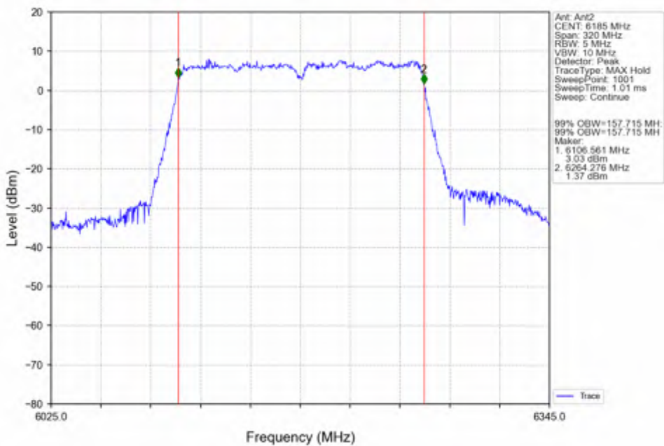
802.11ac(VHT160) MCH_6185MHz_Ant2_NTNV
