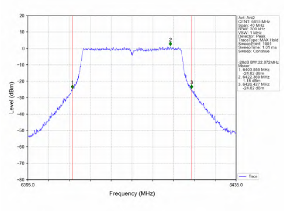
802.11ax(HEW20) HCH 6415MHz SU / Ant2_NTNV
