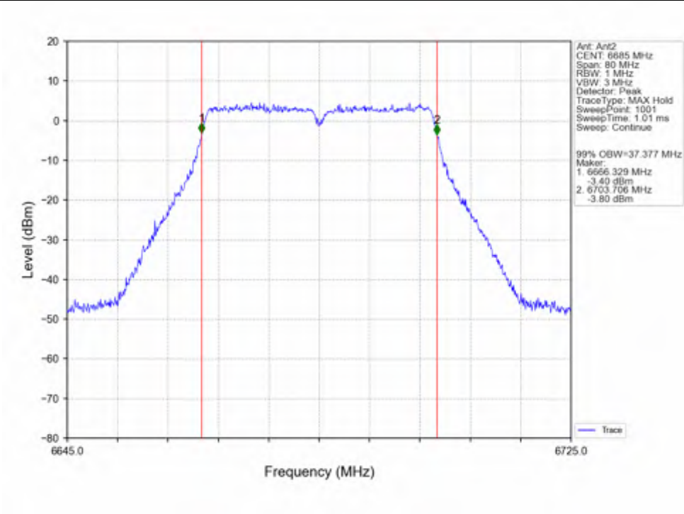
802.11n(HT40)_MCH_6685MHz_Ant2_NTNV
