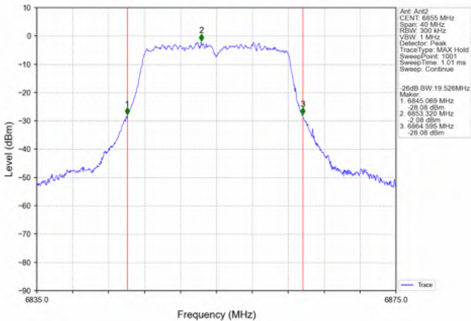
802.11a_HCH_6855MHz_Ant2_NTNV
