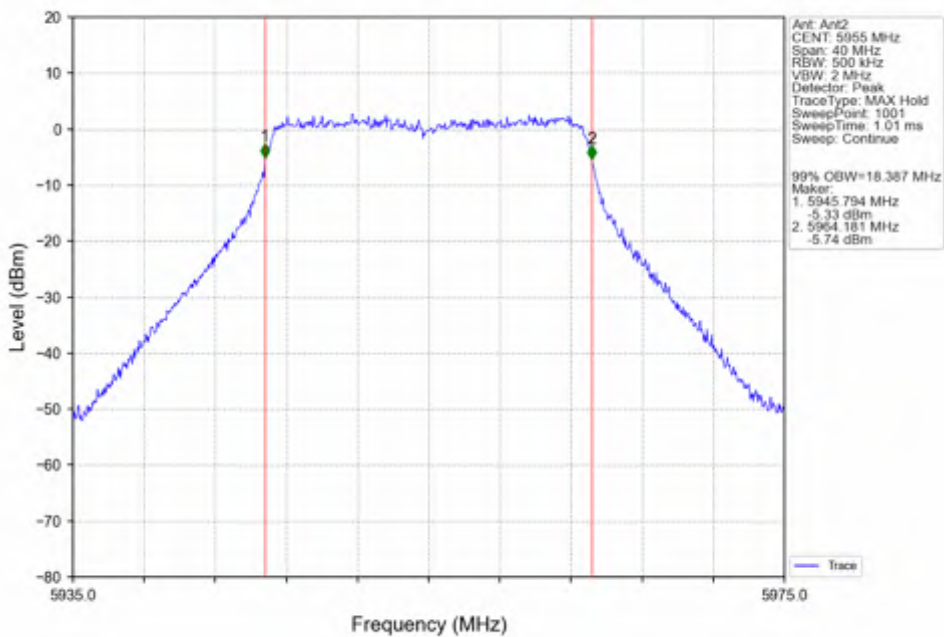
802.11ac(VHT20) LCH_5955MHz_Ant2_NTNV
