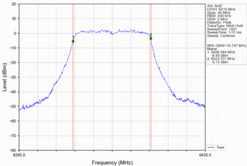
802.11a_HCH_6415MHz_Ant2_NTNV
