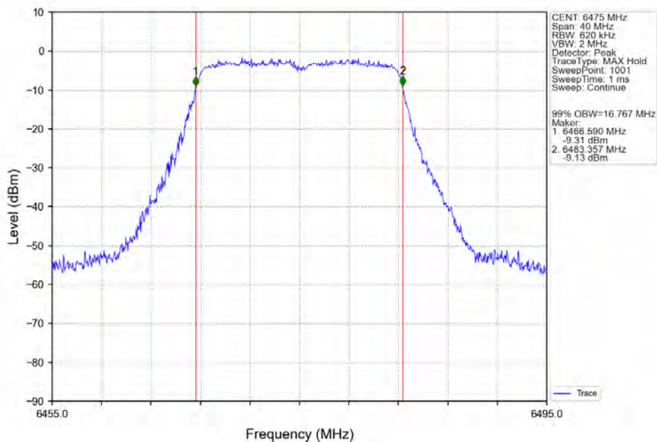
802.11a_MCH_6475MHz_Ant2_NTNV
