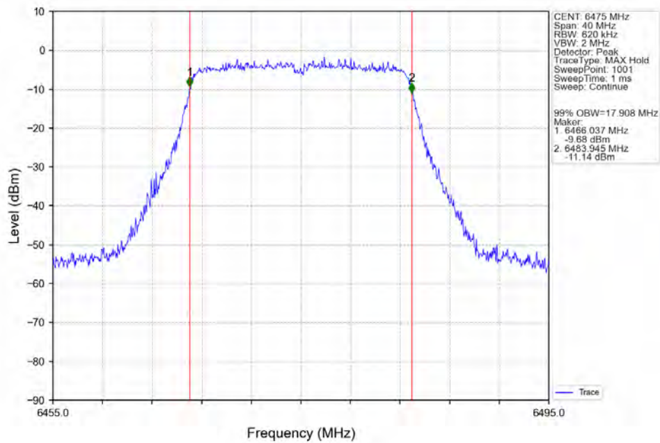
802.11n(HT20) MCH 6475MHz Ant2 NTN
