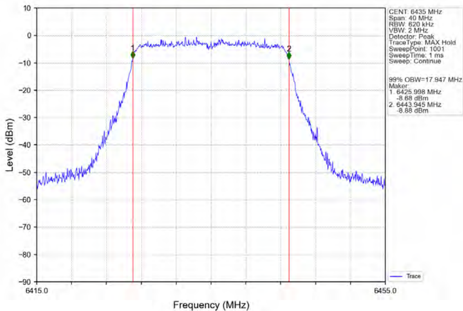
802.11ac(VHT20) LCH_6435MHz_Ant2_NTNV
