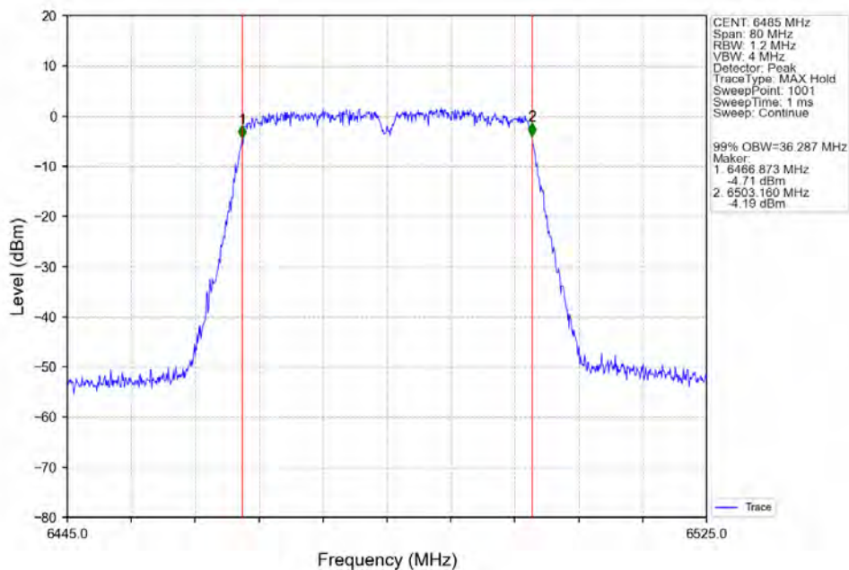
802.11n(HT40) MCH 6485MHz Ant2_NTNV
