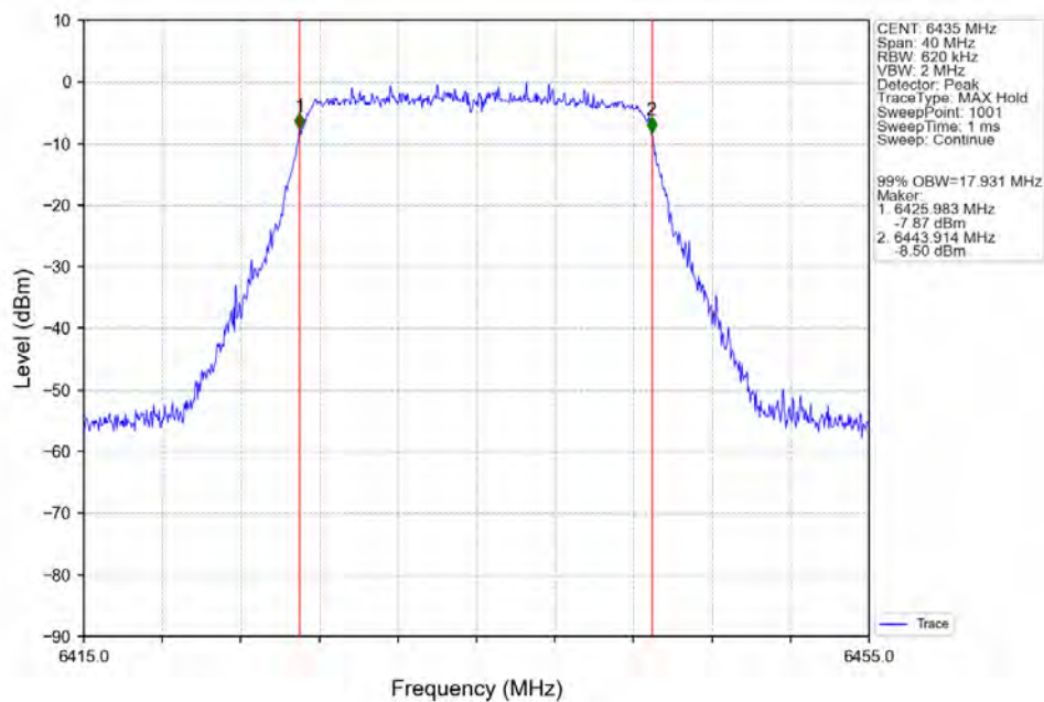
802.11n(HT20) LCH_6435MHz_Ant2_NTNV
