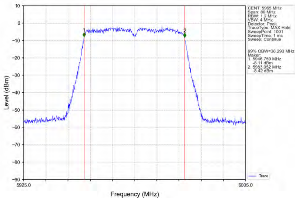
802.11ac(VHT40) LCH_5965MHz_Ant2_NTNV
