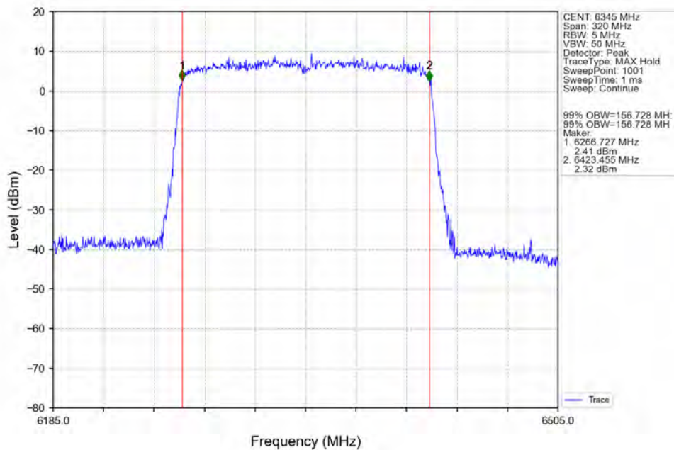
802.11ax(HEW160) HCH 6345MHz SU / Ant2 NTN
