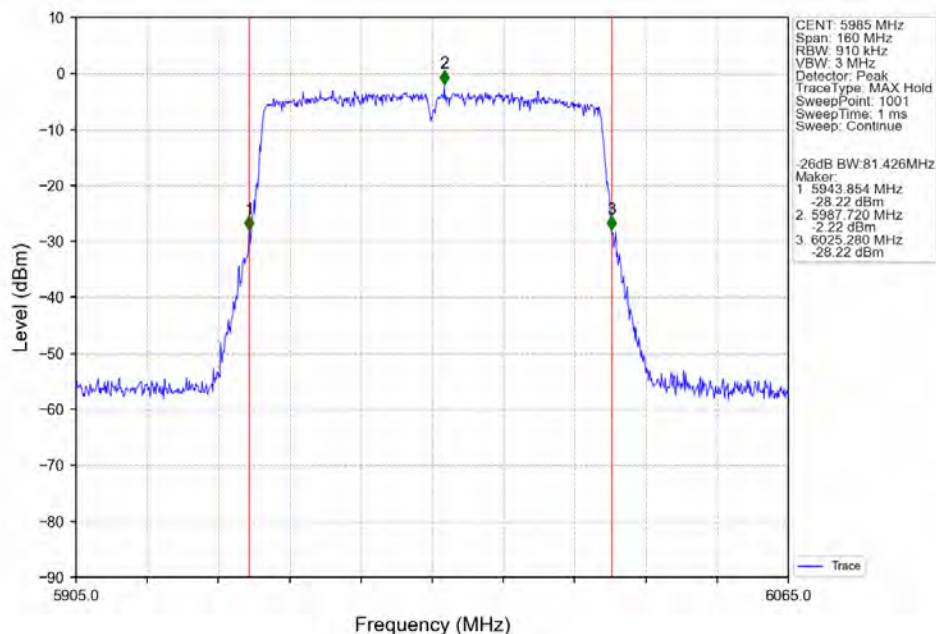
802.11ac(VHT80) LCH_5985MHz_Ant2_NTNV
