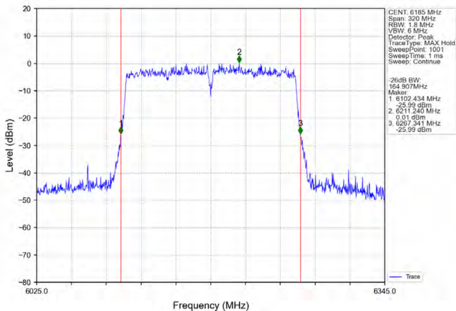
802.11ac(VHT160) MCH_6185MHz_Ant2_NTNV
