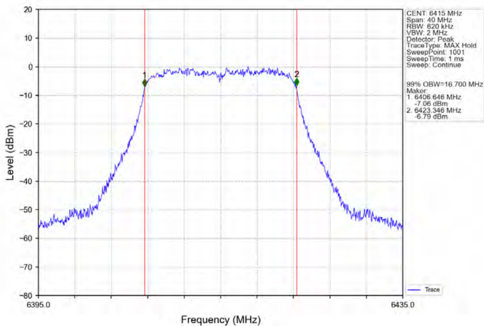
802.11a_HCH_6415MHz_Ant2_NTNV
