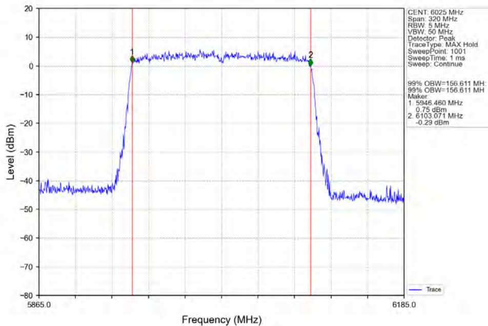
802.11ax(HEW160) LCH 6025MHz SU / Ant2 NTN
