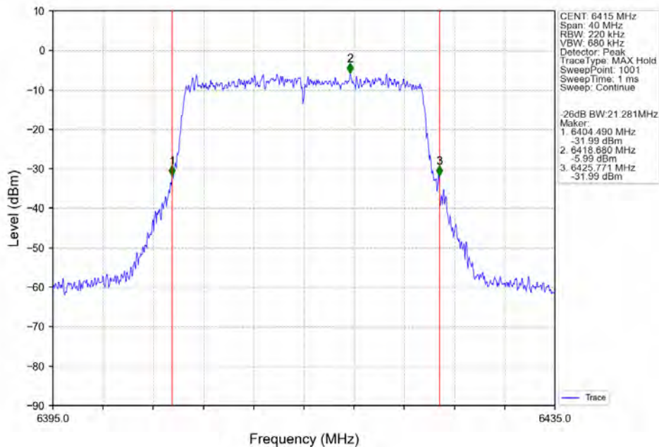
802.11ax(HEW20) HCH 6415MHz SU / Ant2 NTN
