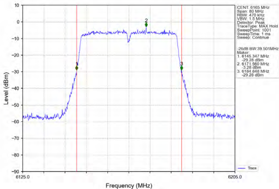
802.11n(HT40) MCH 6165MHz Ant2_NTNV
