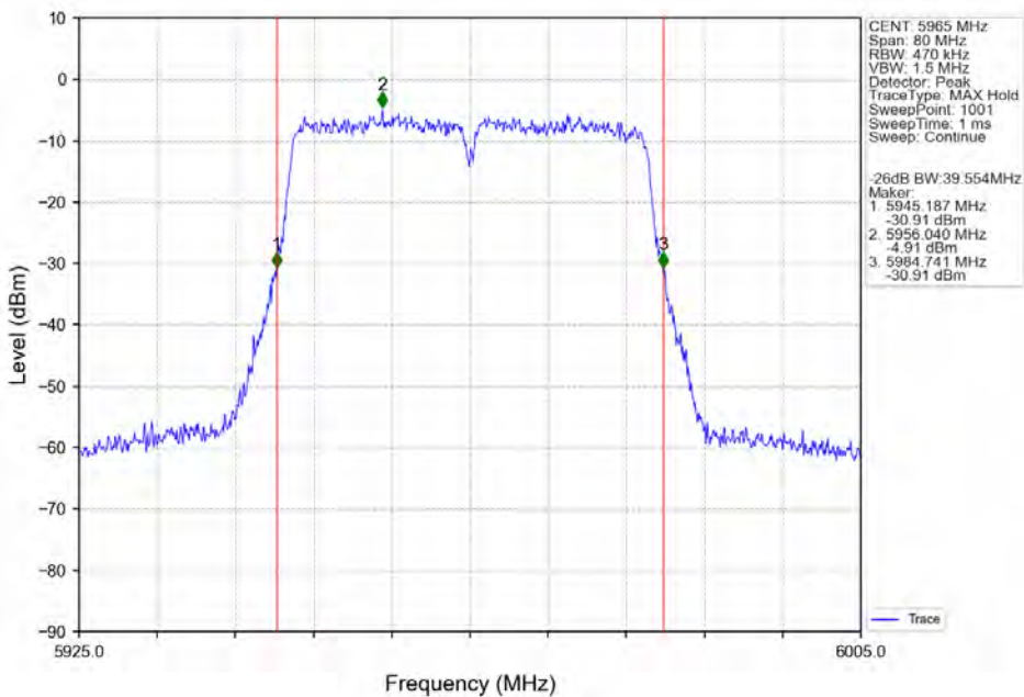
802.11n(HT40) LCH 5965MHz Ant2 NTN
