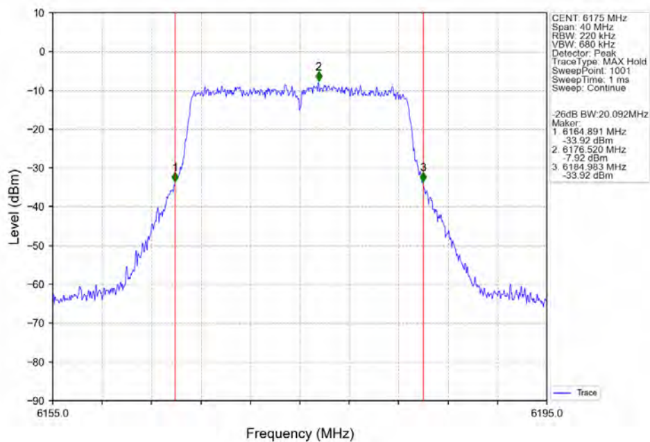
802.11n(HT20) MCH 6175MHz Ant2 NTN
