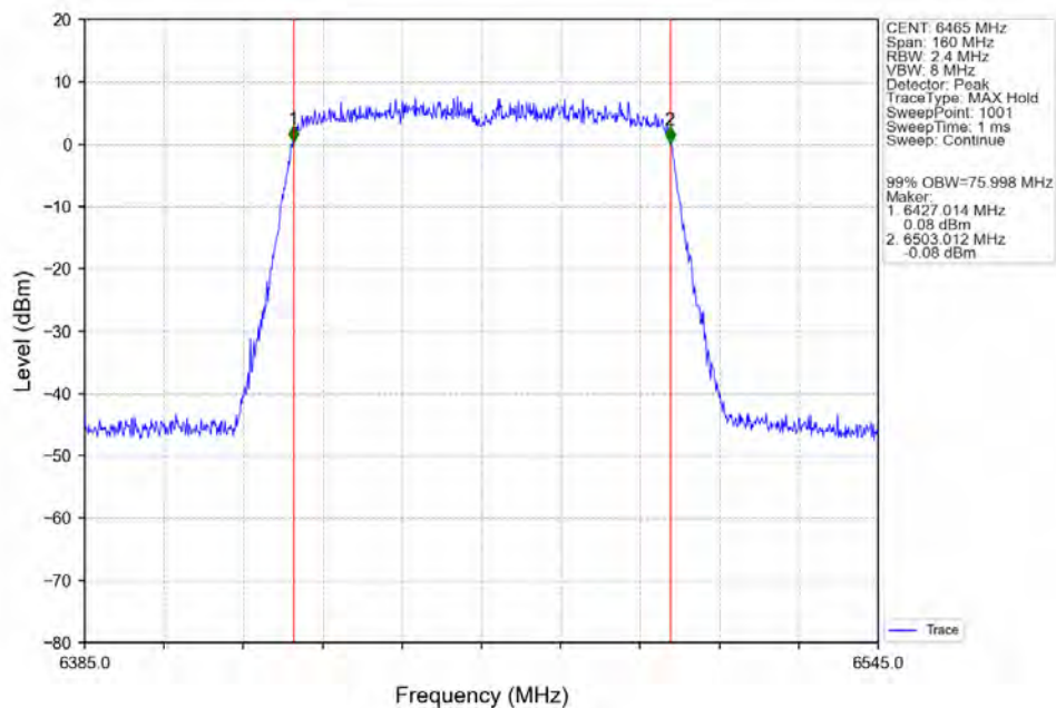
802.11ac(VHT80) LCH_6465MHz_Ant2_NTNV
