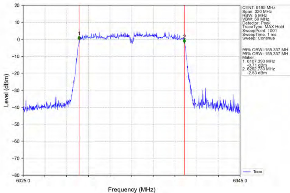
802.11ac(VHT160) MCH_6185MHz_Ant2_NTNV
