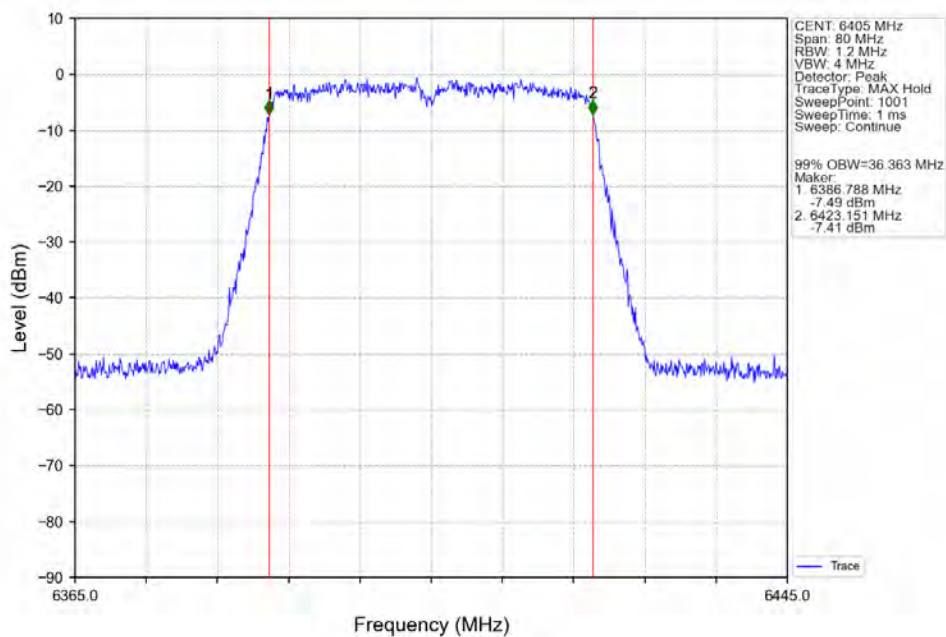
802.11ac(VHT40) HCH 6405MHz Ant2 NTN
