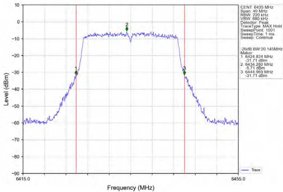
802.11n(HT20) LCH 6435MHz Ant2 NTN
