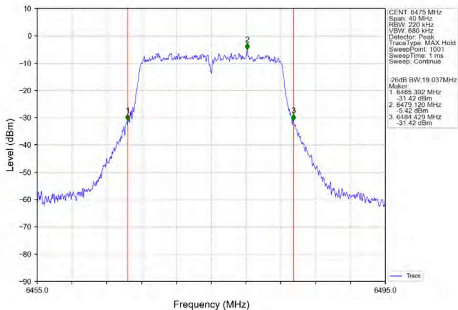
802.11a_MCH_6475MHz_Ant2_NTNV
