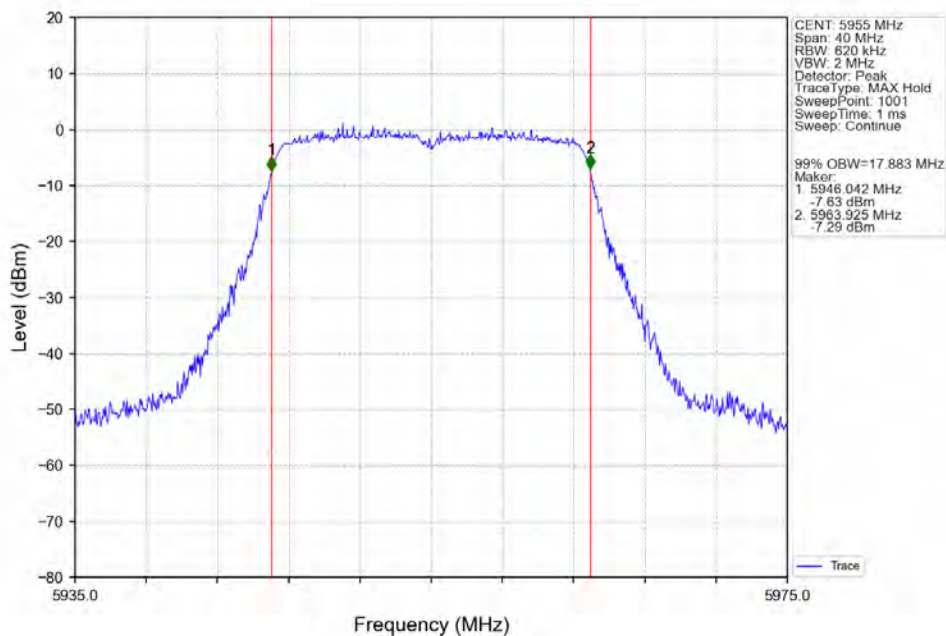
802.11ac(VHT20) LCH_5955MHz_Ant2_NTNV
