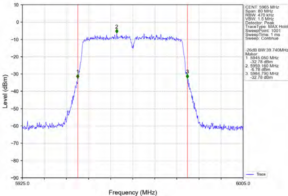
802.11ac(VHT40) LCH_5965MHz_Ant2_NTNV
