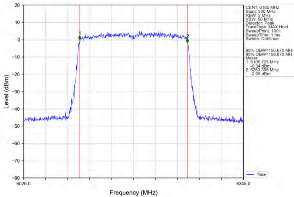
802.11ax(HEW160) MCH 6185MHz SU / Ant2 NTN
