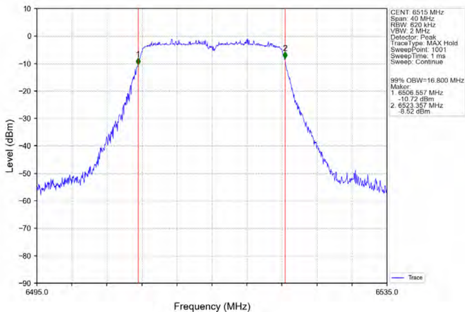
802.11a_HCH_6515MHz_Ant2_NTNV
