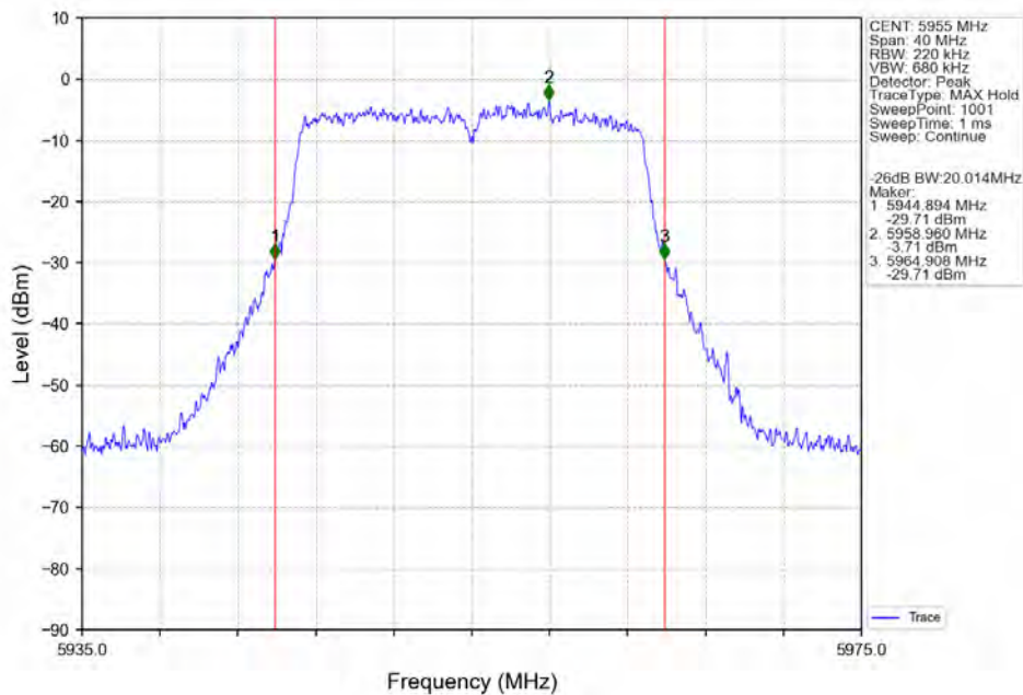
802.11ac(VHT20) LCH_5955MHz_Ant2_NTNV
