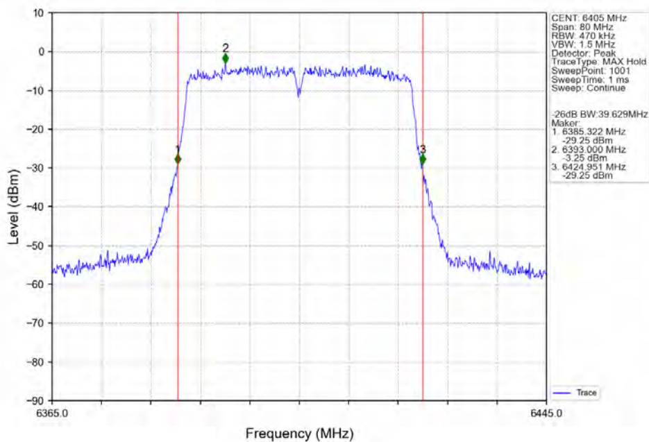
802.11n(HT40) HCH 6405MHz Ant2 NTN
