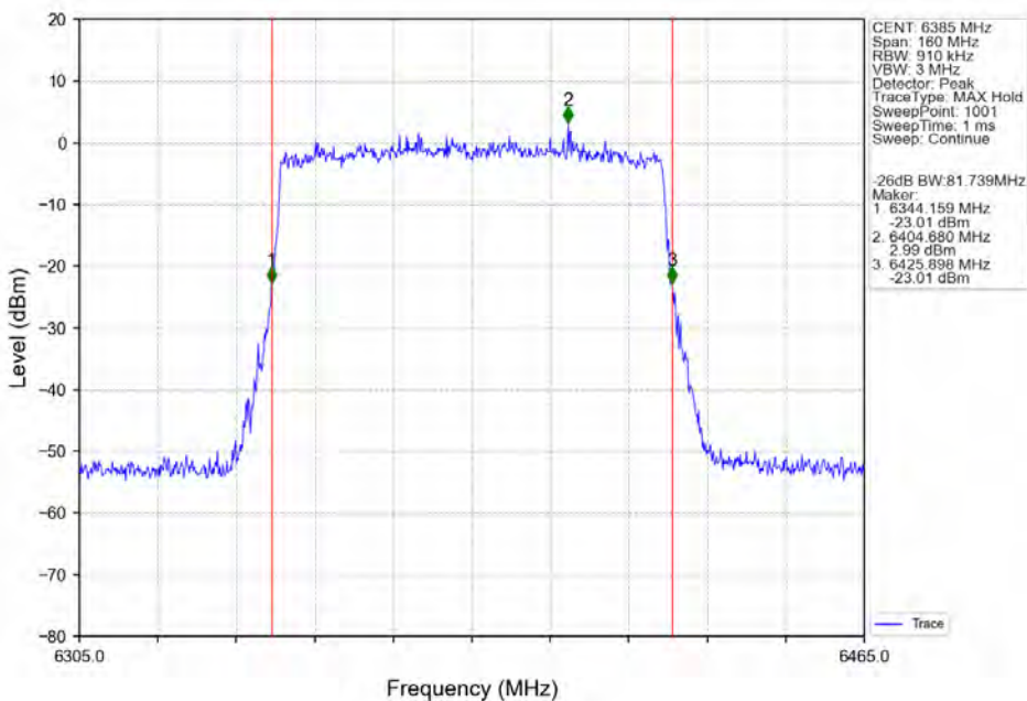
802.11ax(HEW80) HCH 6385MHz SU / Ant2 NTN
