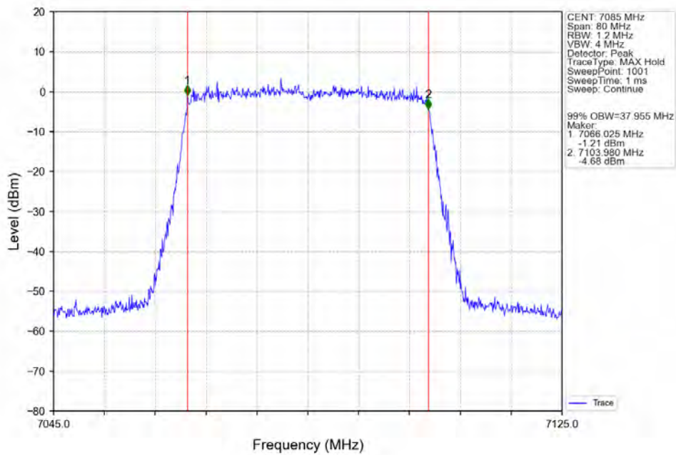
802.11ax(HEW40) HCH 7085MHz SU / Ant2 NTN
