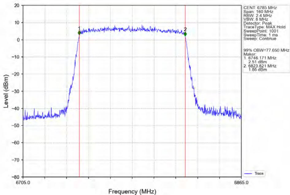
802.11ax(HEW80) HCH 6785MHz SU / Ant2 NTN
