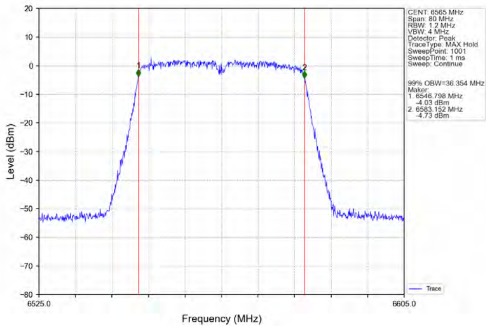
802.11ac(VHT40) LCH_6565MHz_Ant2_NTNV
