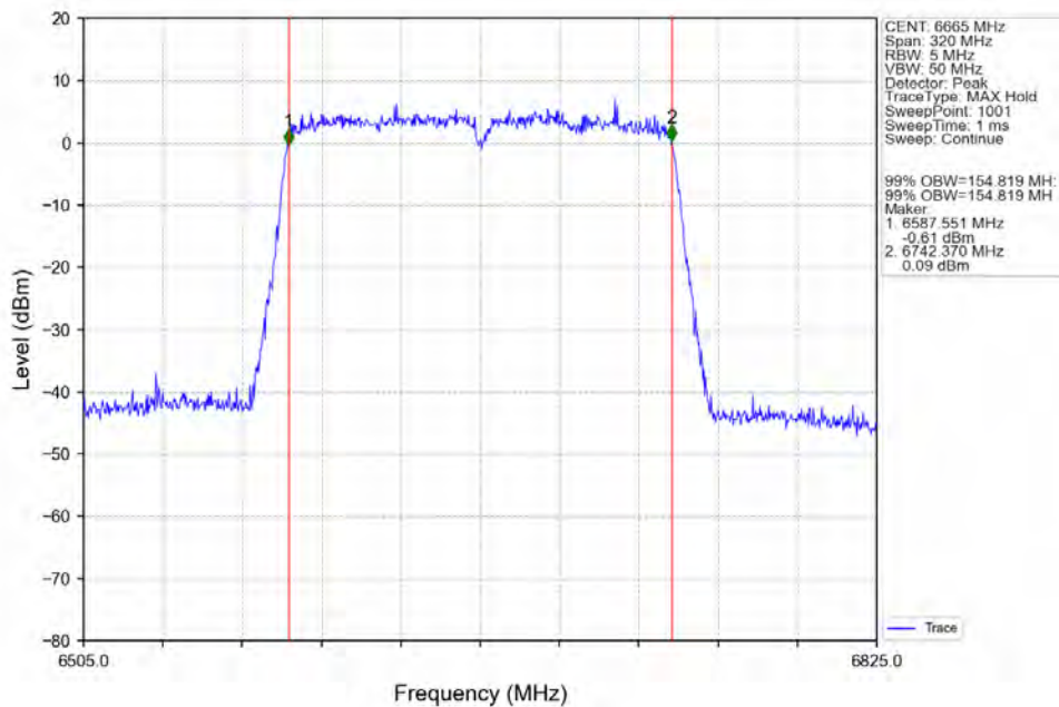
802.11ac(VHT160) MCH_6665MHz_Ant2_NTNV
