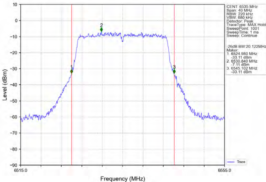
802.11n(HT20) LCH_6535MHz_Ant2_NTNV
