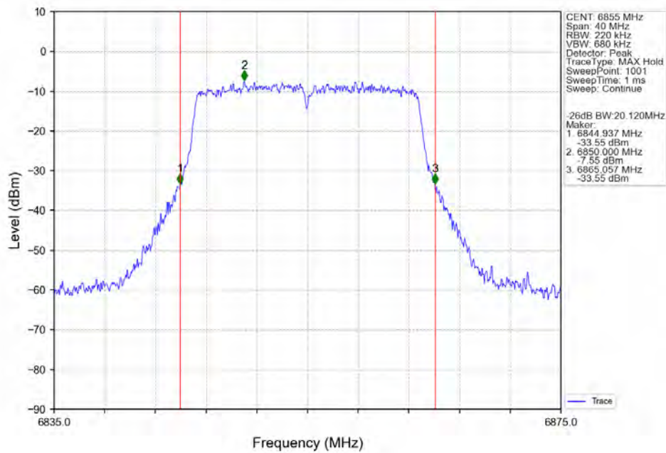
802.11n(HT20) HCH 6855MHz Ant2 NTN
