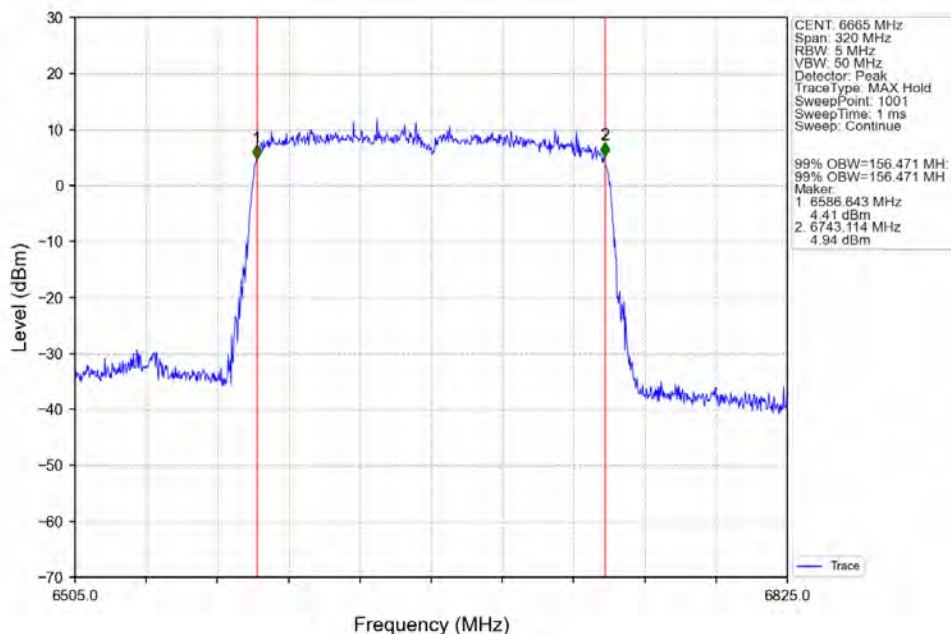
802.11ax(HEW160) MCH 6665MHz SU / Ant2 NTN
