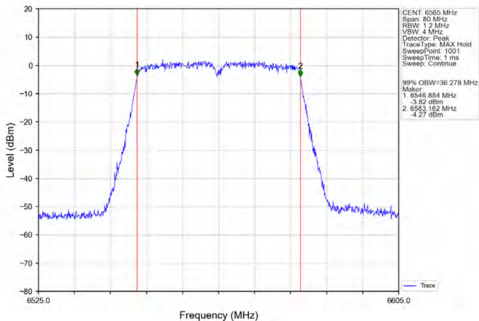
802.11n(HT40) LCH_6565MHz_Ant2_NTNV
