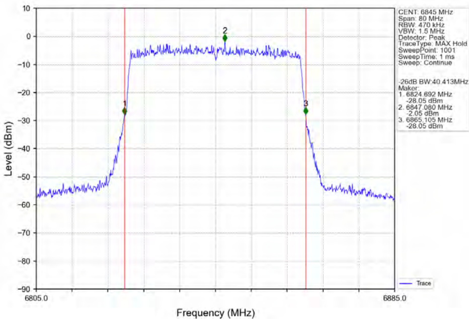
802.11ax(HEW40) HCH 6845MHz SU / Ant2 NTN
