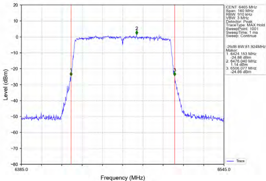
802.11ac(VHT80) LCH_6465MHz_Ant2_NTNV
