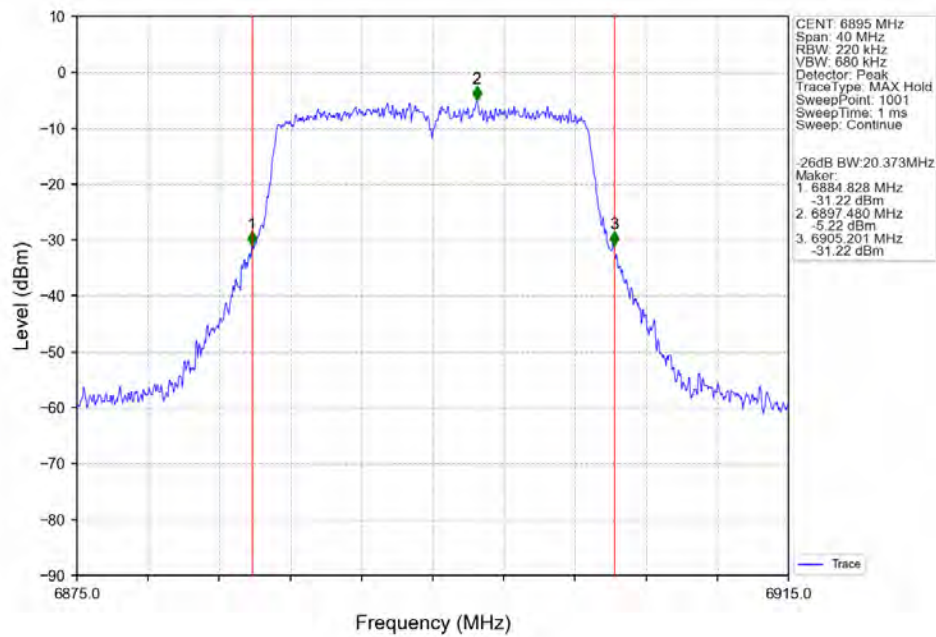
802.11ac(VHT20) LCH 6895MHz Ant2 NTN
