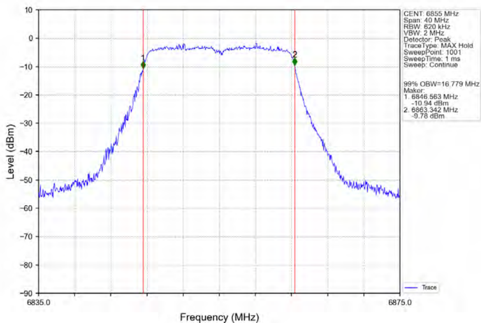
802.11a_HCH_6855MHz_Ant2_NTNV
