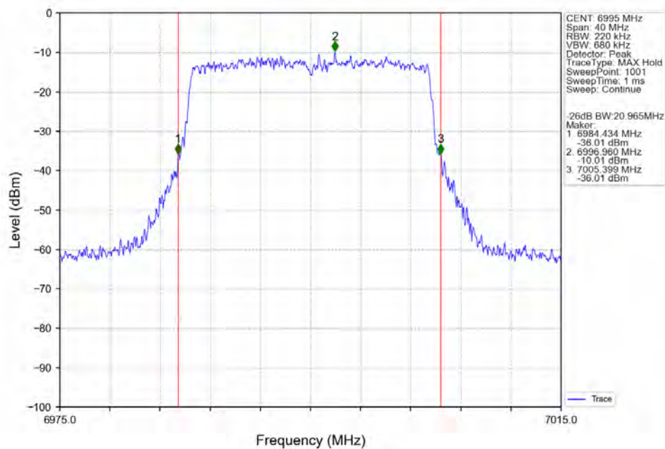
802.11ax(HEW20) MCH 6995MHz SU / Ant2 NTN
