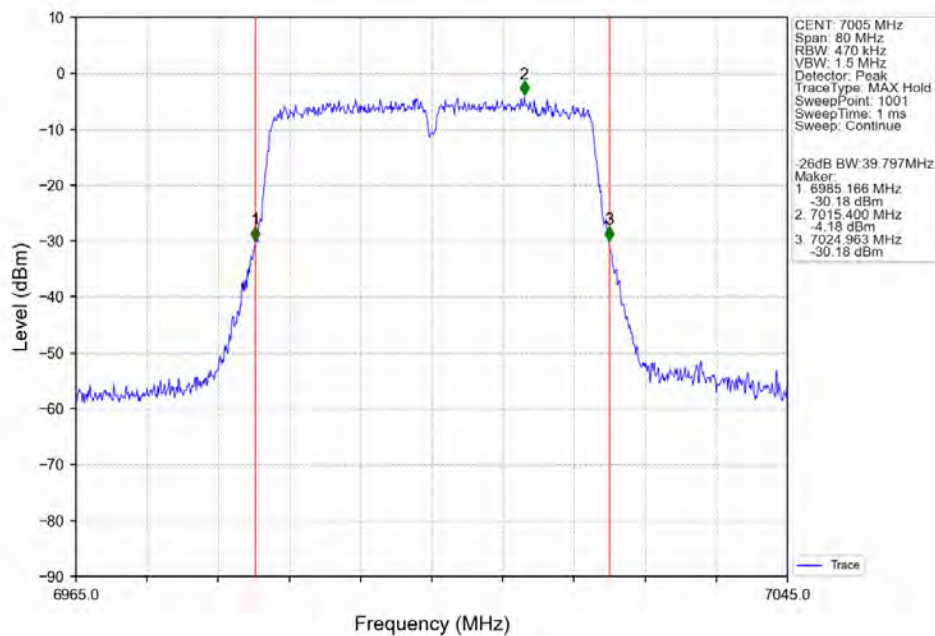
802.11n(HT40) MCH 7005MHz Ant2 NTN
