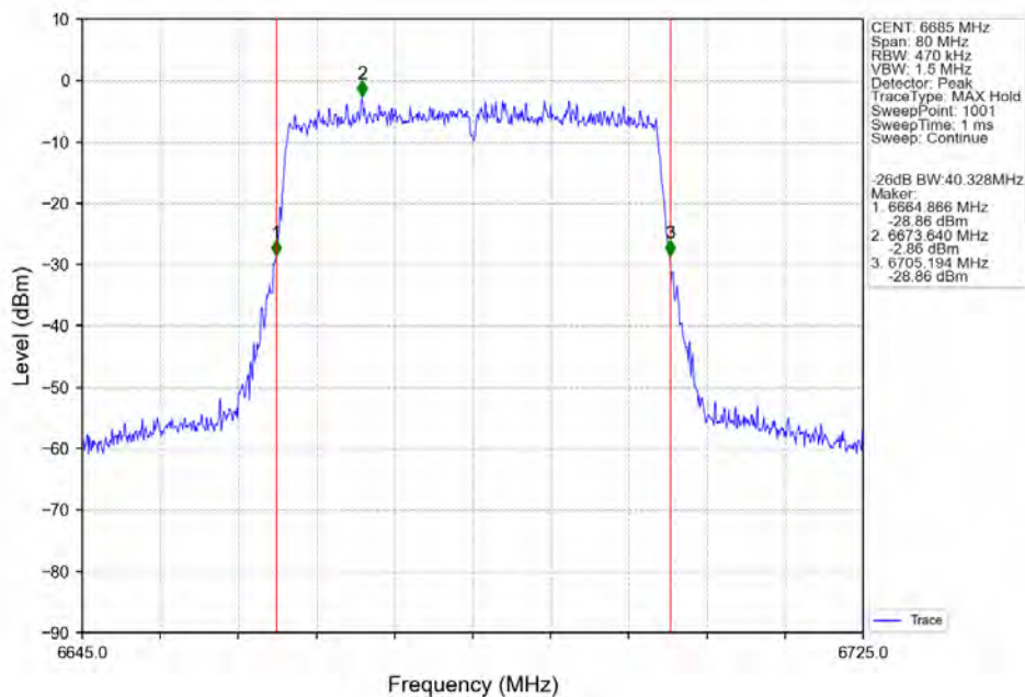
802.11ax(HEW40) MCH 6685MHz SU / Ant2 NTN
