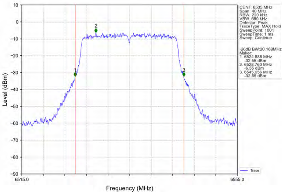
802.11ac(VHT20) LCH_6535MHz_Ant2_NTNV
