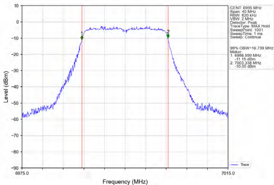
802.11a_MCH_6995MHz_Ant2_NTNV
