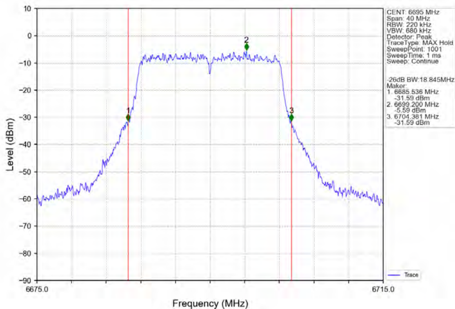
802.11a_MCH_6695MHz_Ant2_NTNV
