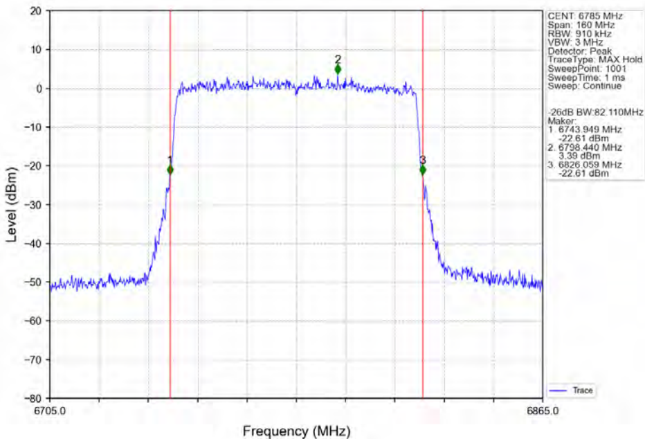
802.11ax(HEW80) HCH 6785MHz SU / Ant2 NTN
