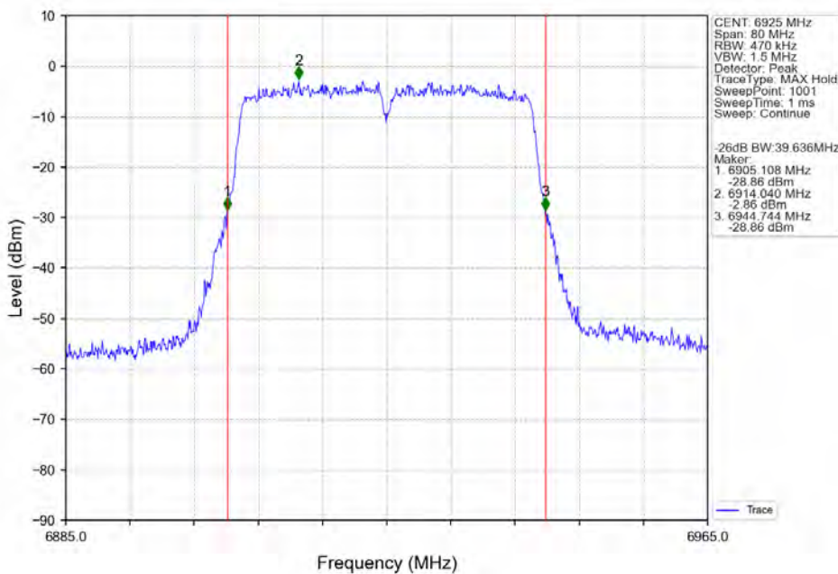
802.11n(HT40) LCH 6925MHz Ant2 NTN
