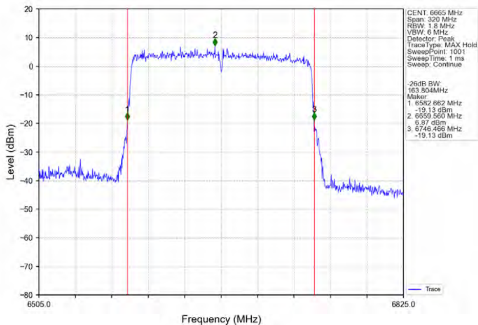
802.11ax(HEW160) MCH 6665MHz SU / Ant2_NTNV
