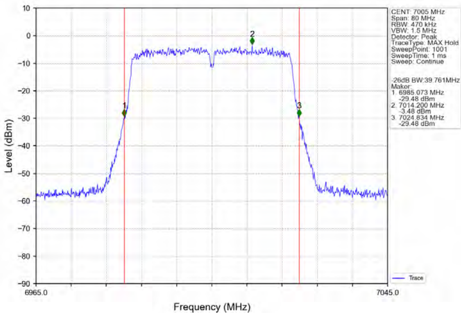
802.11ac(VHT40) MCH 7005MHz Ant2 NTVN
