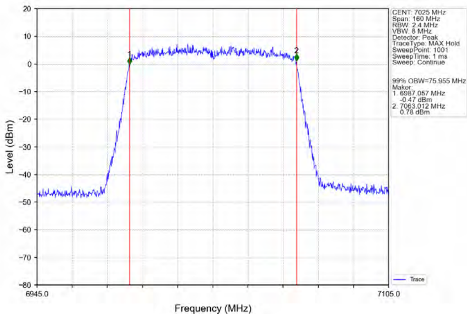
802.11ac(VHT80) HCH_7025MHz_Ant2_NTNV
