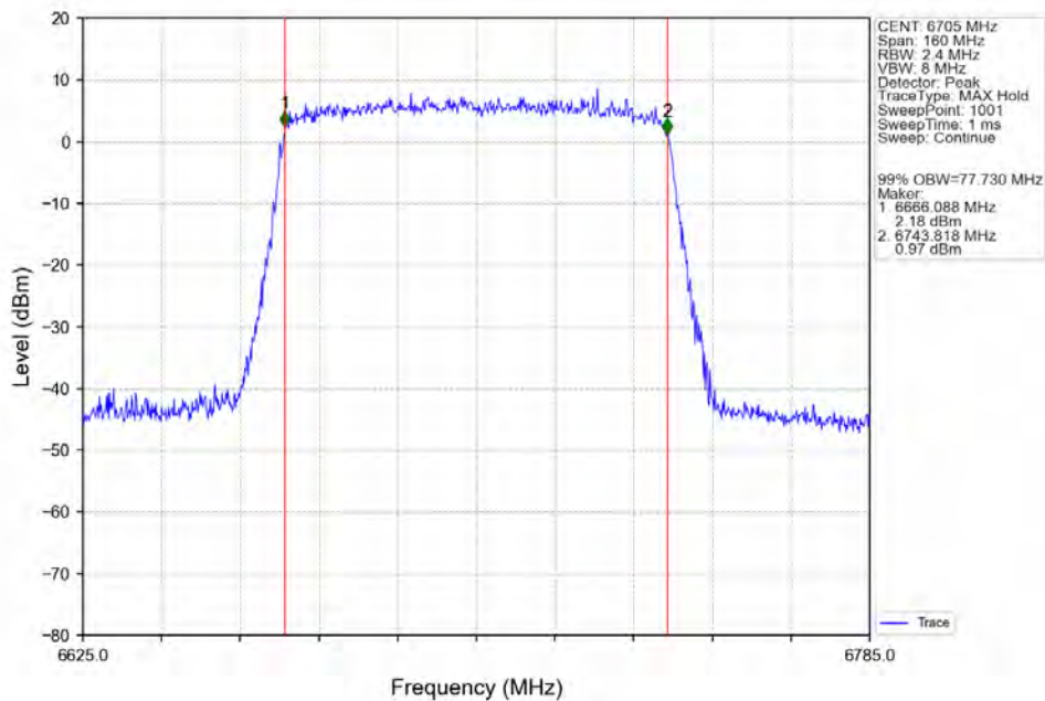
802.11ax(HEW80) MCH_6705MHz_SU / Ant2_NTNV
