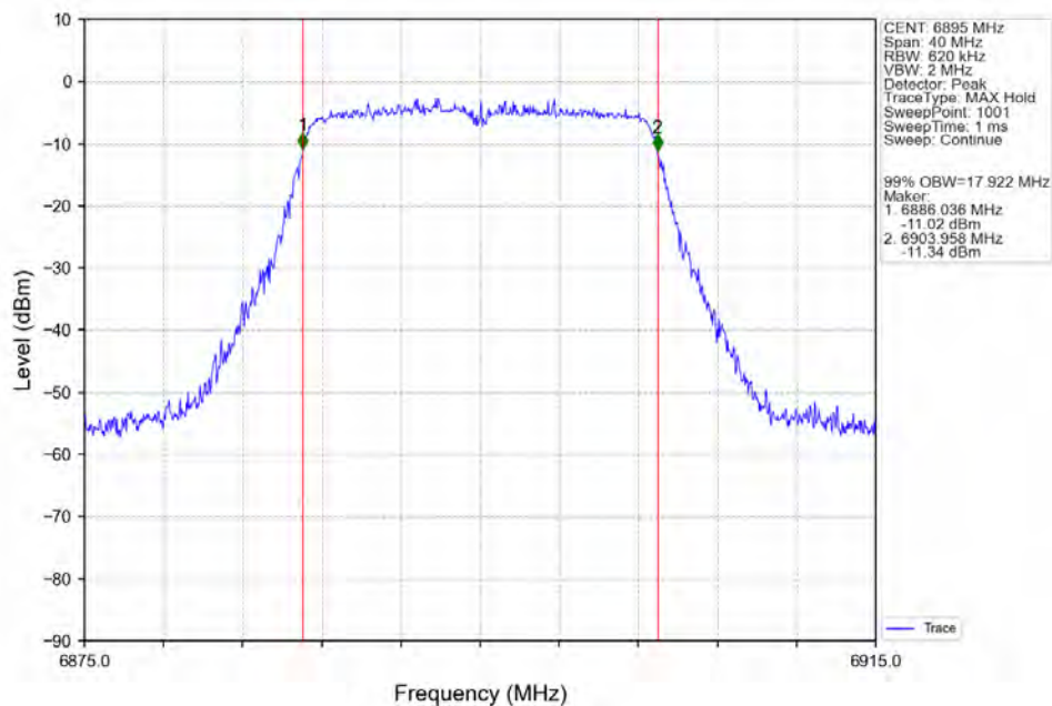
802.11n(HT20) LCH_6895MHz_Ant2_NTNV
