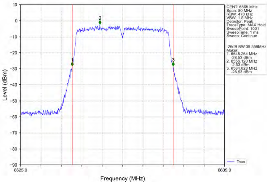
802.11n(HT40) LCH_6565MHz_Ant2_NTNV
