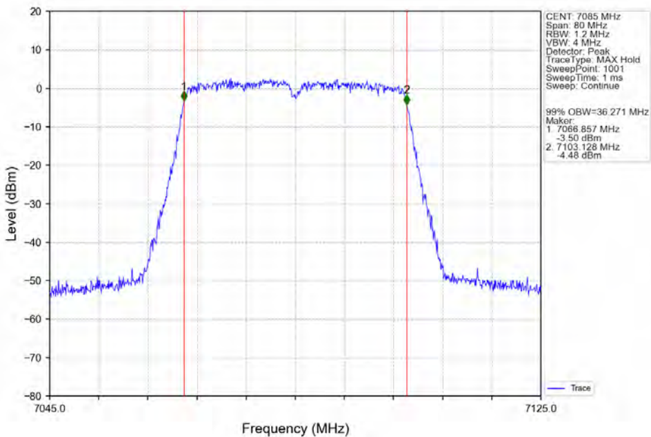
802.11ac(VHT40) HCH_7085MHz_Ant2_NTNV
