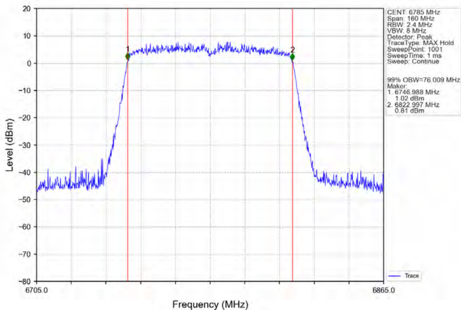
802.11ac(VHT80) HCH 6785MHz Ant2 NTN
