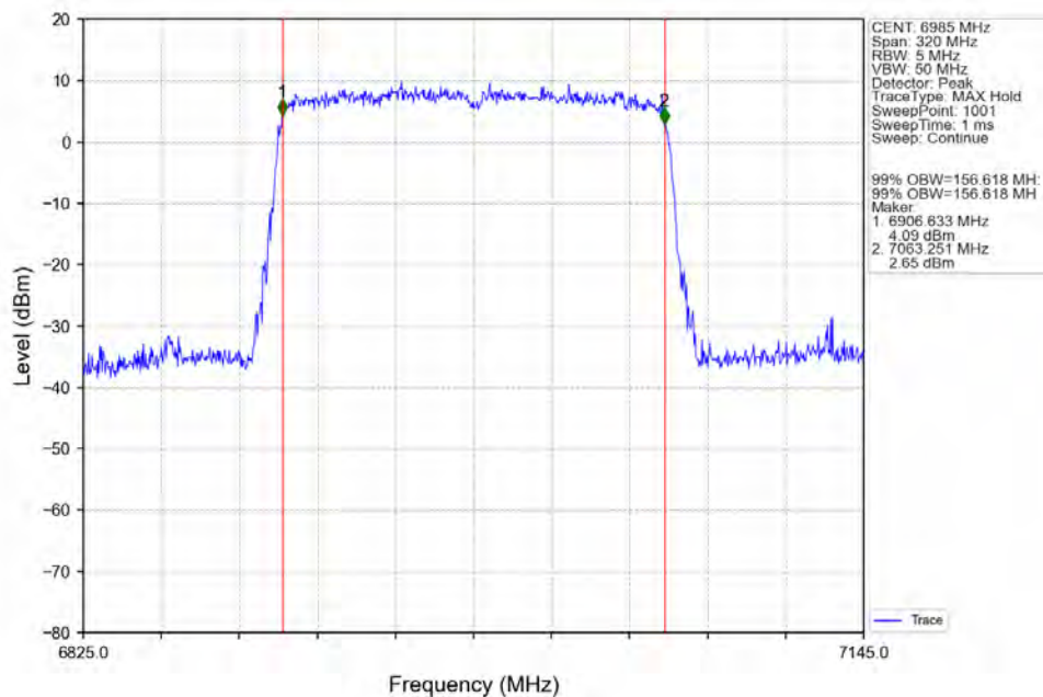
802.11ax(HEW160) MCH 6985MHz SU / Ant2 NTN
