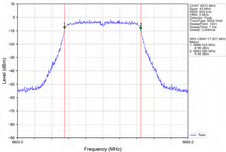
802.11n(HT20) HCH 6875MHz Ant2 NTN
