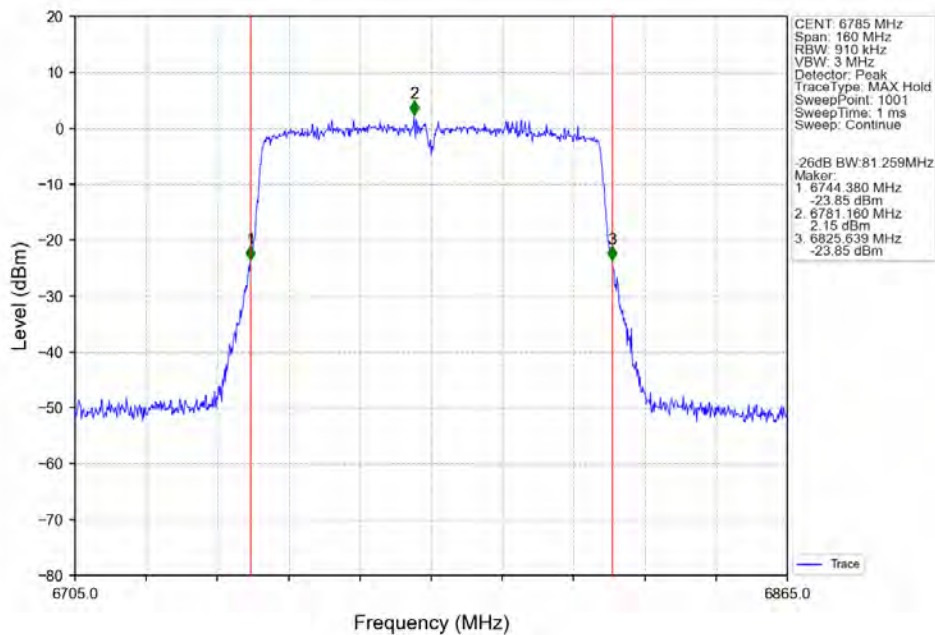
802.11ac(VHT80) HCH_6785MHz_Ant2_NTNV
