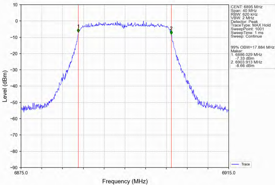
802.11ac(VHT20) LCH_6895MHz_Ant2_NTNV
