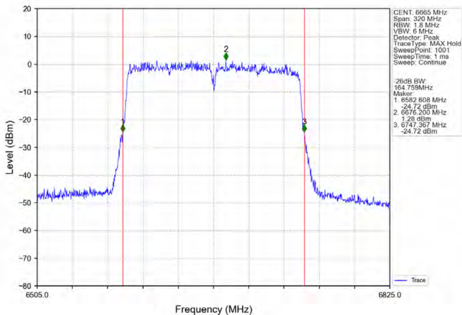
802.11ac(VHT160) MCH_6665MHz_Ant2_NTNV
