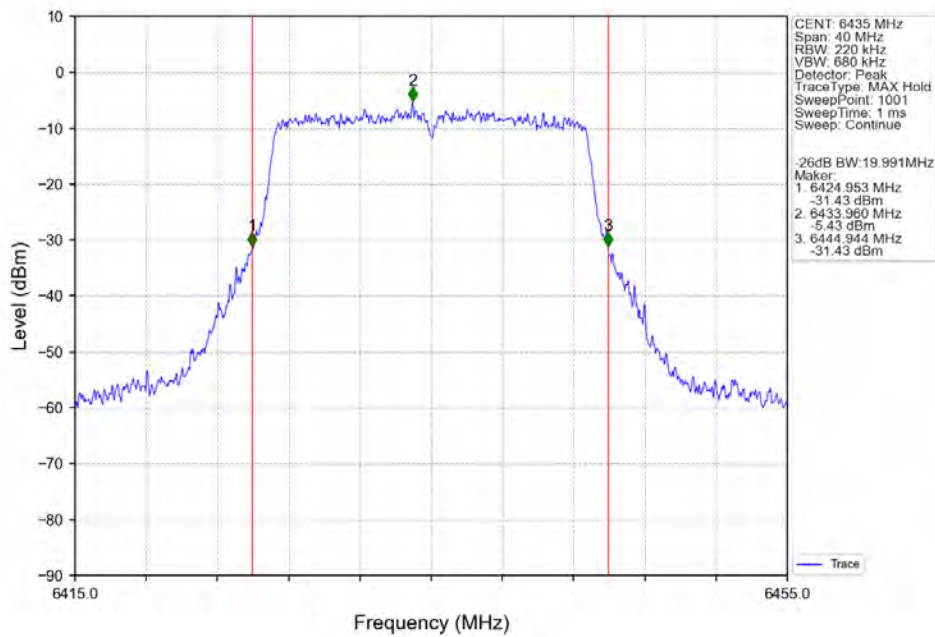
802.11ac(VHT20) LCH_6435MHz_Ant2_NTNV
