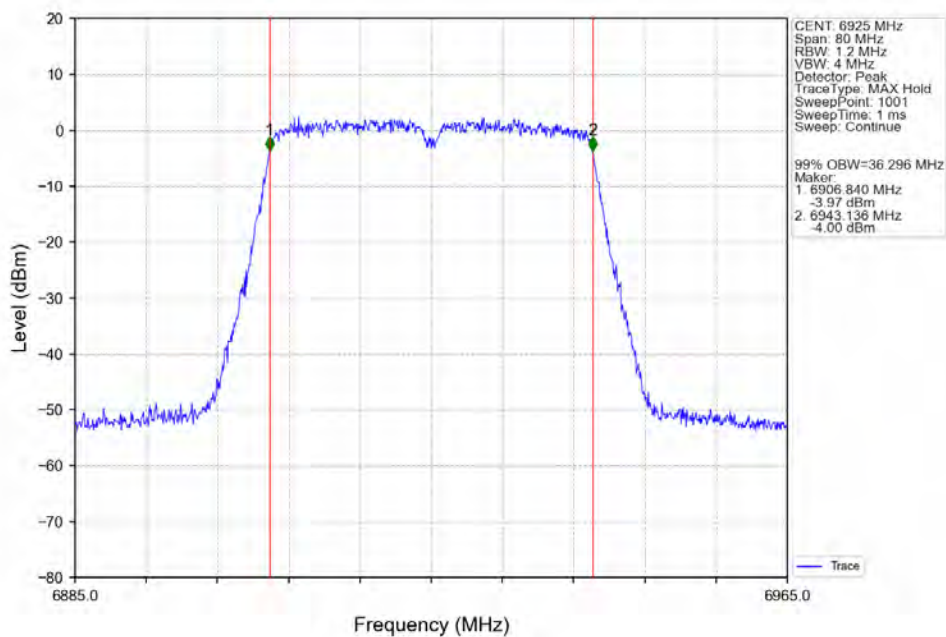
802.11ac(VHT40) LCH_6925MHz_Ant2_NTNV
