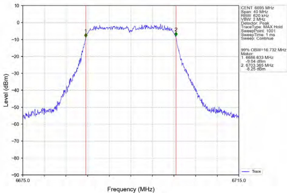
802.11a_MCH_6695MHz_Ant2_NTNV
