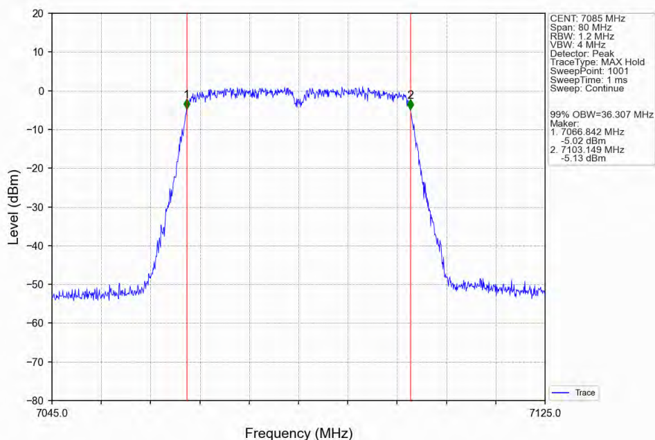
802.11n(HT40) HCH 7085MHz Ant2 NTN
