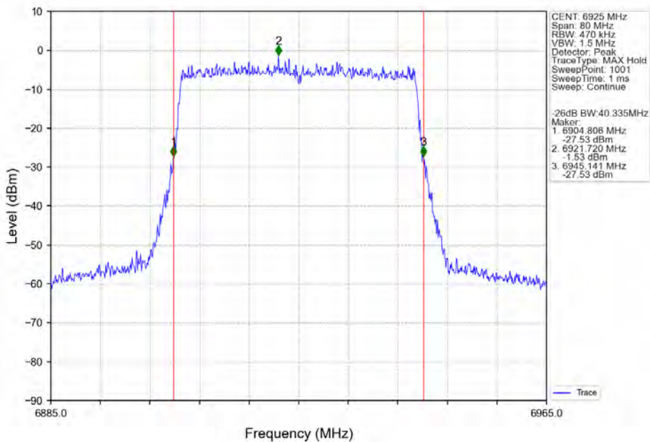
802.11ax(HEW40) LCH 6925MHz SU / Ant2 NTN
