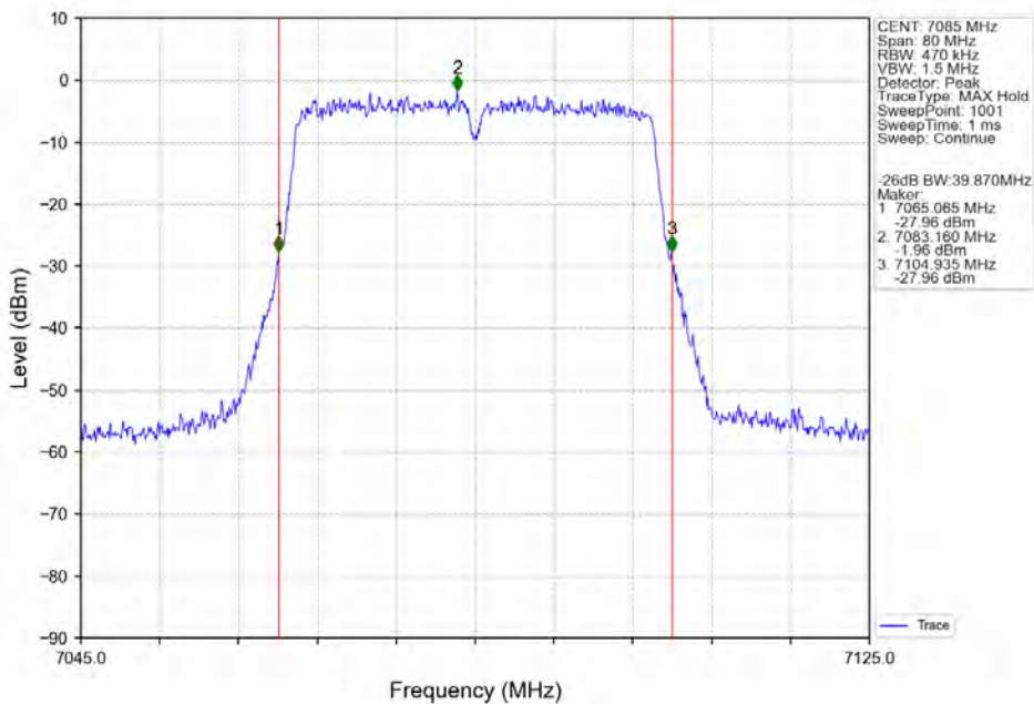
802.11ac(VHT40) HCH 7085MHz Ant2 NTN
