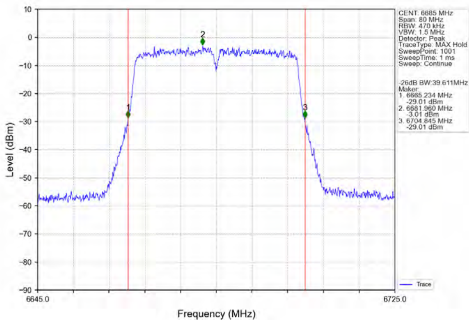
802.11n(HT40) MCH 6685MHz Ant2 NTN
