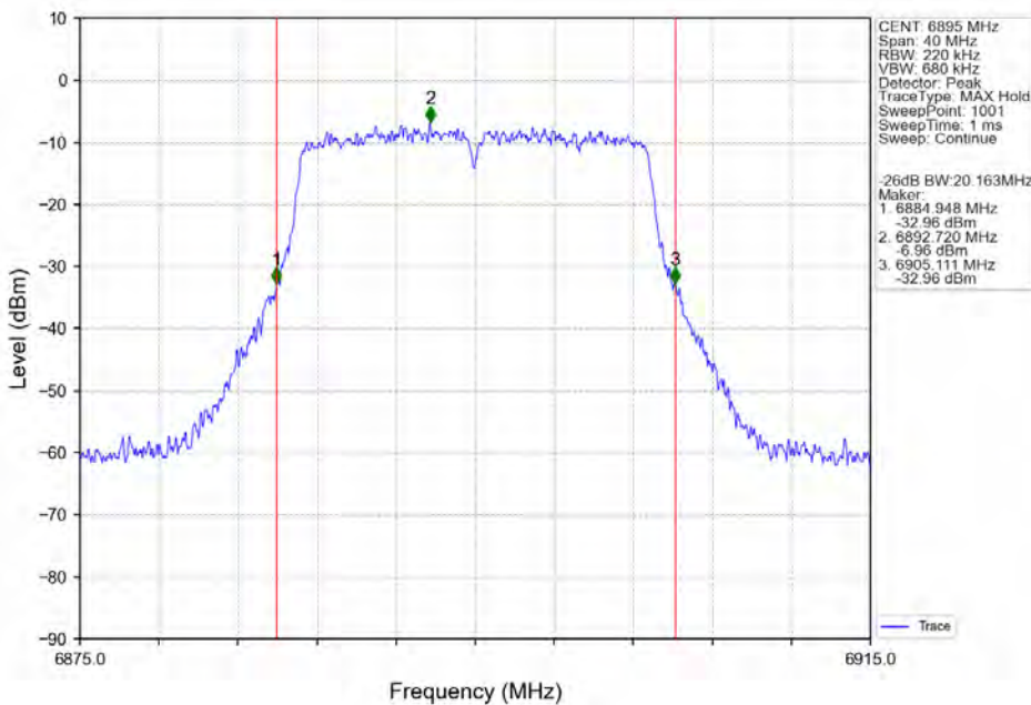
802.11n(HT20) LCH_6895MHz_Ant2_NTNV
