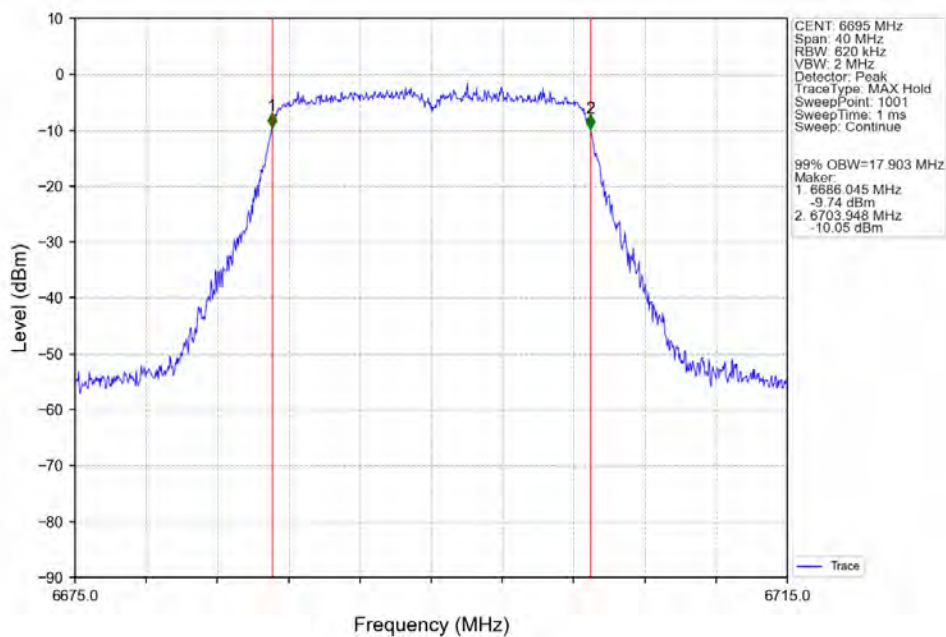
802.11n(HT20)_MCH_6695MHz_Ant2_NTNV
