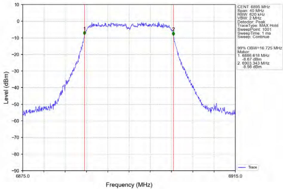
802.11a_LCH_6895MHz_Ant2_NTNV
