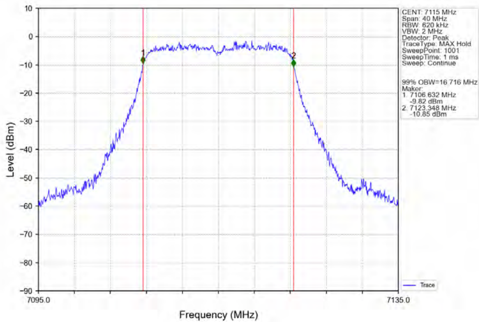
802.11a_HCH_7115MHz_Ant2_NTNV
