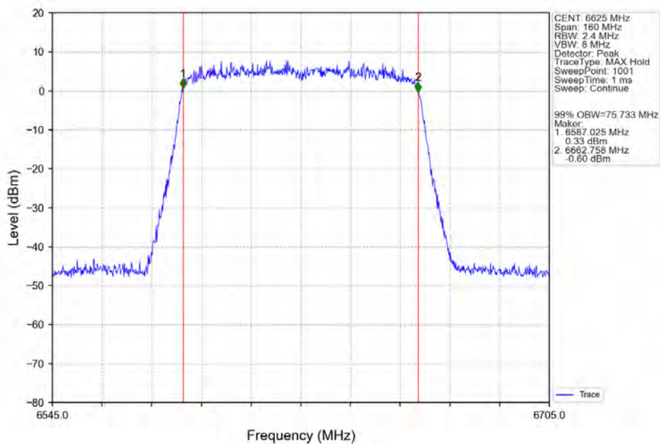
802.11ac(VHT80) LCH_6625MHz_Ant2_NTNV
