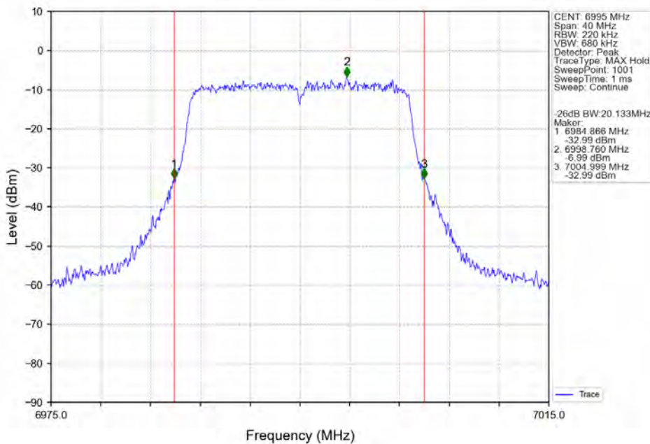
802.11ac(VHT20) MCH 6995MHz Ant2 NTN
