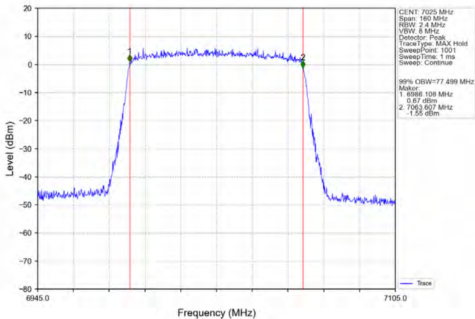
802.11ax(HEW80) HCH 7025MHz SU / Ant2 NTN
