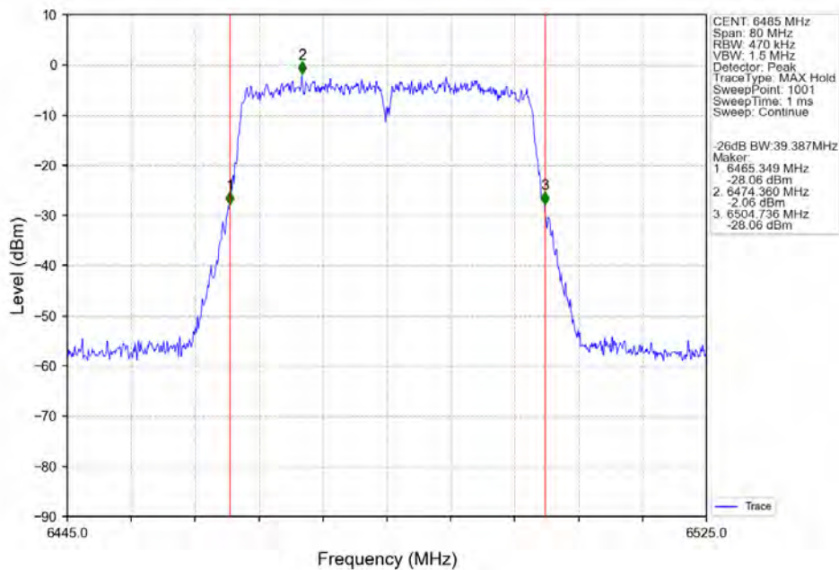
802.11n(HT40) MCH 6485MHz Ant2 NTN
