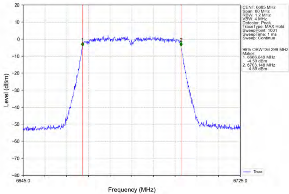
802.11n(HT40) MCH 6685MHz Ant2_NTNV
