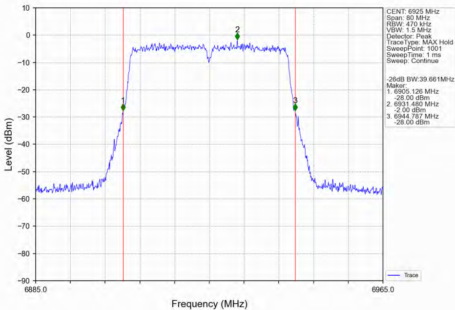
802.11ac(VHT40) LCH 6925MHz Ant2 NTN
