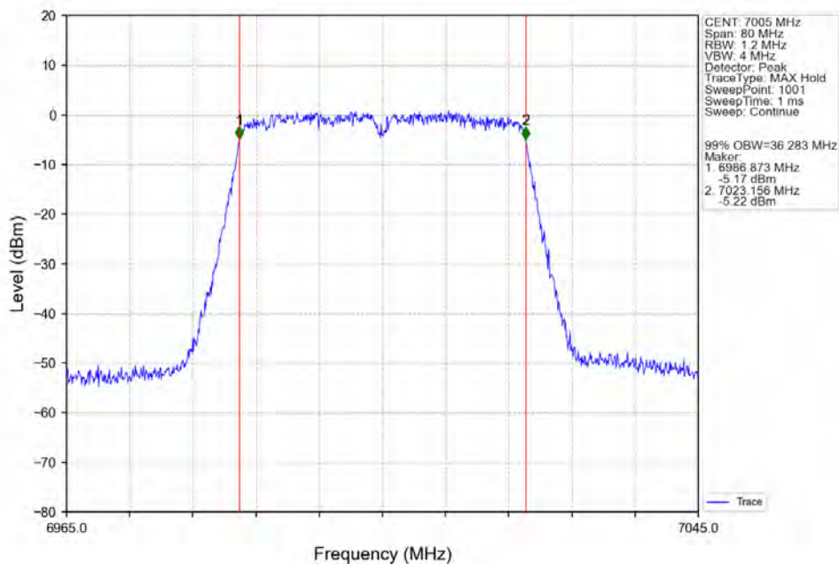
802.11n(HT40) MCH_7005MHz_Ant2_NTNV
