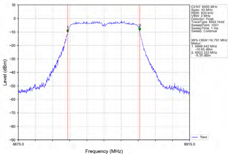
802.11a_LCH_6895MHz_Ant2_NTNV
