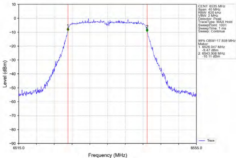
802.11ac(VHT20) LCH_6535MHz_Ant2_NTNV
