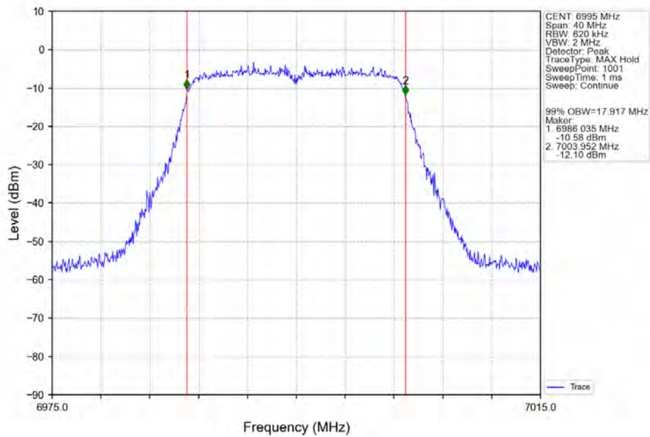
802.11n(HT20) MCH 6995MHz Ant2 NTN
