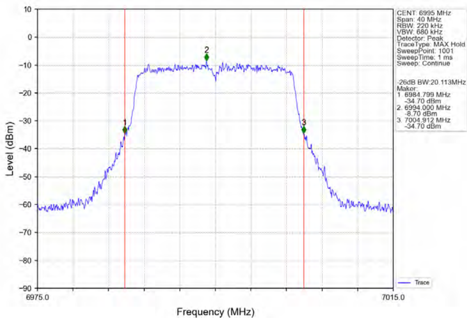
802.11n(HT20) MCH 6995MHz Ant2_NTNV
