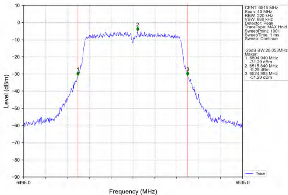
802.11ac(VHT20) HCH 6515MHz Ant2 NTN
