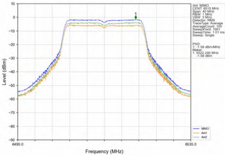
802.11n(HT20)_HCH_6515MHz_MIMO_NTNV
