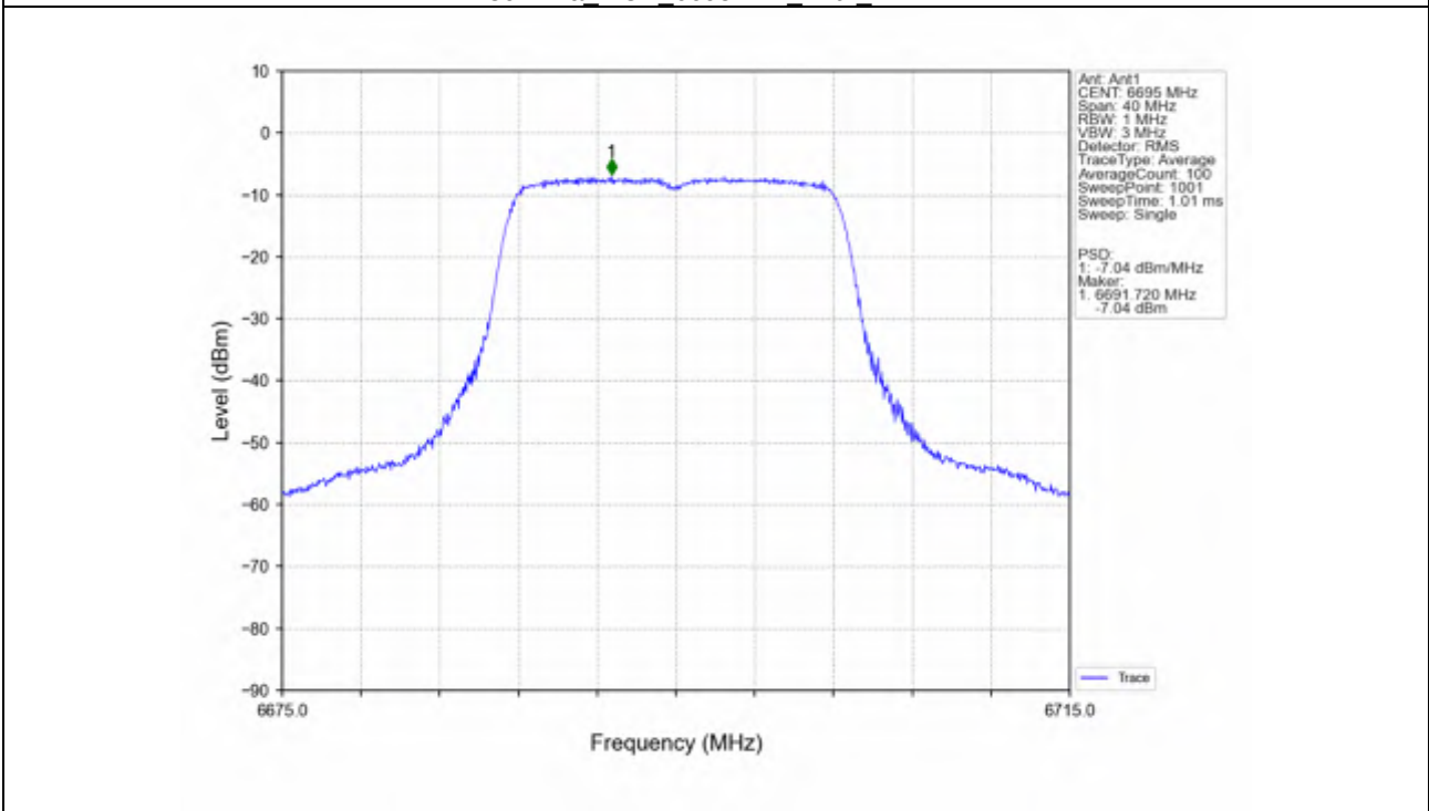
802.11a_MCH_6695MHz_Ant1_NTNV
