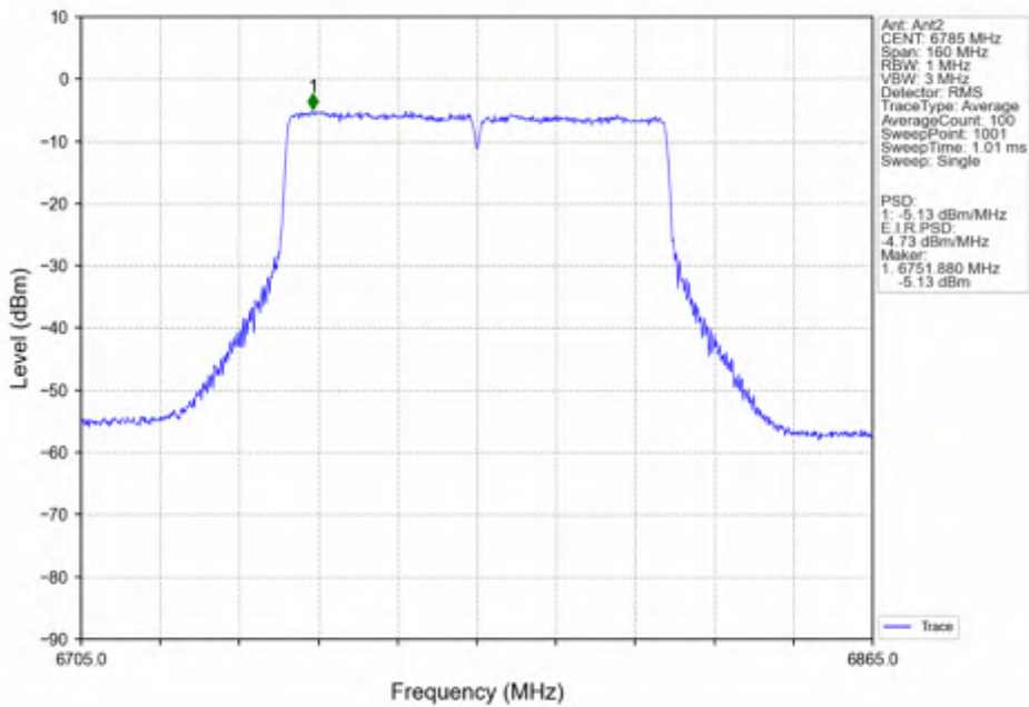
802.11ac(VHT80)_HCH_6785MHz_MIMO_NTNV
