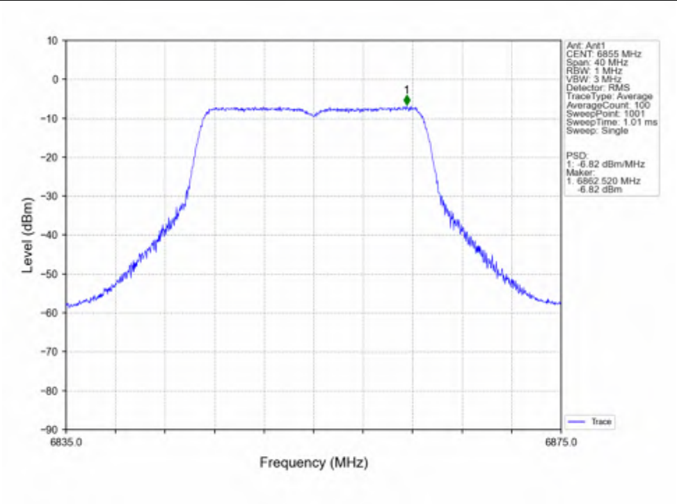
802.11n(HT20) HCH 6855MHz Ant1 NTN
