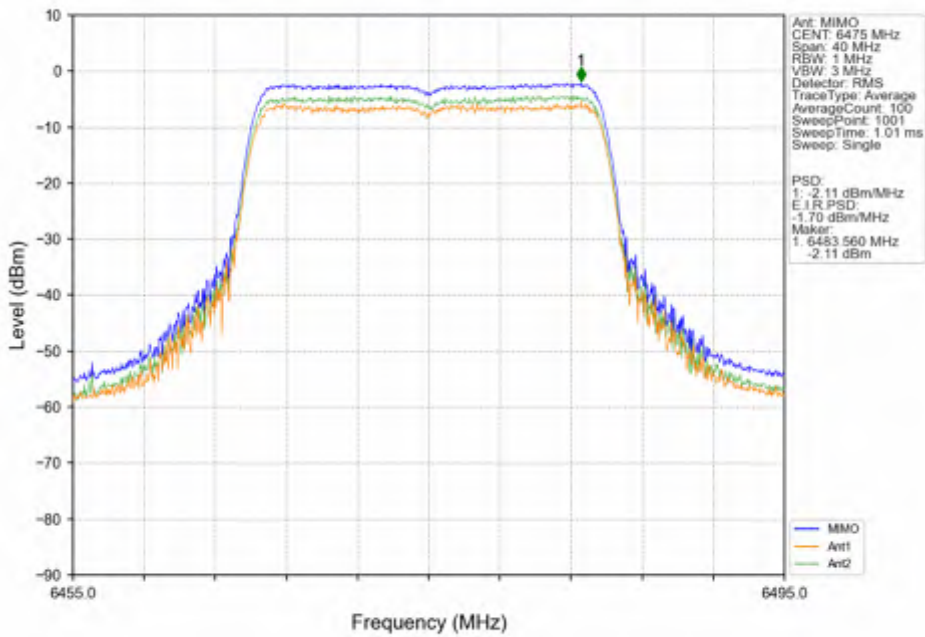
802.11ax(HEW20) MCH 6475MHz SU / MIMO NTN
