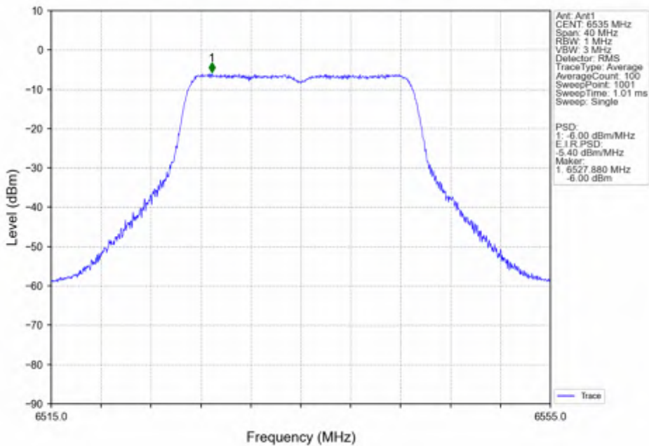
802.11n(HT20)_LCH_6535MHz_Ant1_NTNV
