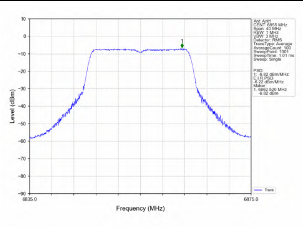
802.11n(HT20) HCH 6855MHz Ant1_NTNV
