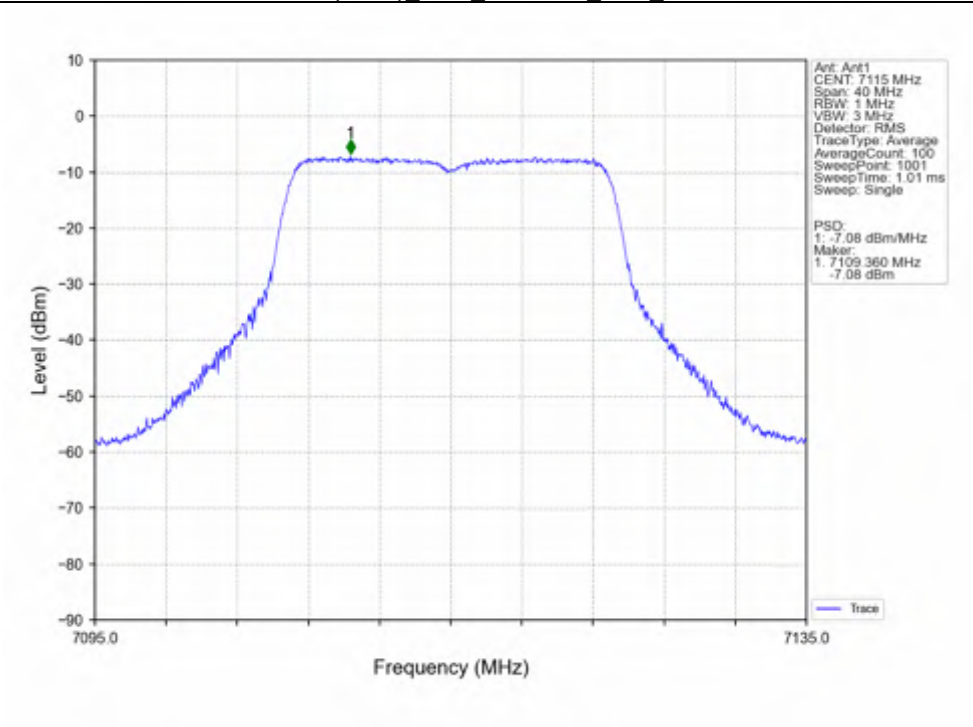
802.11n(HT20) HCH 7115MHz Ant1_NTNV
