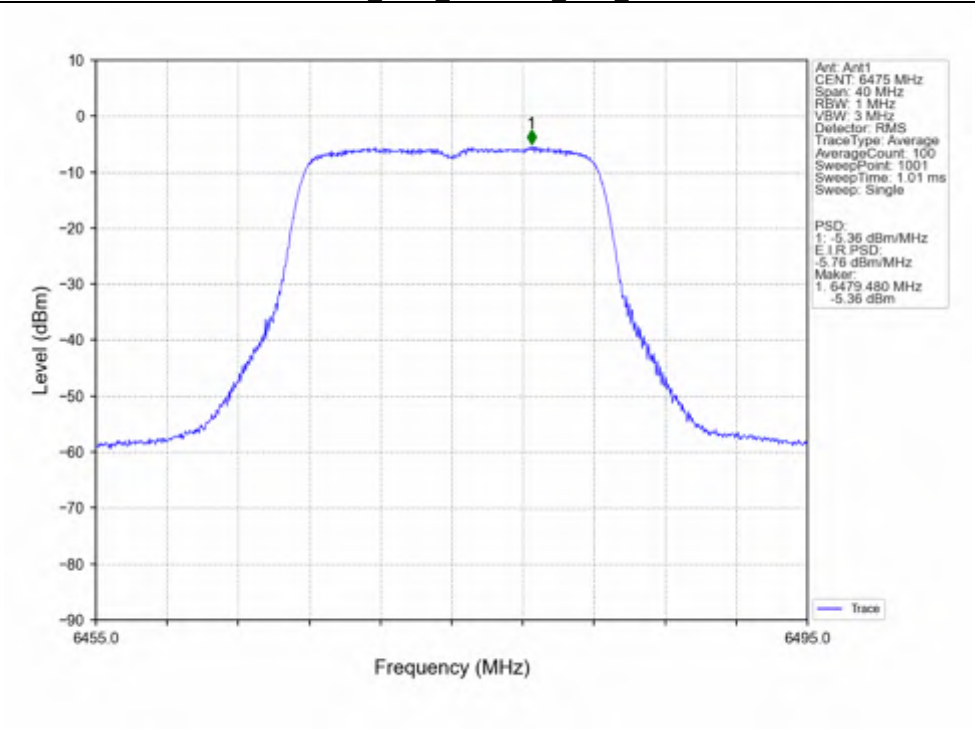
802.11a_MCH_6475MHz_Ant1_NTNV
