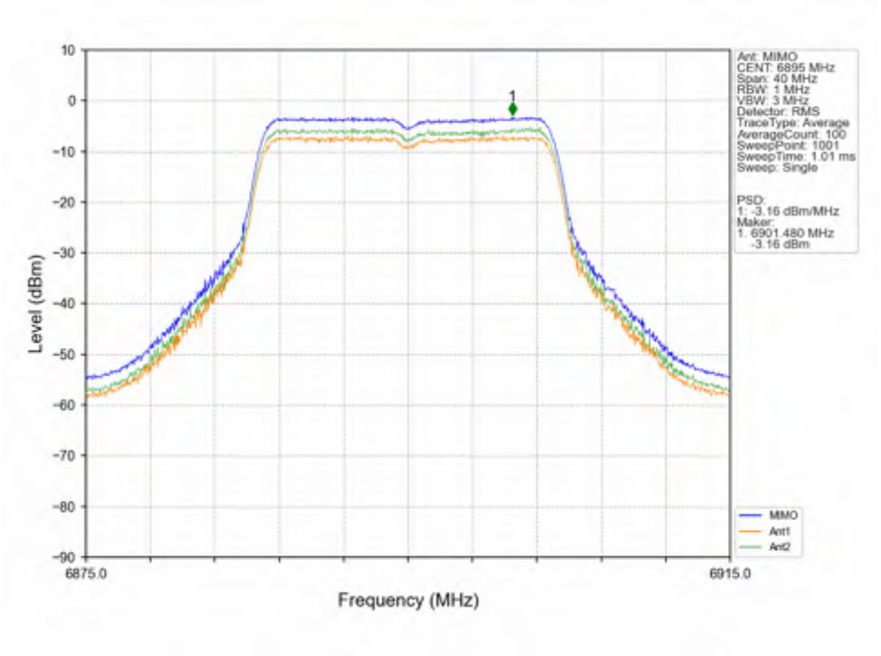
802.11n(HT20)_LCH_6895MHz_MIMO_NTNV
