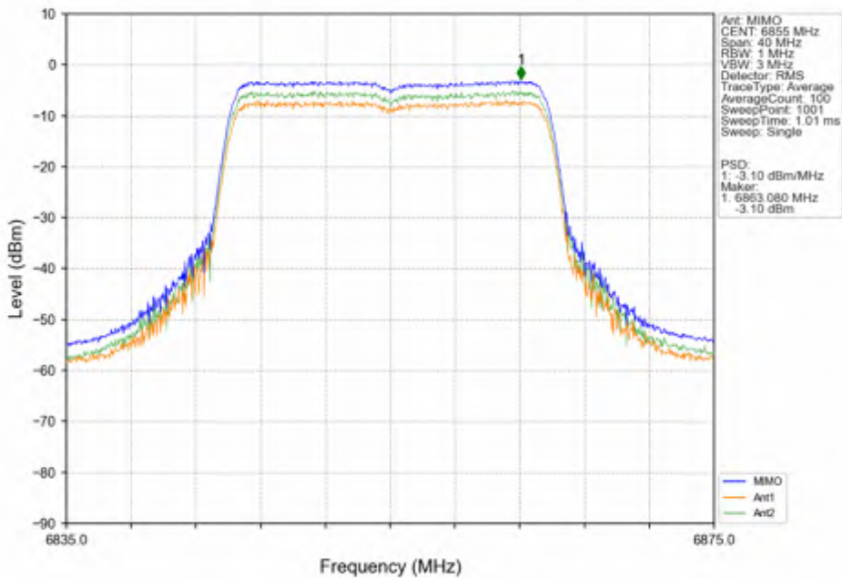
802.11ax(HEW20) HCH 6855MHz SU / MIMO_NTNV
