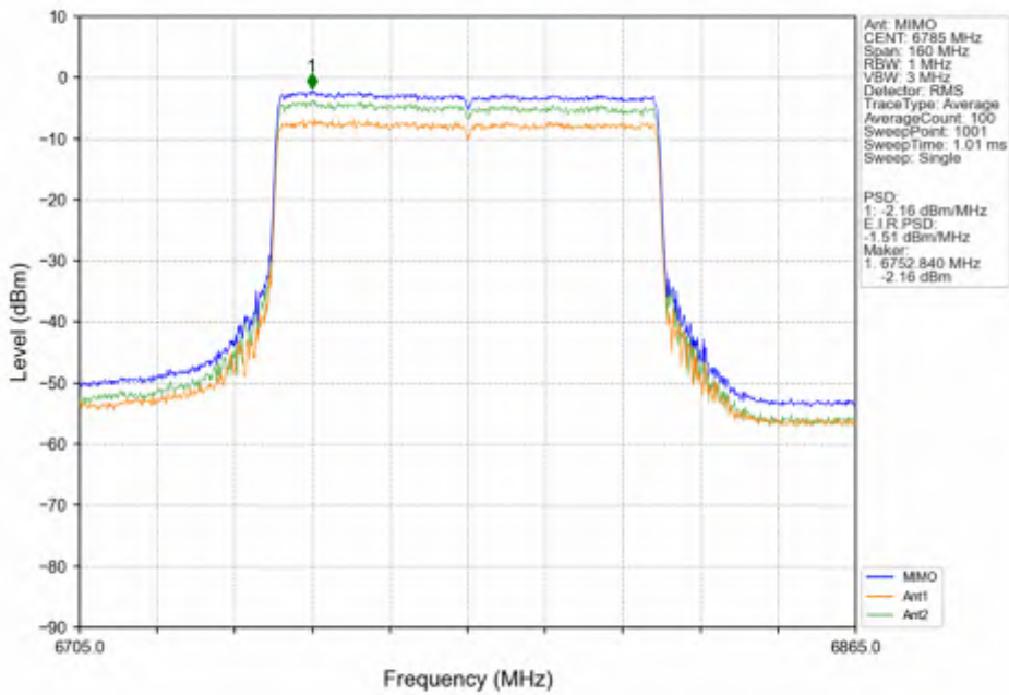
802.11ax(HEW80) HCH 6785MHz SU / MIMO_NTNV
