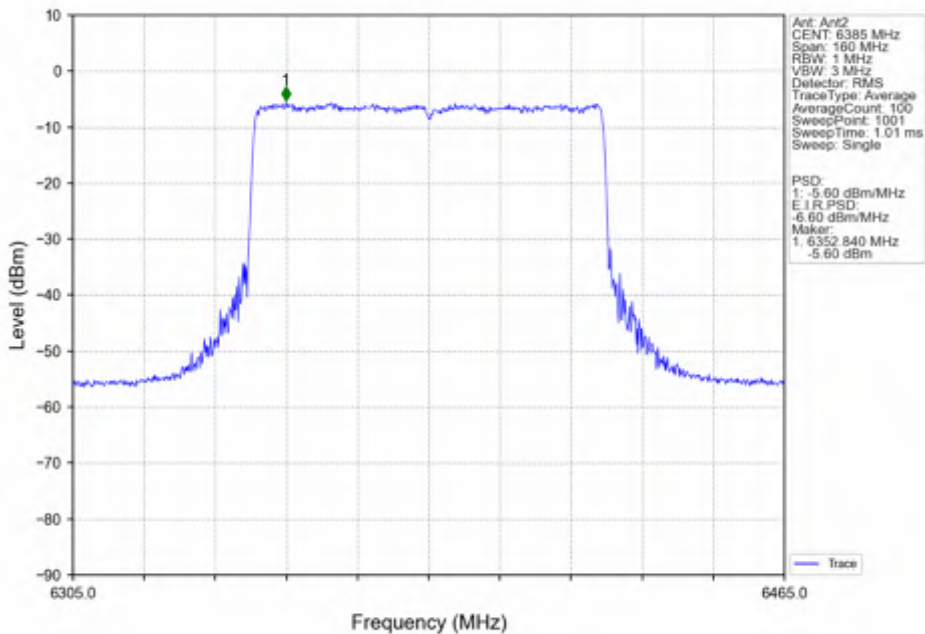
802.11ax(HEW80) HCH 6385MHz SU / MIMO NTN
