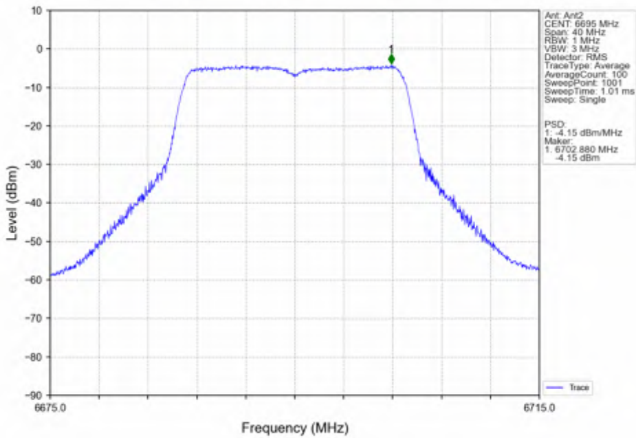
802.11n(HT20)_MCH_6695MHz_Ant2_NTNV
