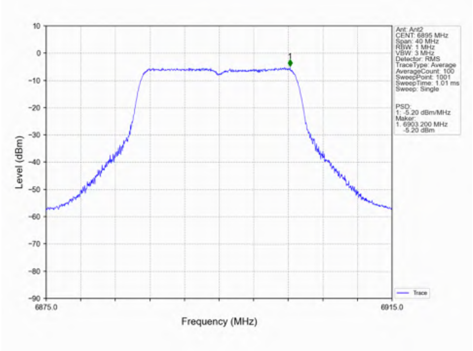
802.11n(HT20)_LCH_6895MHz_MIMO_NTNV
