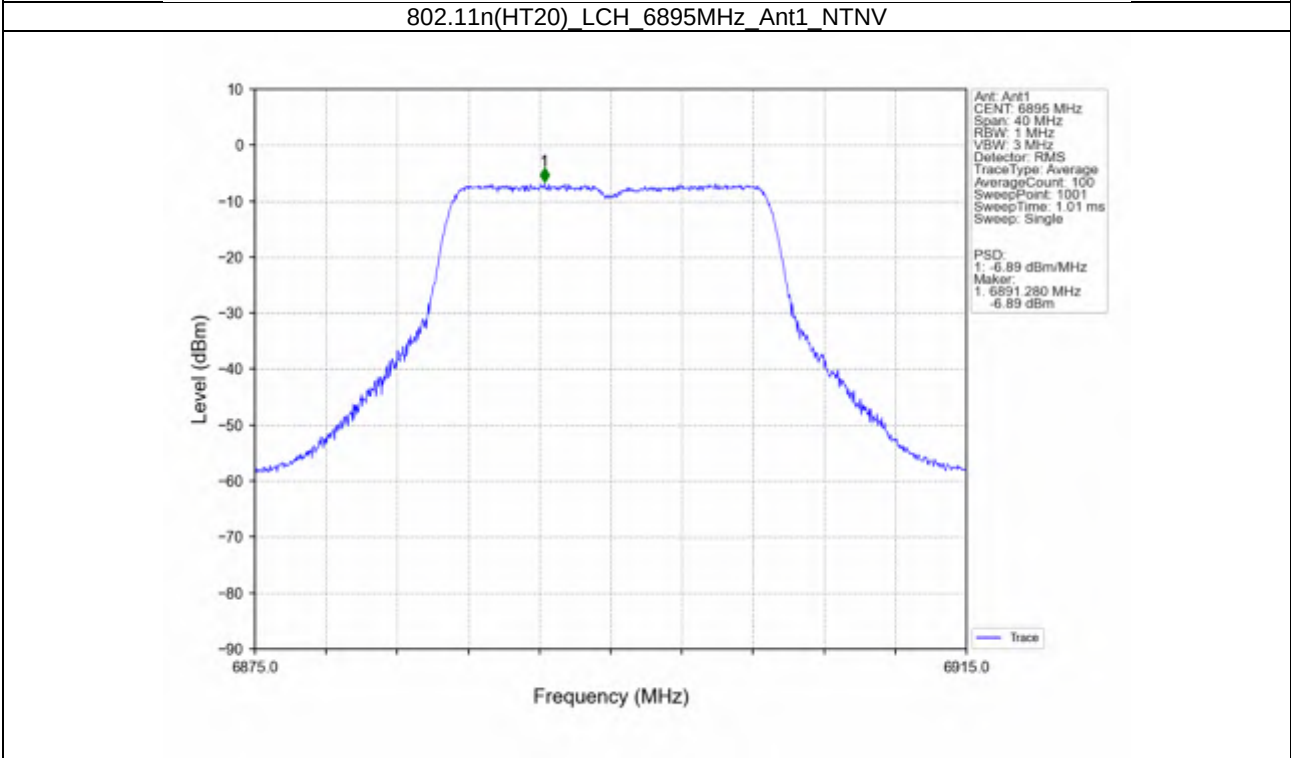
802.11n(HT20)_LCH_6895MHz_Ant1_NTNV
