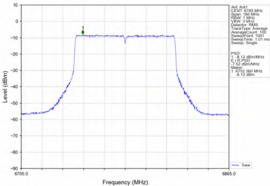
802.11ac(VHT80)_HCH_6785MHz_Ant1_NTNV
