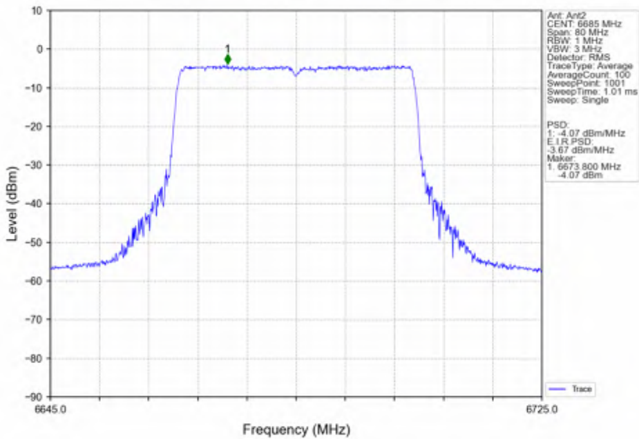
802.11ax(HEW40) MCH 6685MHz SU / MIMO NTN
