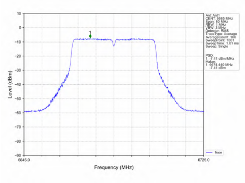
802.11n(HT40)_MCH_6685MHz_Ant1_NTNV
