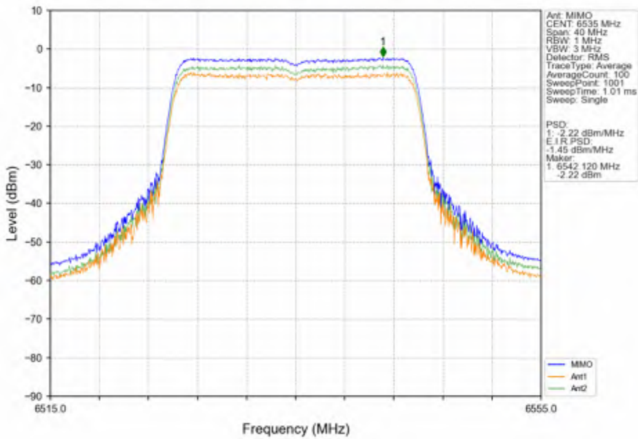
802.11ax(HEW20) LCH 6535MHz SU / MIMO NTN
