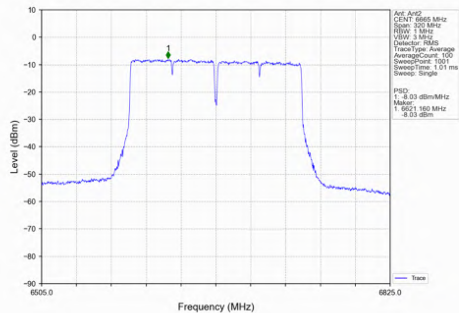
802.11ac(VHT160) MCH_6665MHz_Ant2_NTNV
