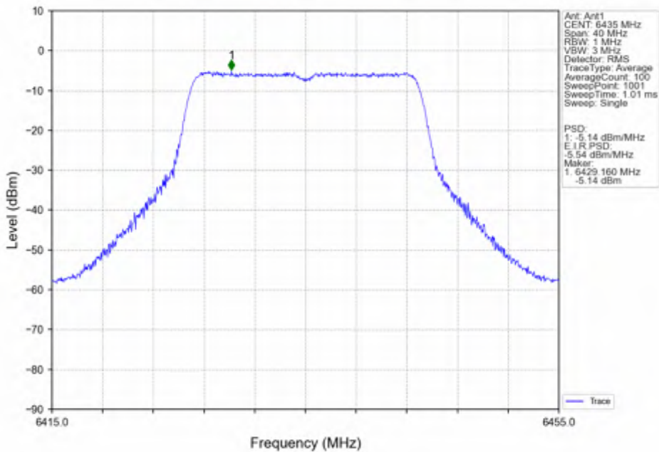
802.11n(HT20)_LCH_6435MHz_Ant1_NTNV
