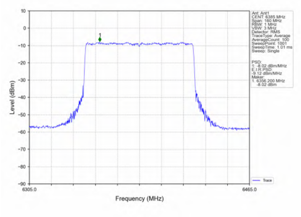
802.11ax(HEW80)_HCH_6385MHz_SU / Ant1_NTNV
