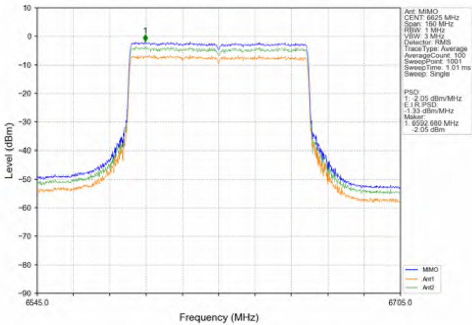
802.11ax(HEW80) LCH 6625MHz SU / MIMO_NTNV
