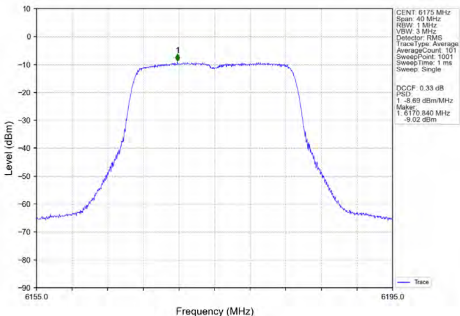
802.11n(HT20) MCH 6175MHz Ant2 NTN
