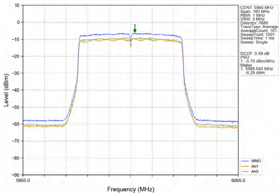
802.11ac(VHT80) LCH 5985MHz MIMO NTN
