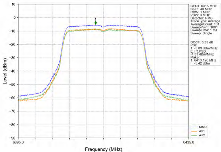
802.11ac(VHT20) HCH 6415MHz MIMO NTN
