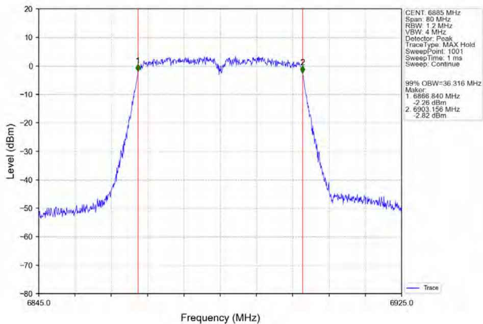
802.11ac(VHT40) HCH 6885MHz Ant2 NTN
