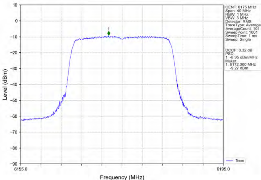
802.11ax(HEW20) MCH 6175MHz SU / Ant2 NTN
