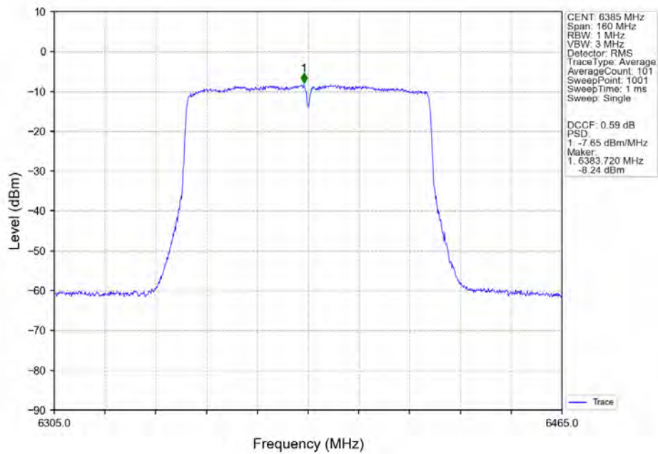
802.11ac(VHT80) HCH 6385MHz MIMO NTN
