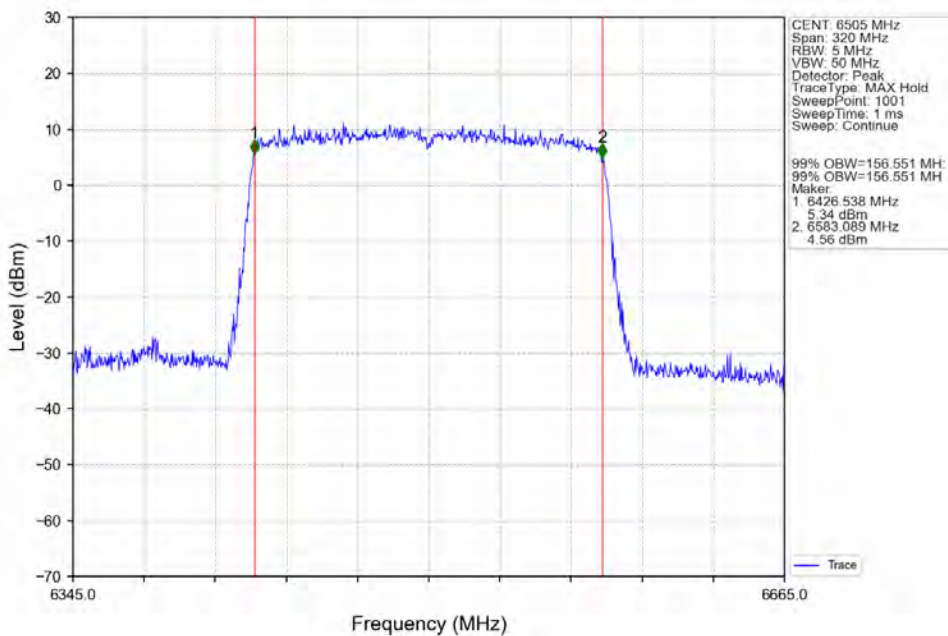
802.11ax(HEW160) HCH 6505MHz SU / Ant2 NTN
