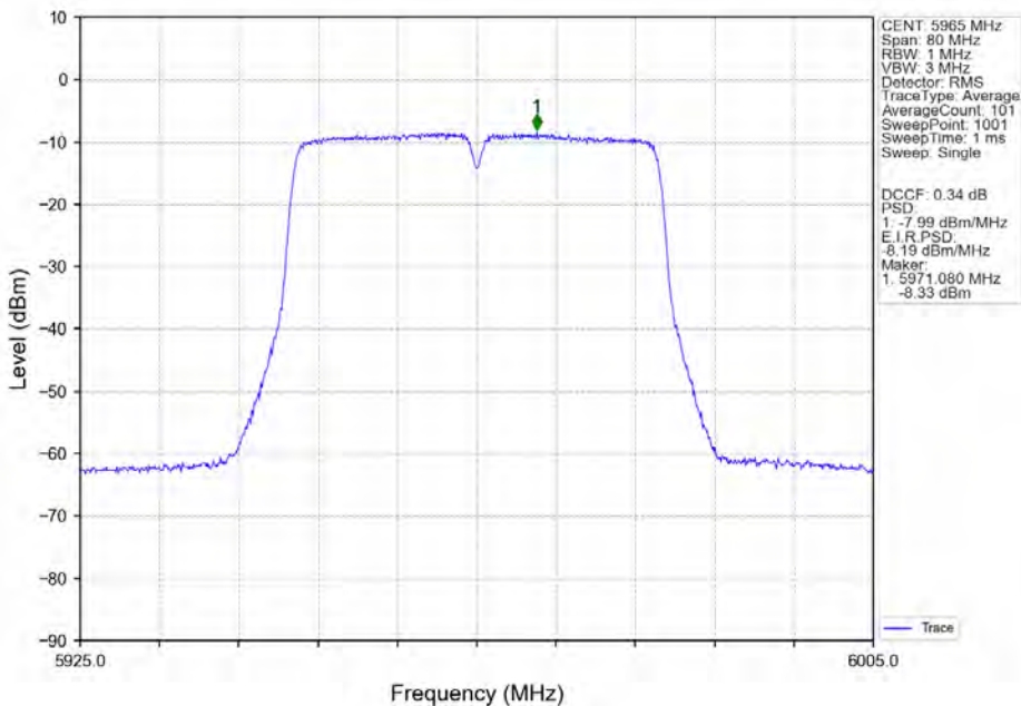
802.11ac(VHT40) LCH_5965MHz_Ant2_NTNV
