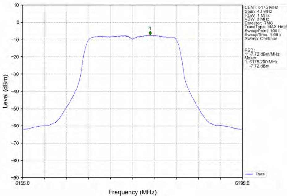
802.11a MCH 6175MHz MIMO NTN
