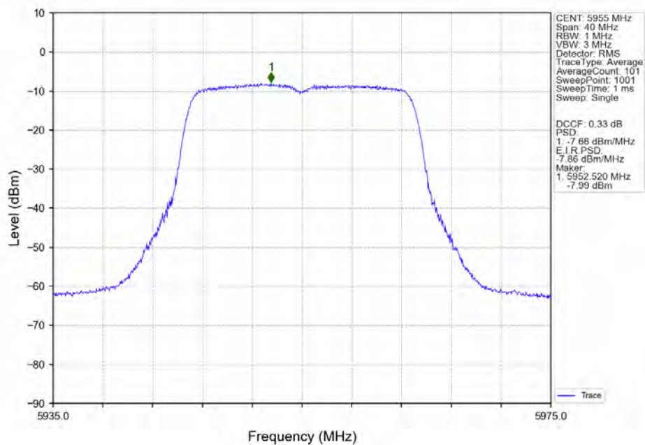
802.11n(HT20) LCH 5955MHz MIMO NTN
