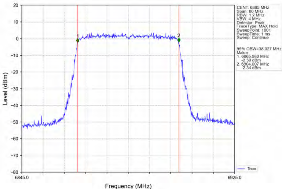
802.11ax(HEW40) HCH 6885MHz SU / Ant2 NTN
