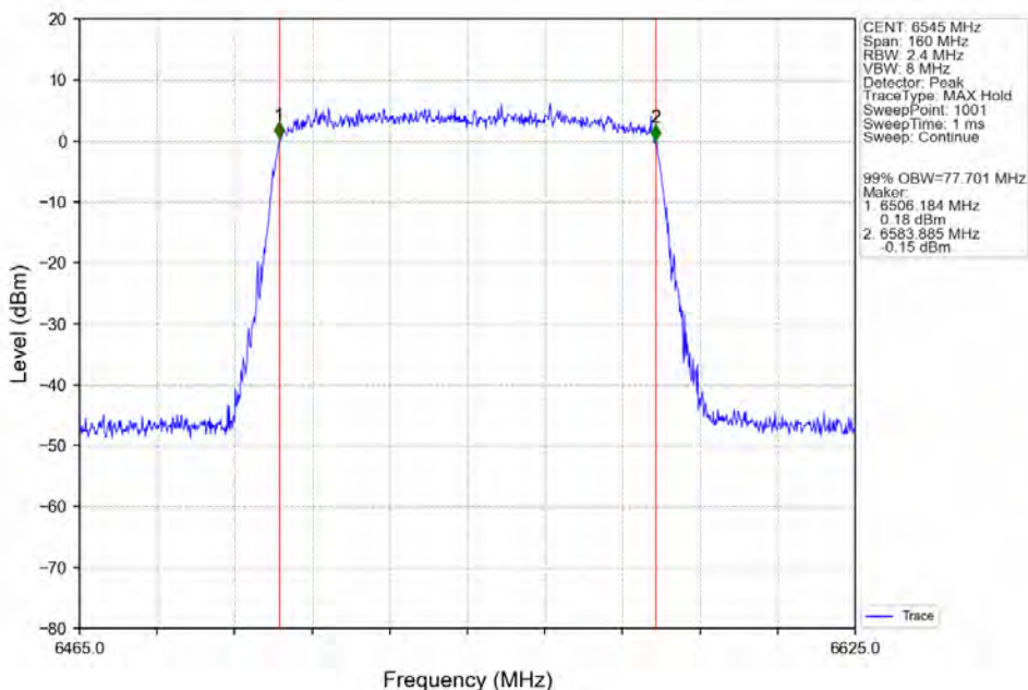
802.11ax(HEW80) HCH 6545MHz SU / Ant2 NTN
