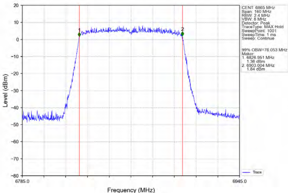
802.11ac(VHT80) HCH 6865MHz Ant2 NTN
