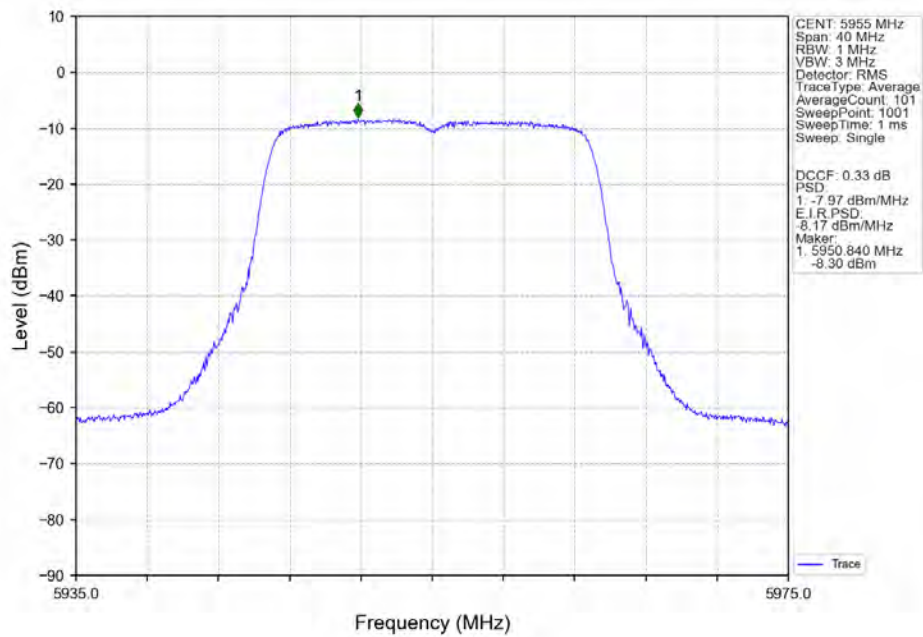
802.11ac(VHT20) LCH 5955MHz MIMO NTN
