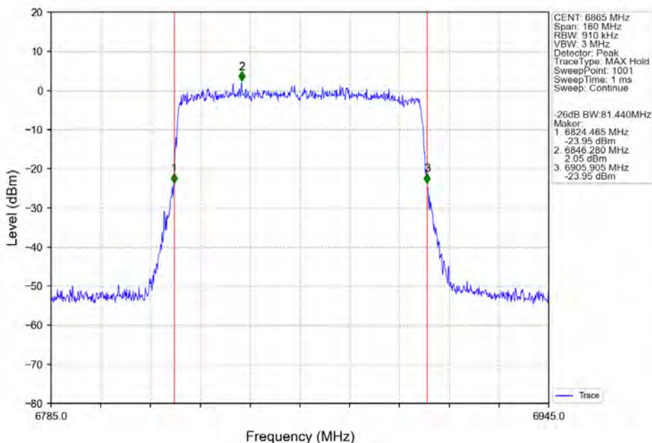
802.11ax(HEW80) HCH 6865MHz SU / Ant2 NTN
