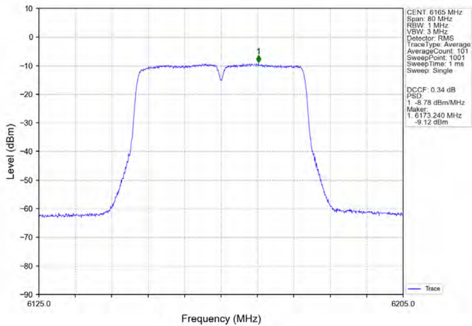
802.11ac(VHT40) MCH 6165MHz MIMO NTN
