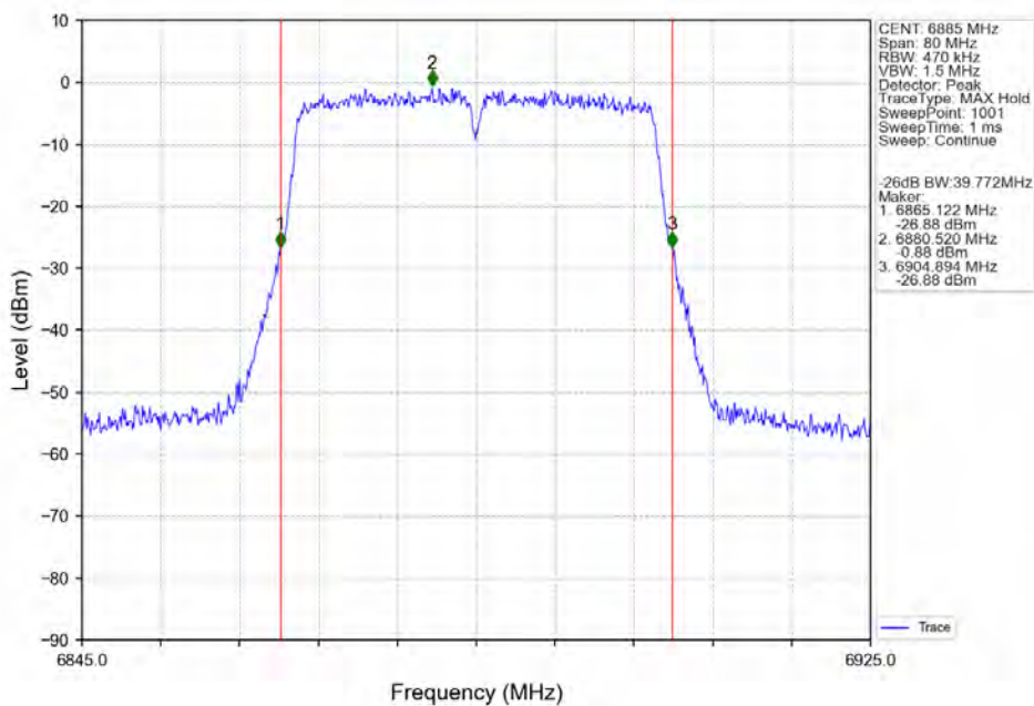
802.11ac(VHT40) HCH 6885MHz Ant2 NTN
