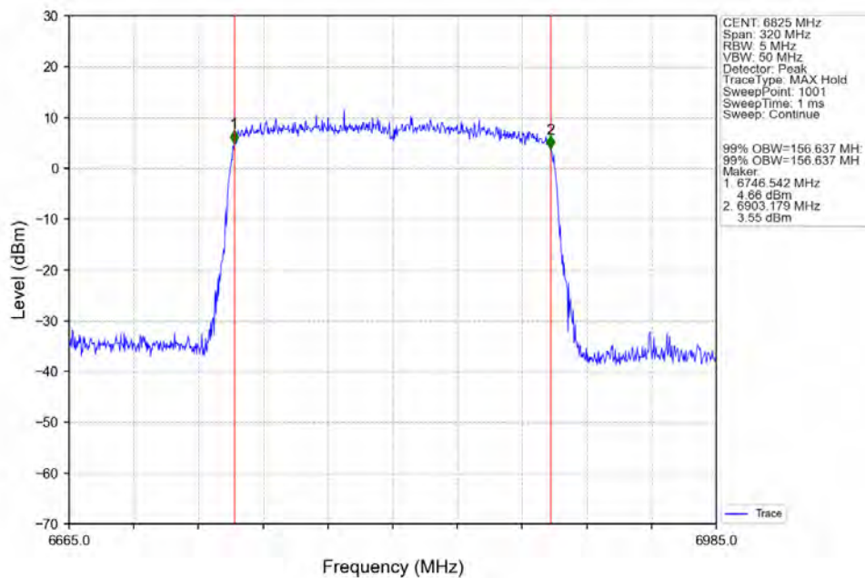
802.11ax(HEW160) HCH 6825MHz SU / Ant2 NTN
