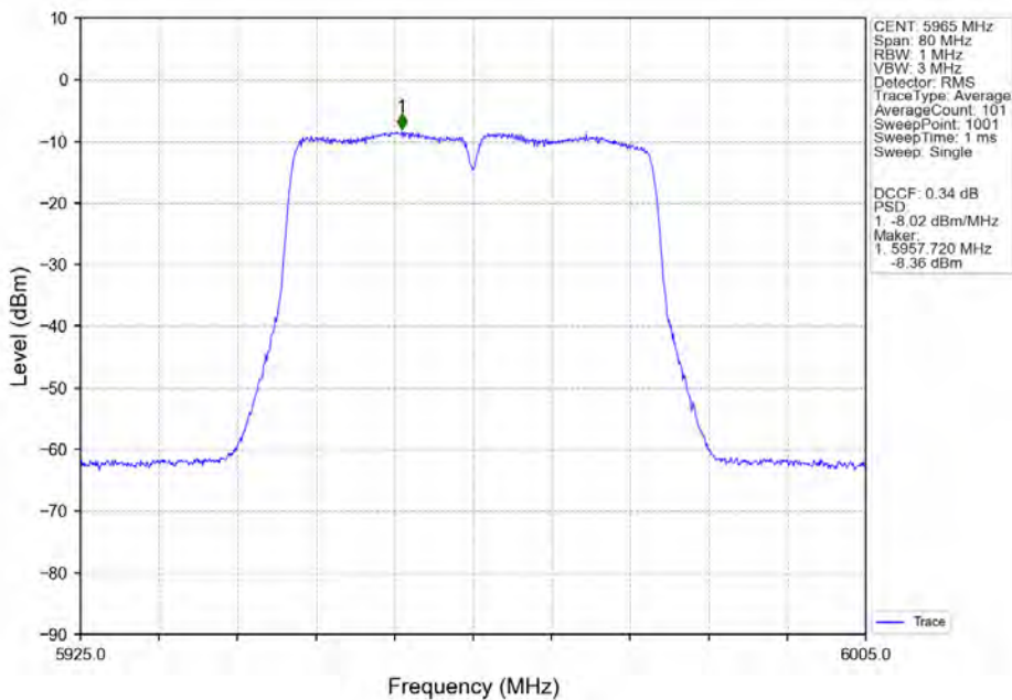
802.11ac(VHT40) LCH 5965MHz Ant2 NTN
