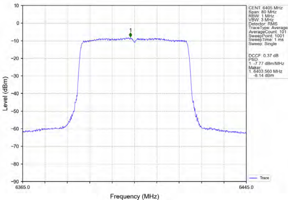
802.11ax(HEW40) HCH 6405MHz SU / Ant2 NTN
