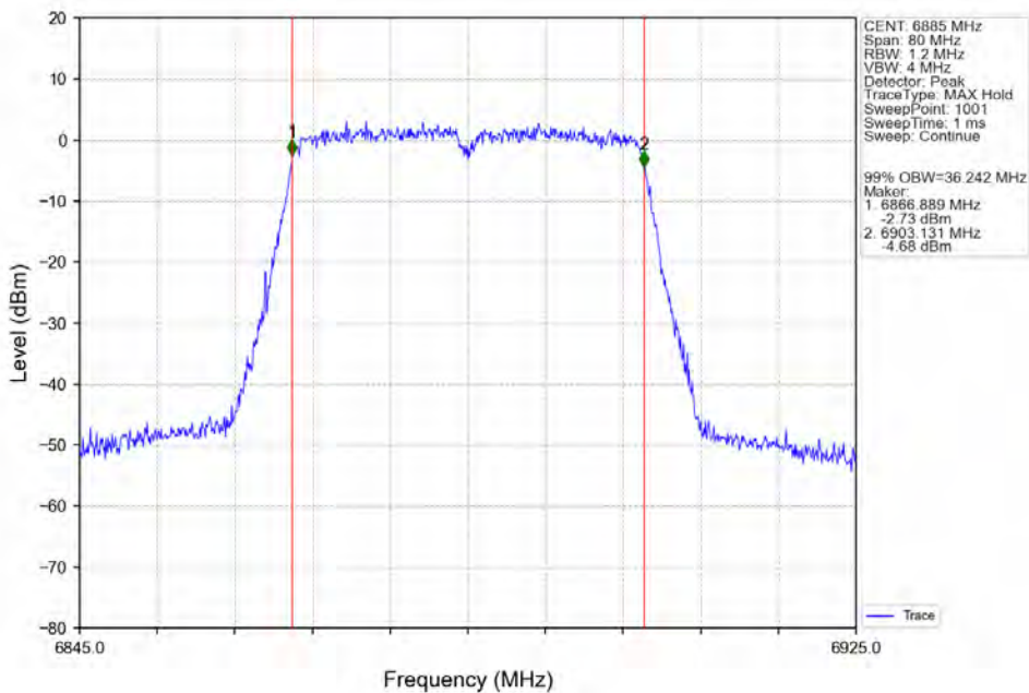
802.11n(HT40) HCH 6885MHz Ant2 NTN
