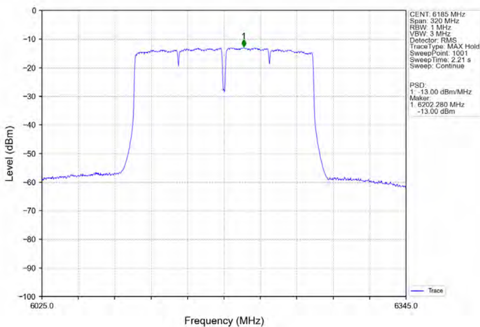
802.11ac(VHT160) MCH 6185MHz MIMO NTN
