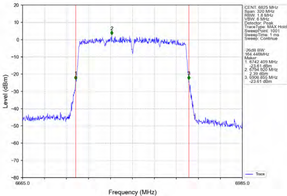
802.11ac(VHT160) HCH 6825MHz Ant2 NTN
