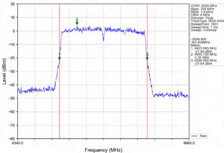
802.11ac(VHT160) HCH 6505MHz Ant2 NTN
