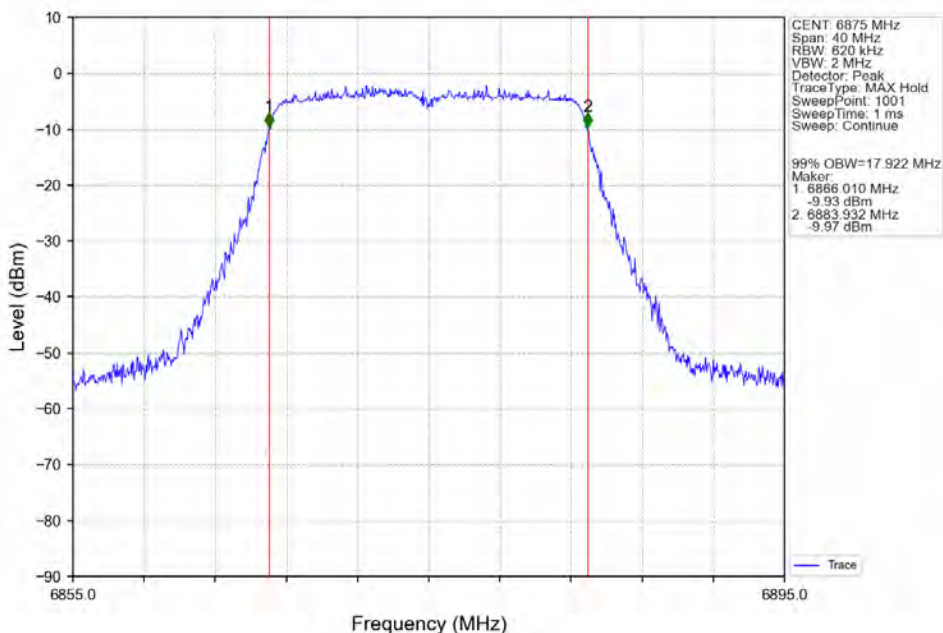
802.11ac(VHT20) HCH 6875MHz Ant2 NTN
