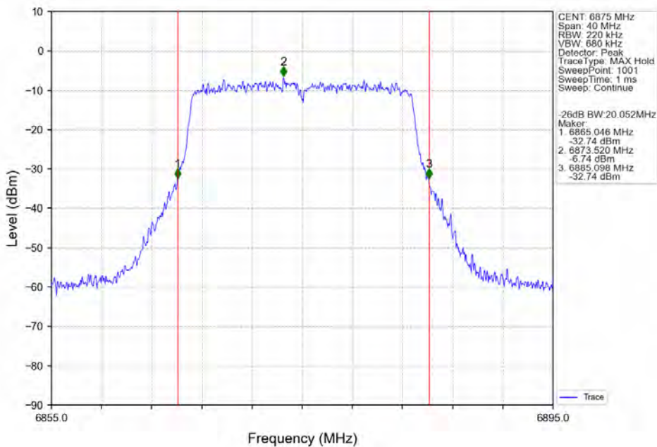
802.11n(HT20) HCH 6875MHz Ant2 NTN
