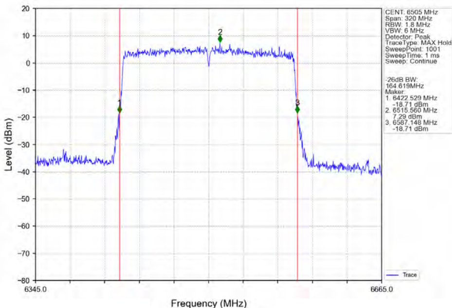
802.11ax(HEW160) HCH 6505MHz SU / Ant2 NTN
