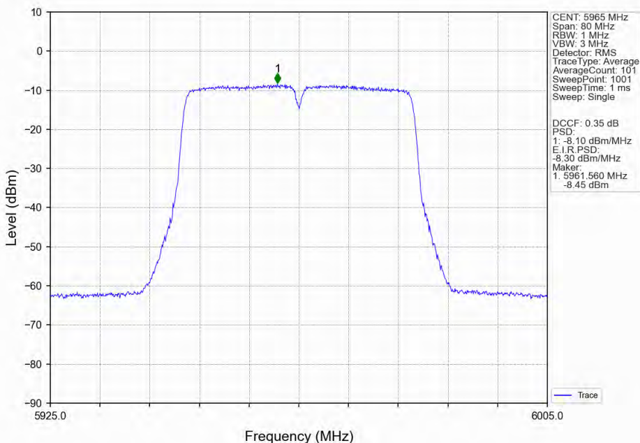
802.11n(HT40) LCH 5965MHz Ant2 NTN
