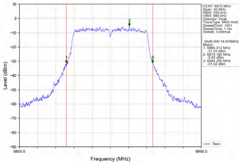
802.11a HCH 6875MHz Ant2 NTN
