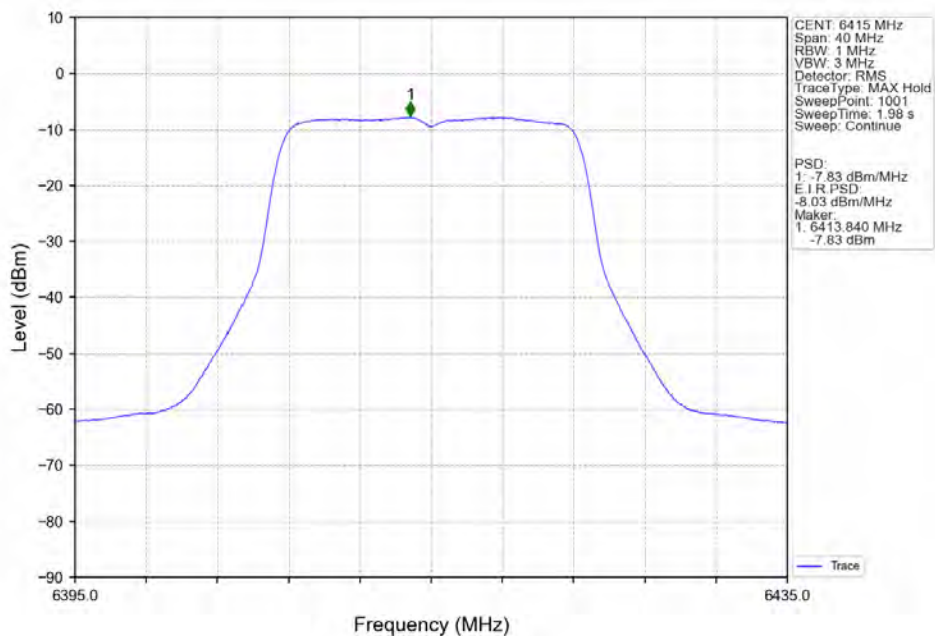
802.11a_HCH_6415MHz_Ant2_NTNV
