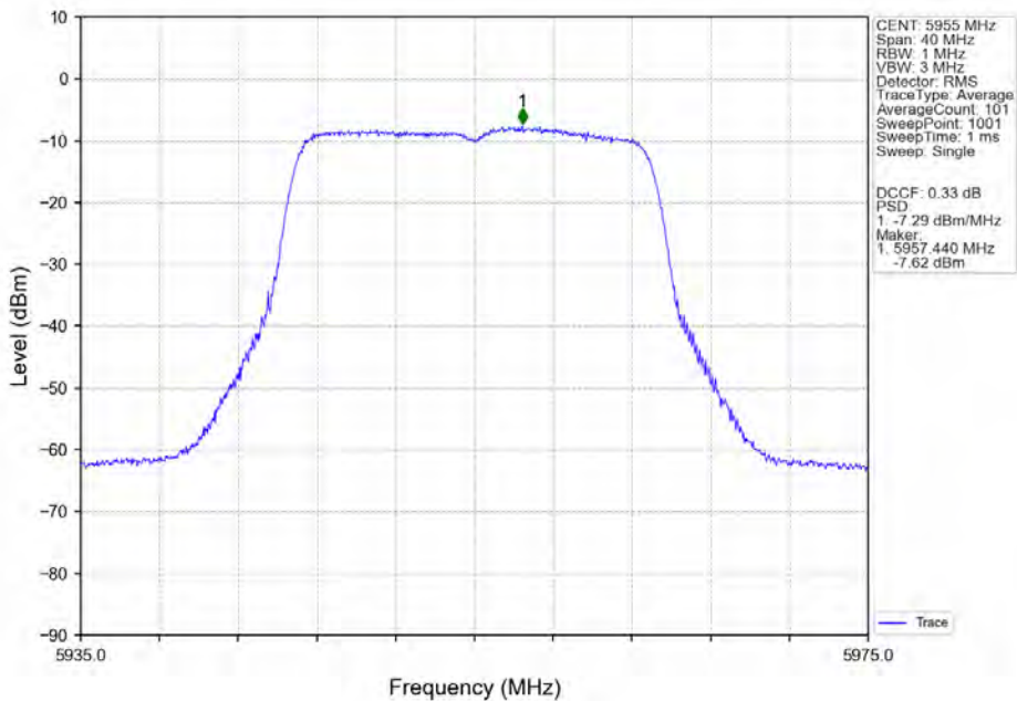
802.11ac(VHT20) LCH 5955MHz Ant1 NTN
