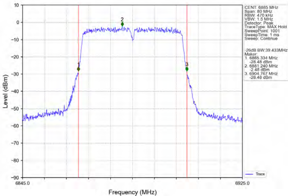
802.11n(HT40) HCH 6885MHz Ant2 NTN
