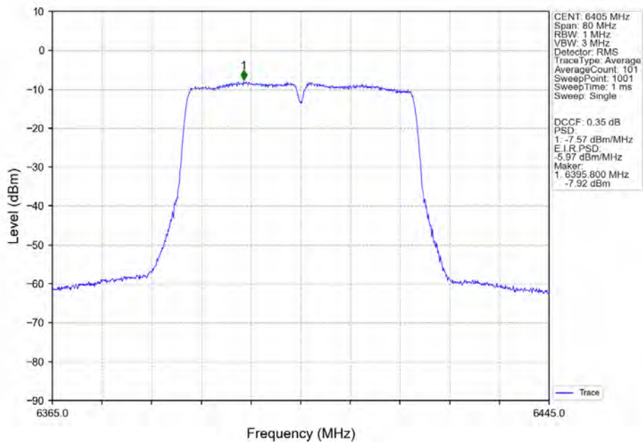
802.11n(HT40) HCH 6405MHz Ant2 NTN
