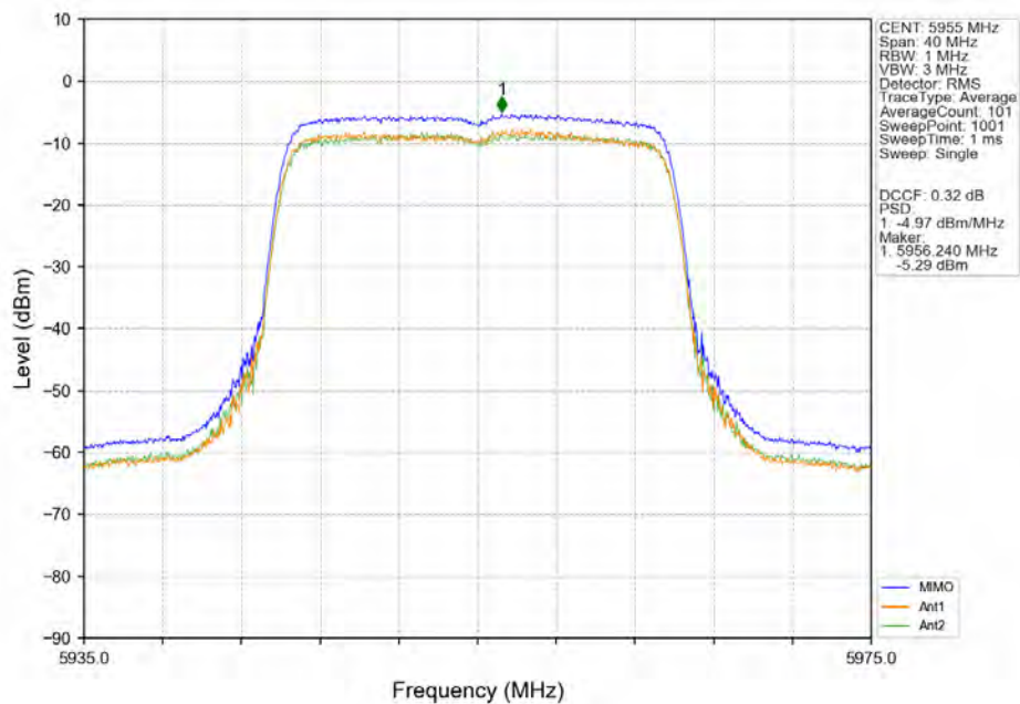
802.11ax(HEW20) LCH 5955MHz SU / MIMO NTN
