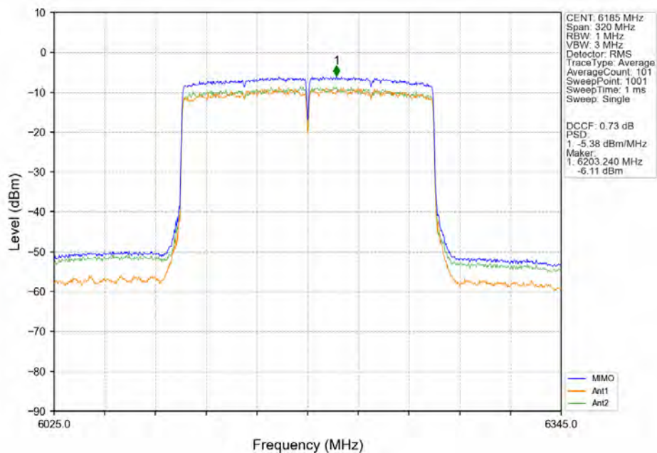
802.11ax(HEW160) MCH 6185MHz SU / MIMO NTN
