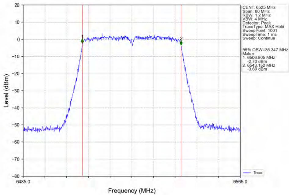
802.11ac(VHT40) HCH 6525MHz Ant2 NTN
