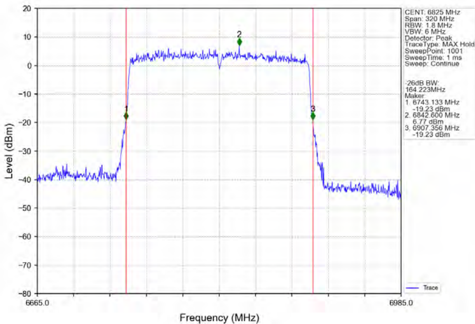
802.11ax(HEW160) HCH 6825MHz SU / Ant2 NTVN
