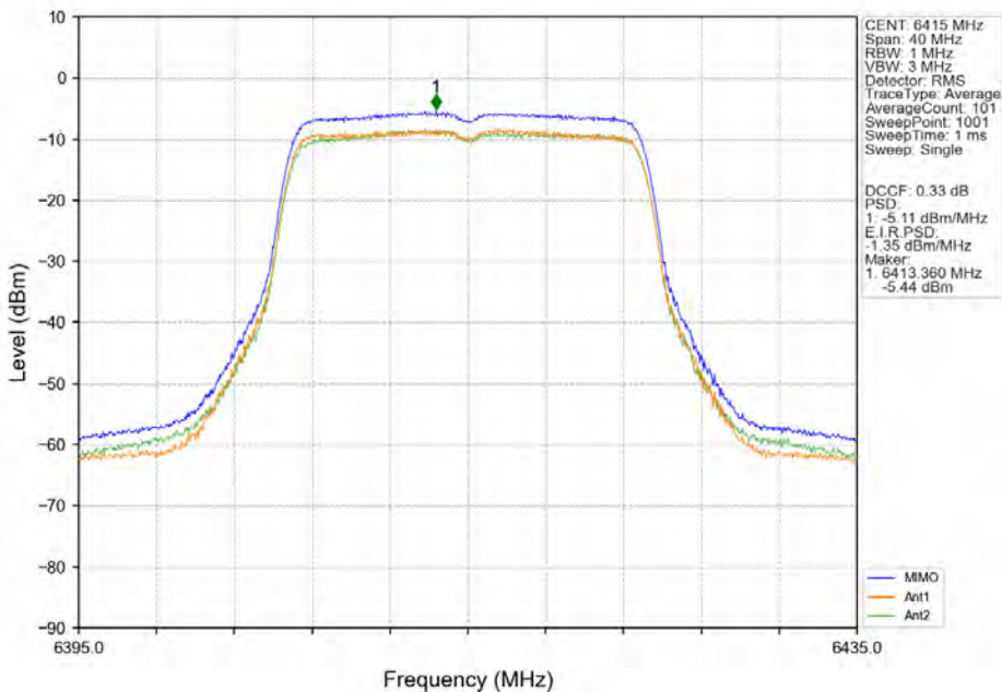
802.11n(HT20) HCH 6415MHz MIMO NTN
