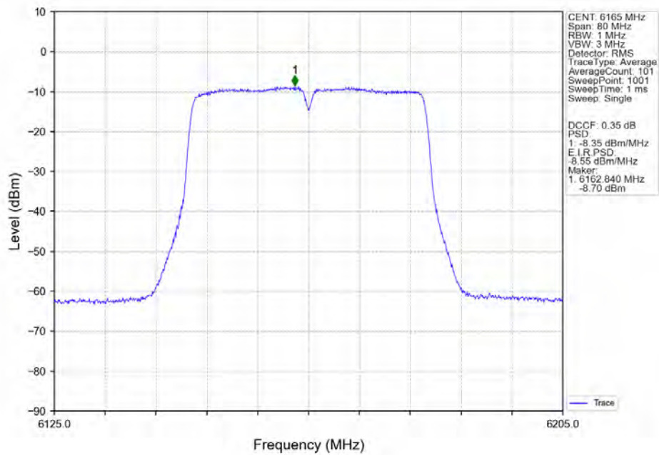
802.11n(HT40) MCH 6165MHz MIMO NTN
