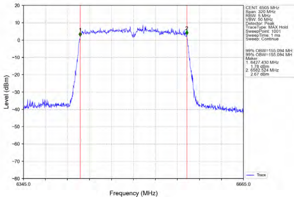
802.11ac(VHT160) HCH 6505MHz Ant2 NTN
