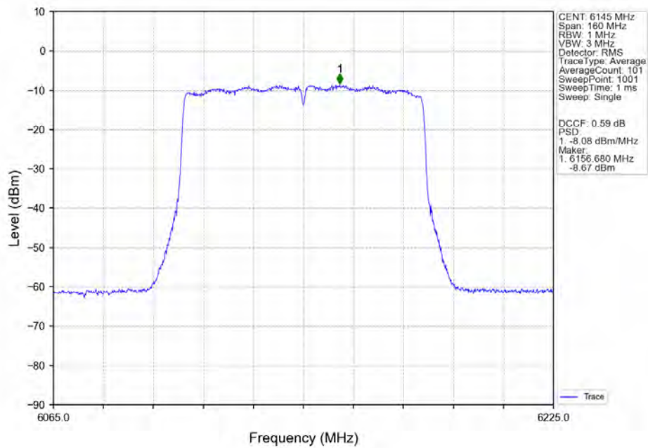
802.11ac(VHT80) MCH 6145MHz Ant2 NTN
