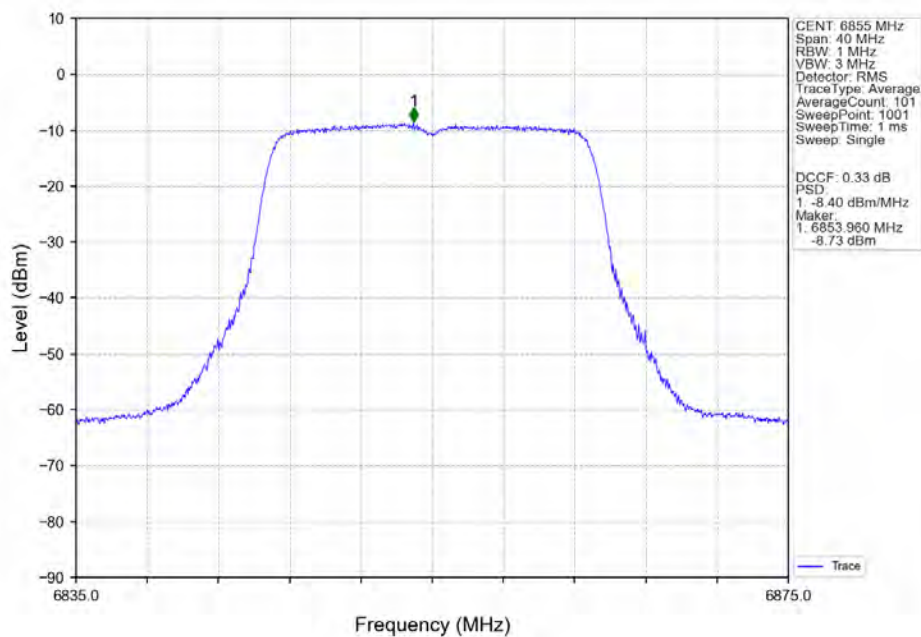
802.11n(HT20)_HCH_6855MHz_MIMO_NTNV
