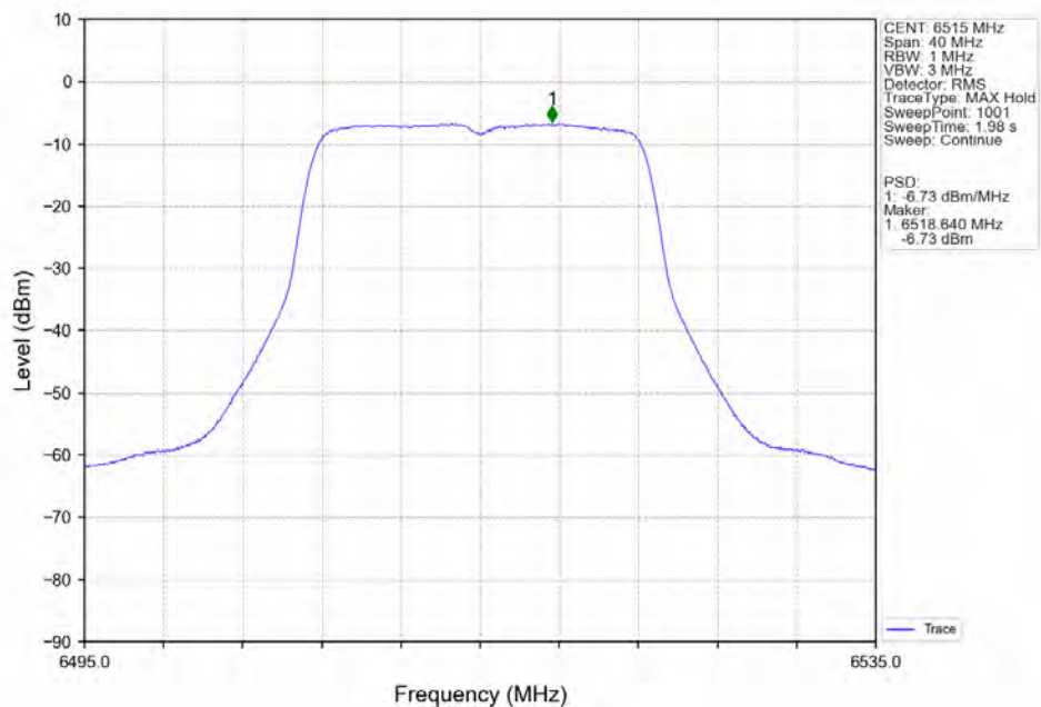
802.11a_HCH_6515MHz_Ant2_NTNV
