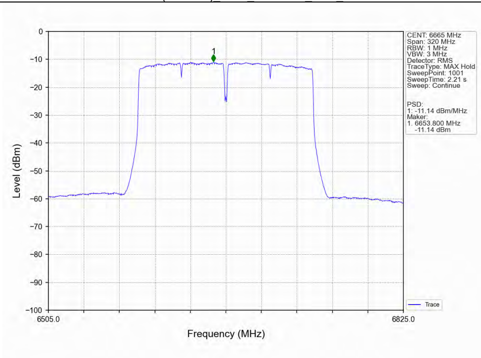
802.11ac(VHT160) MCH_6665MHz_Ant2_NTNV
