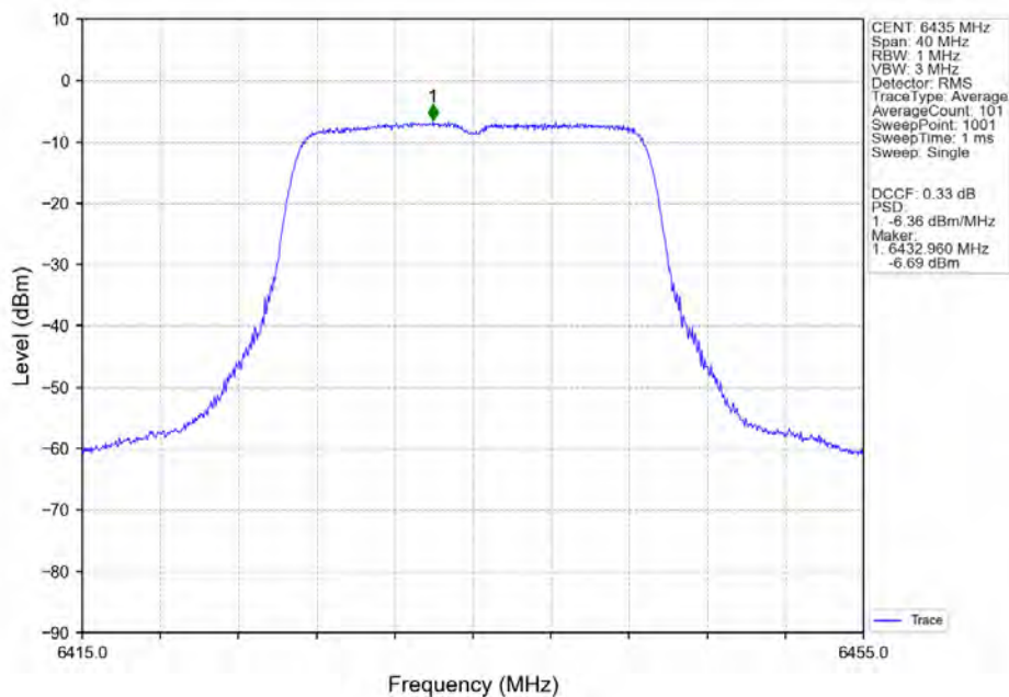
802.11ac(VHT20) LCH_6435MHz_Ant2_NTNV
