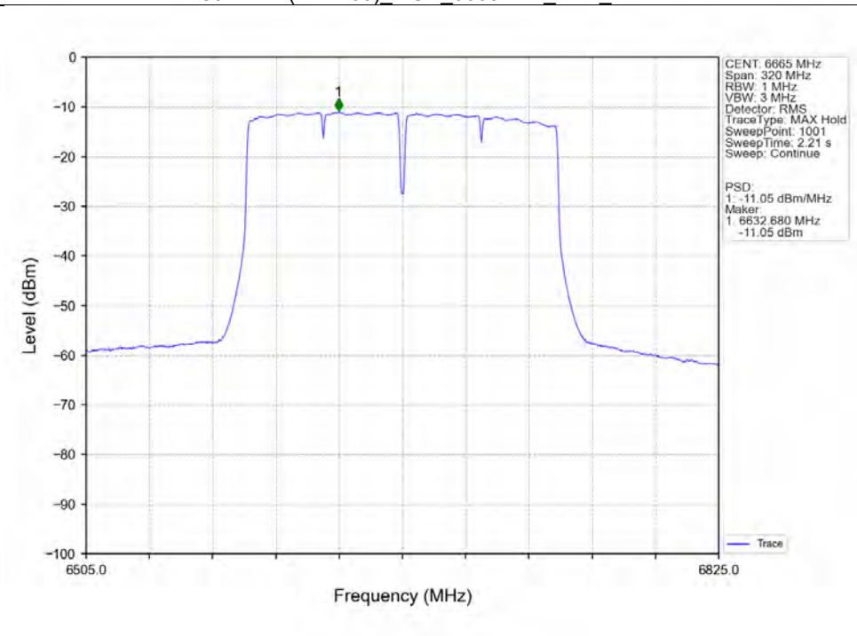
802.11ac(VHT160) MCH_6665MHz_Ant2_NTNV
