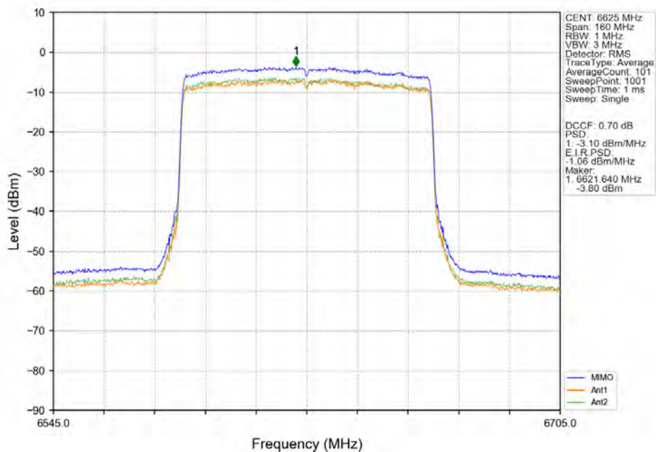
802.11ax(HEW80) LCH 6625MHz SU / MIMO NTN
