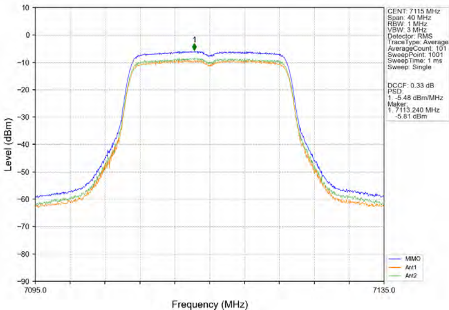
802.11ac(VHT20) HCH 7115MHz MIMO NTN
