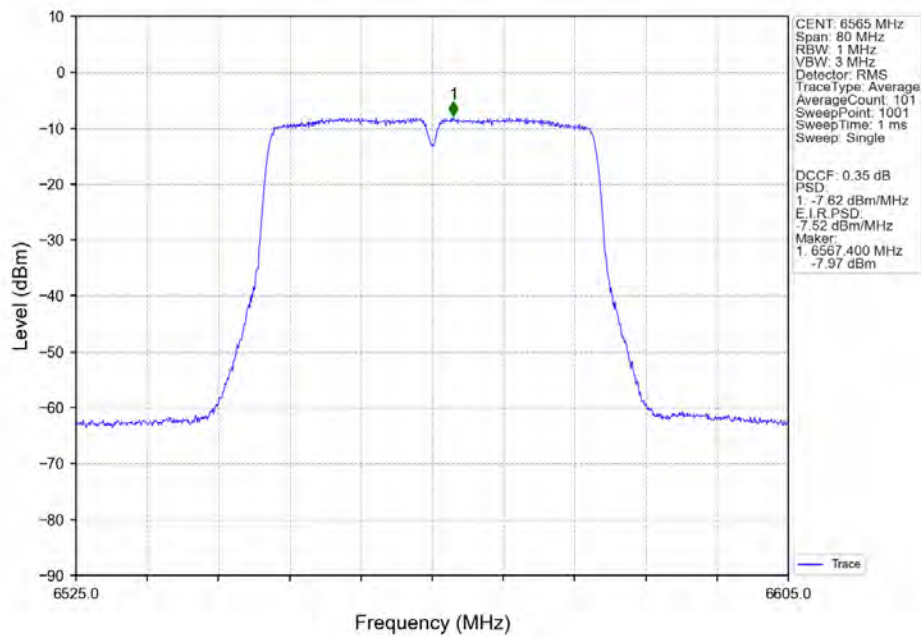
802.11n(HT40) LCH 6565MHz Ant2 NTN
