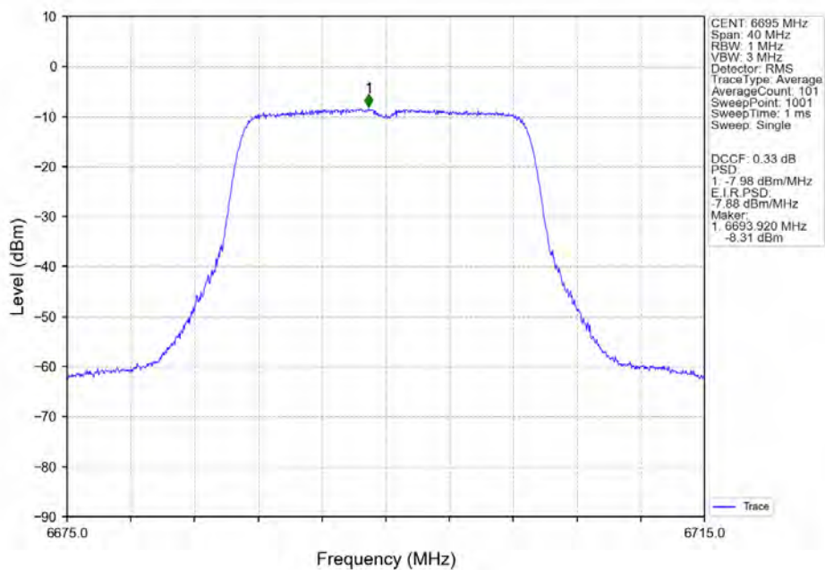
802.11n(HT20) MCH 6695MHz Ant2 NTN
