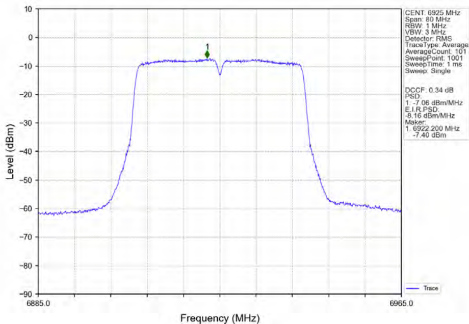
802.11ac(VHT40) LCH_6925MHz_Ant2_NTNV
