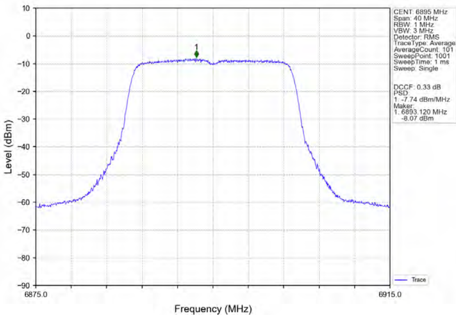
802.11ac(VHT20) LCH 6895MHz MIMO NTN
