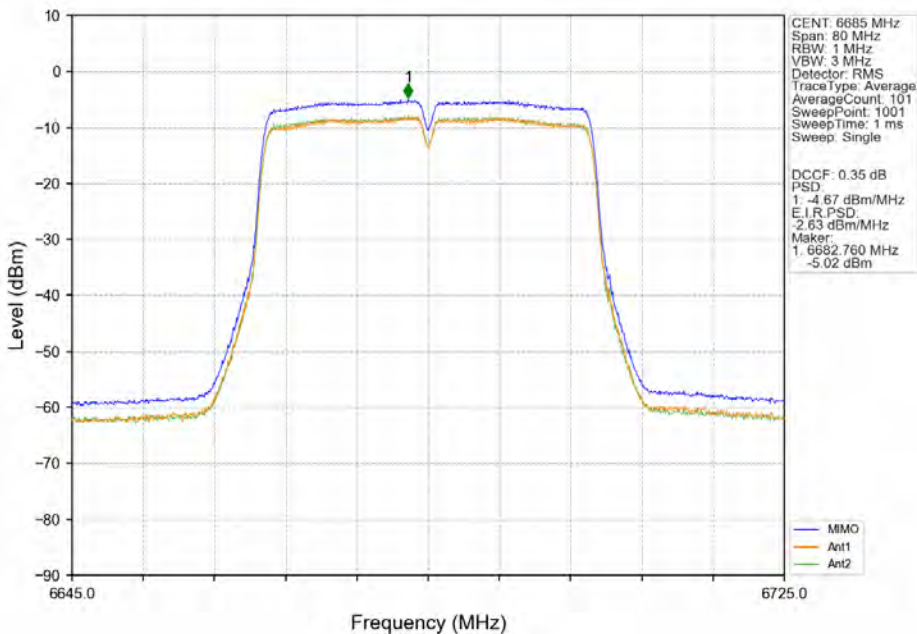
802.11n(HT40) MCH 6685MHz MIMO NTN
