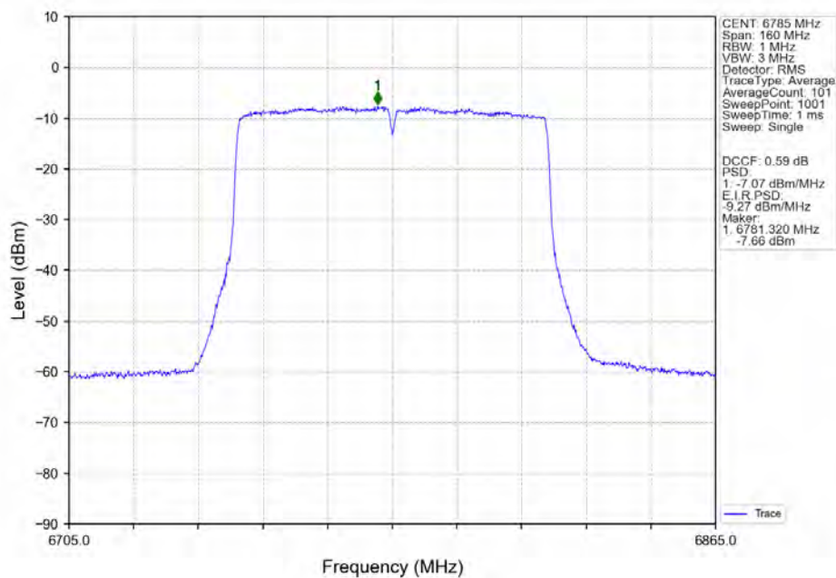
802.11ac(VHT80) HCH 6785MHz MIMO NTN
