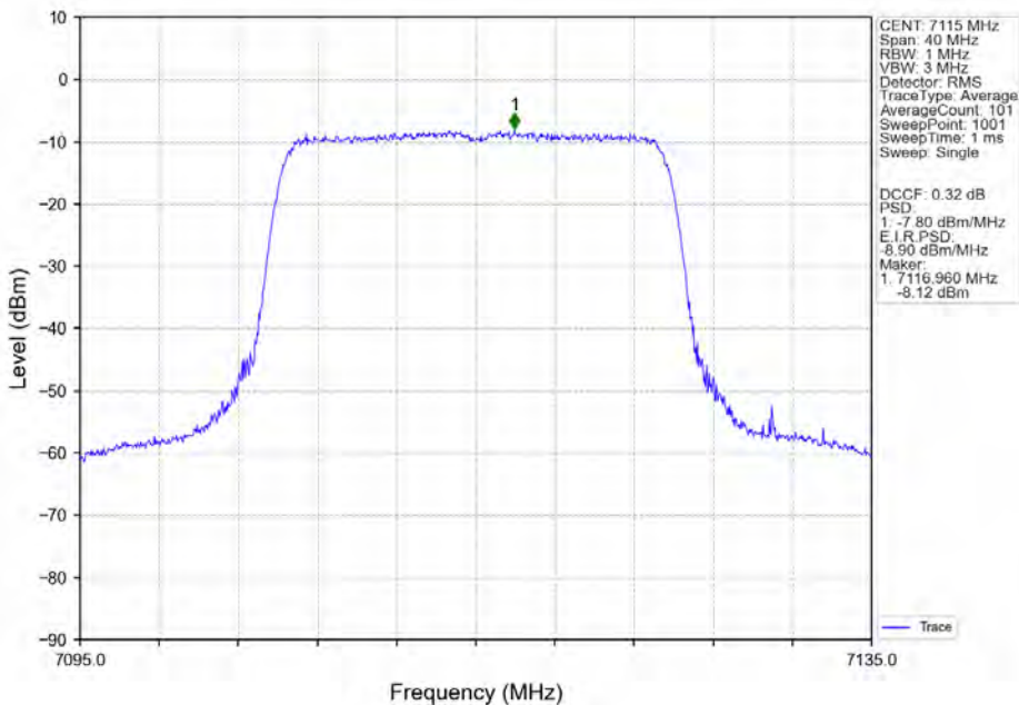
802.11ax(HEW20) HCH 7115MHz SU / Ant2 NTN
