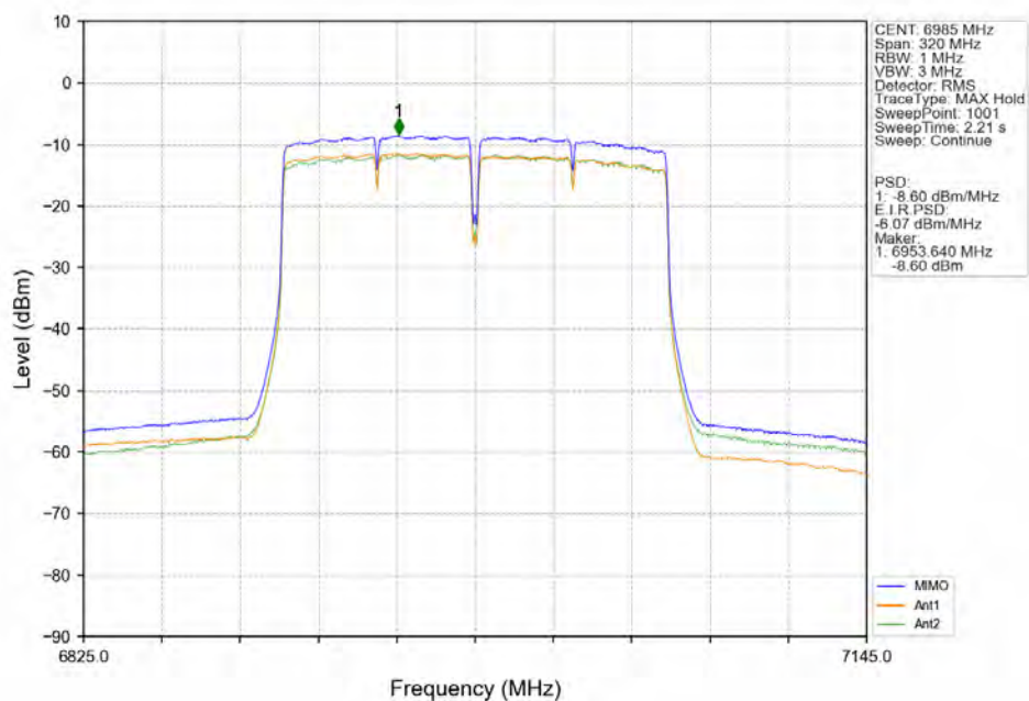
802.11ac(VHT160) MCH_6985MHz_MIMO_NTNV
