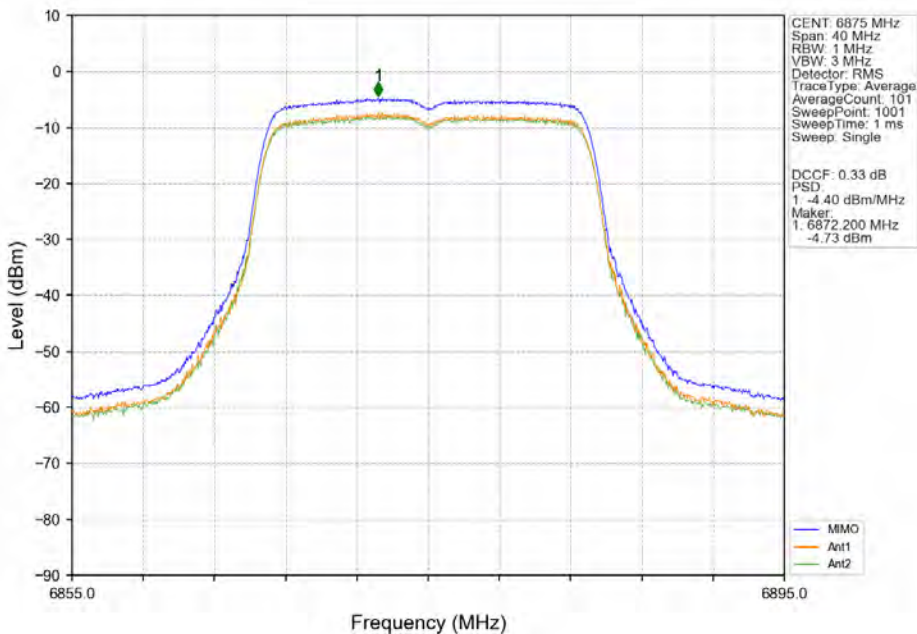
802.11ac(VHT20) HCH 6875MHz MIMO NTN
