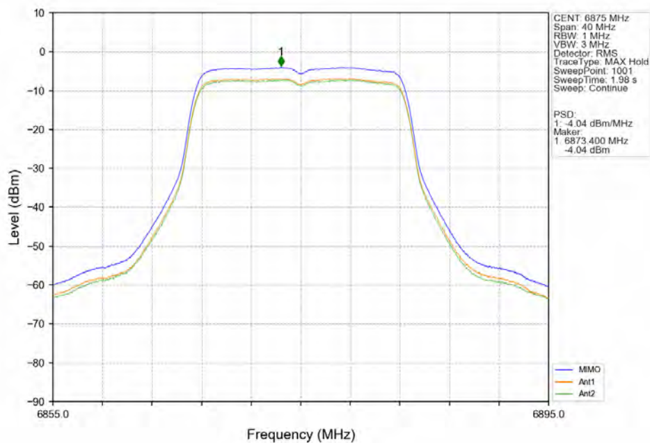
802.11n(HT20) HCH 6875MHz Ant1 NTN
