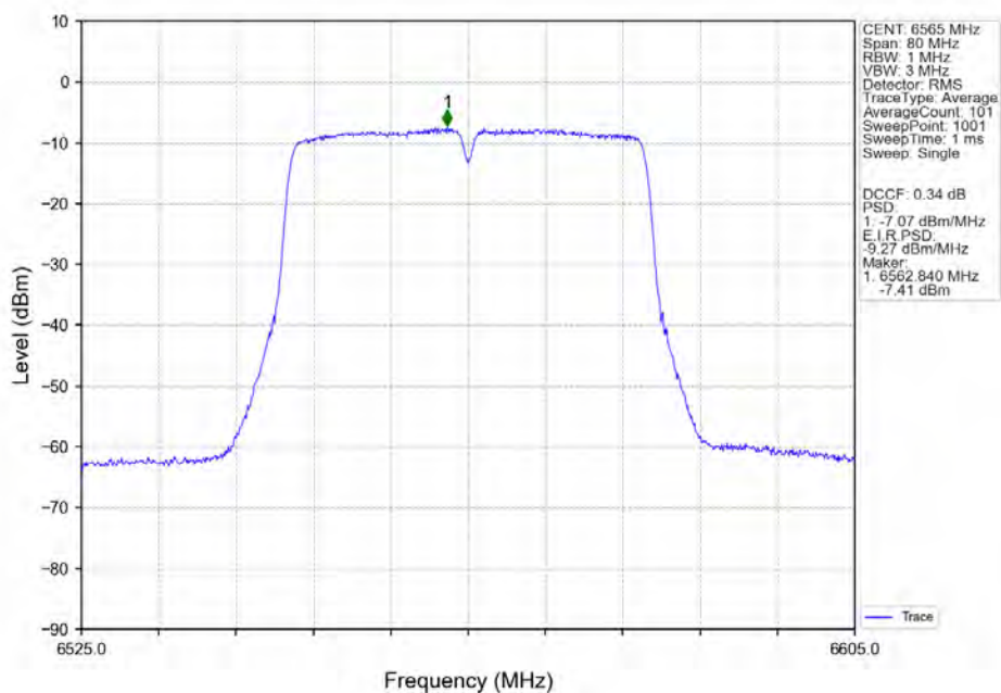
802.11ac(VHT40) LCH_6565MHz_Ant2_NTNV
