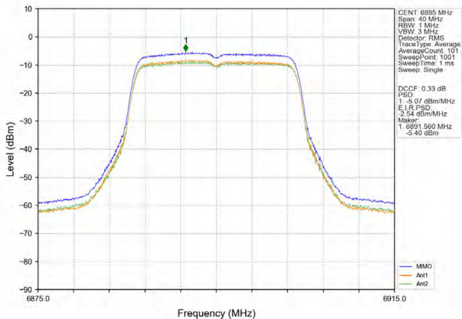
802.11n(HT20) LCH 6895MHz MIMO NTN
