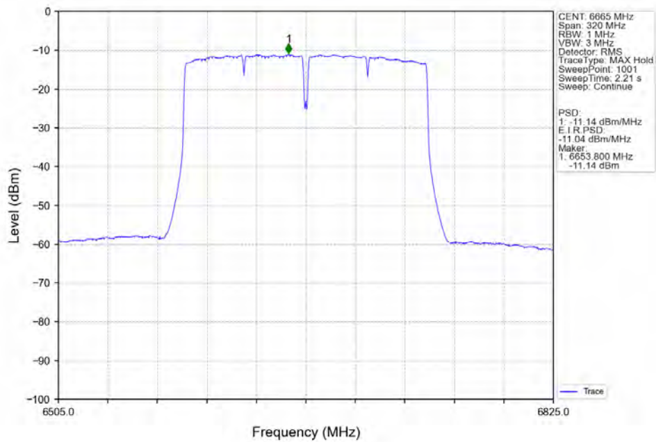
802.11ac(VHT160) MCH_6665MHz_Ant2_NTNV
