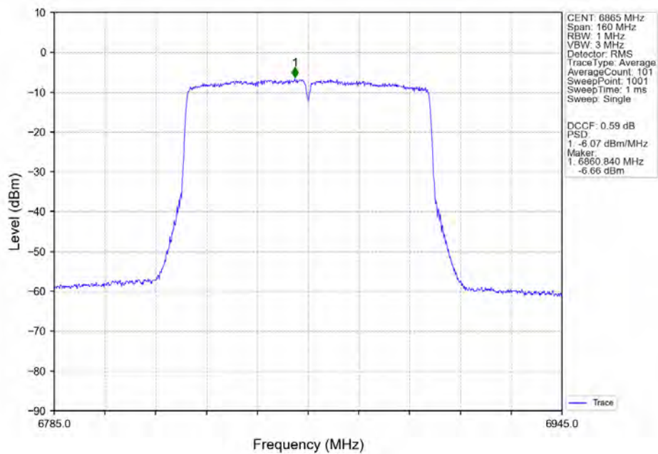
802.11ac(VHT80) HCH_6865MHz_Ant1_NTNV
