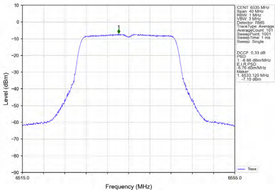
802.11ac(VHT20) LCH 6535MHz Ant1 NTN
