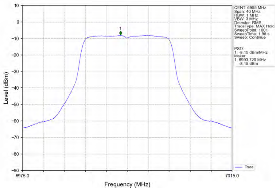
802.11a MCH 6995MHz MIMO NTN
