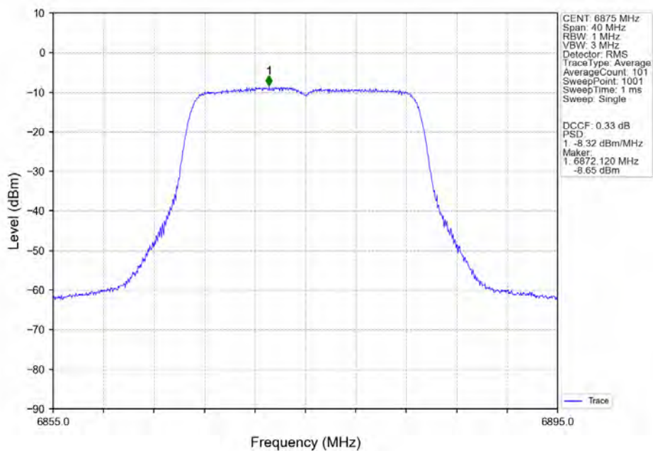
802.11n(HT20)_HCH_6875MHz_MIMO_NTNV
