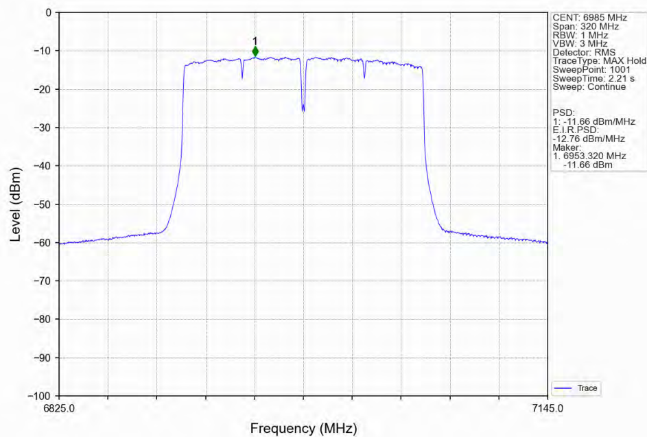
802.11ac(VHT160) MCH_6985MHz_MIMO_NTNV
