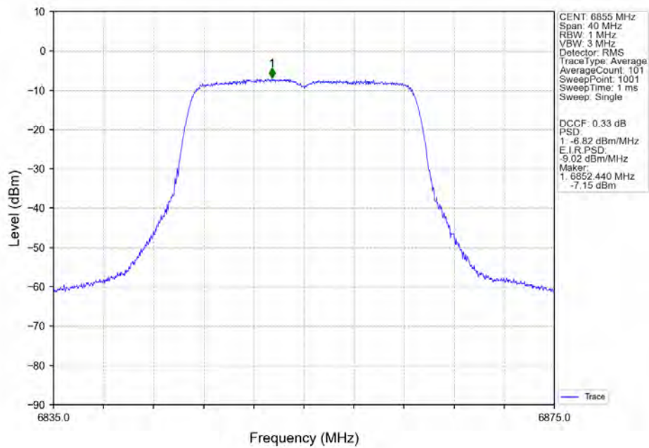
802.11ac(VHT20) HCH 6855MHz MIMO NTN
