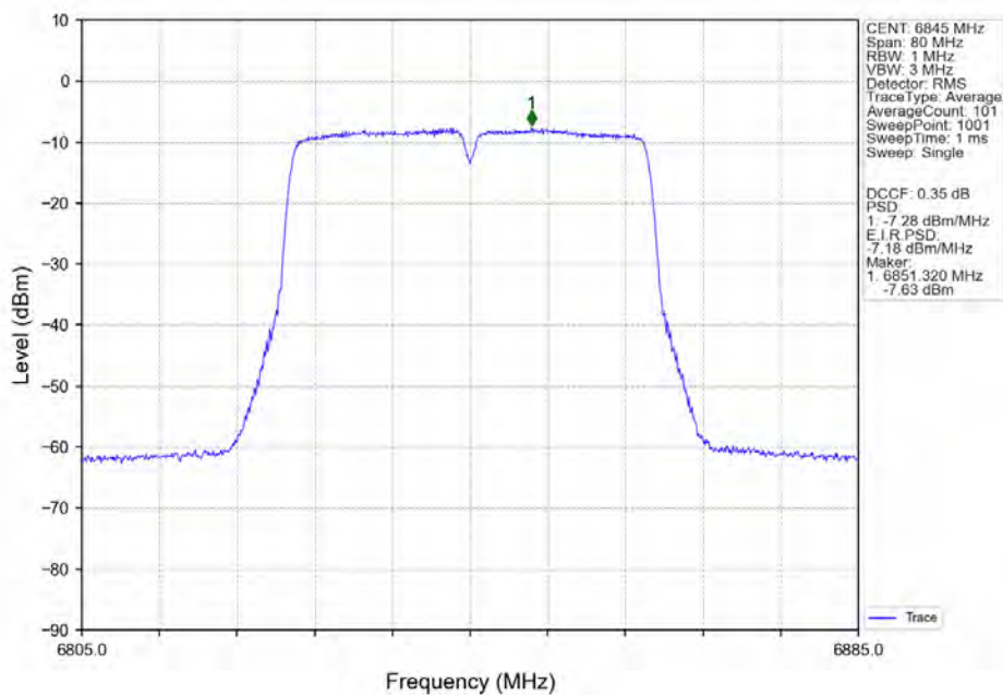
802.11n(HT40) HCH 6845MHz_Ant2_NTNV
