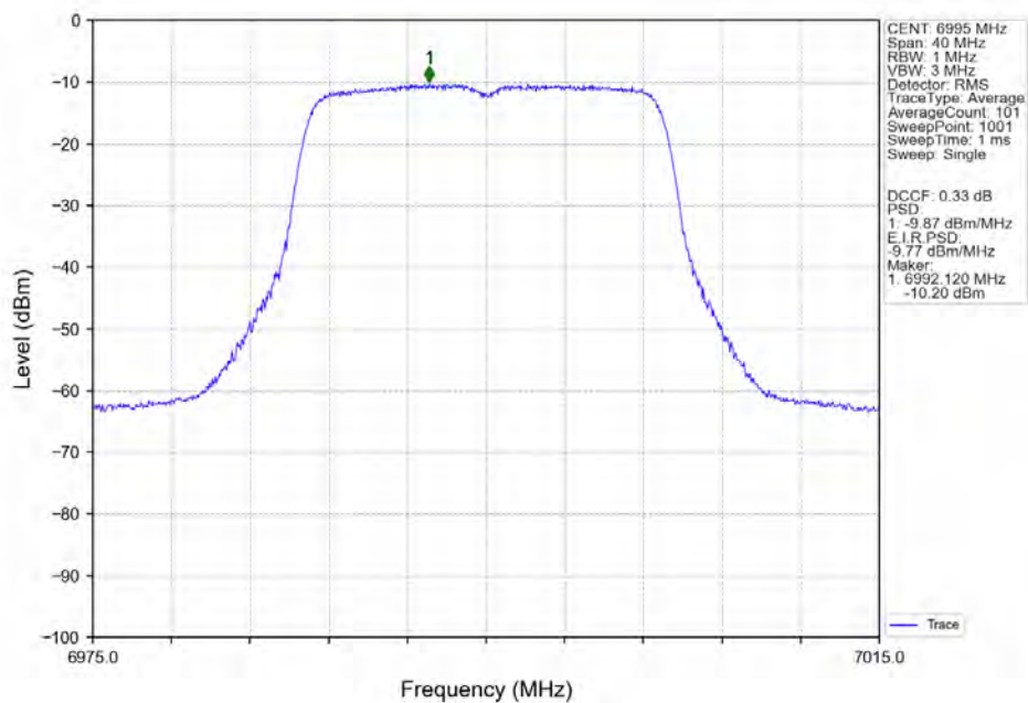
802.11n(HT20) MCH 6995MHz Ant2 NTN
