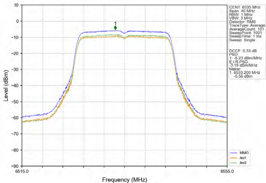
802.11n(HT20) LCH 6535MHz MIMO NTN
