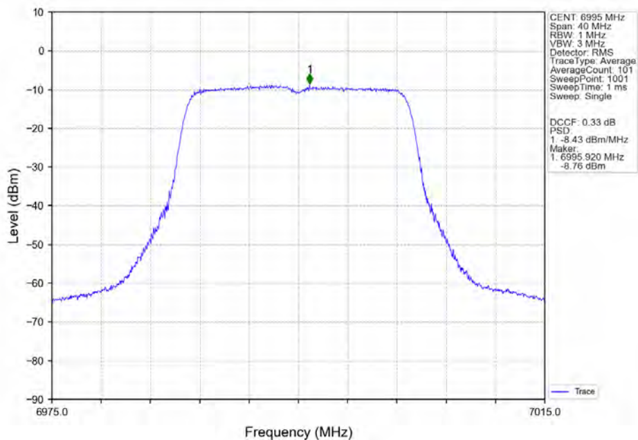
802.11ac(VHT20) MCH 6995MHz Ant2 NTV
