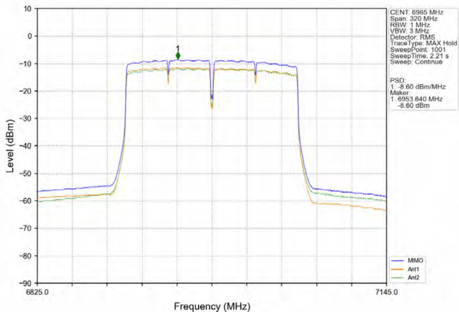
802.11ac(VHT160) MCH_6985MHz_MIMO_NTNV
