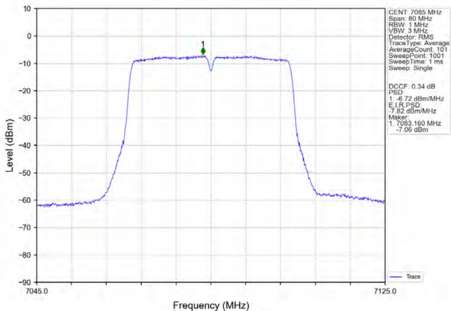
802.11ac(VHT40) HCH 7085MHz Ant2 NTN
