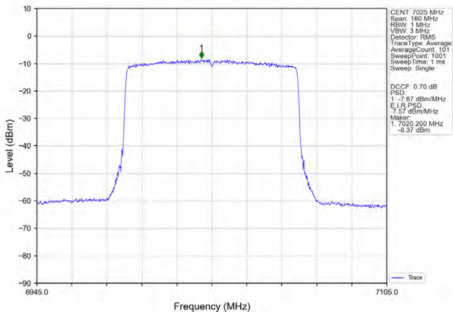
802.11ax(HEW80) HCH 7025MHz SU / Ant1 NTN
