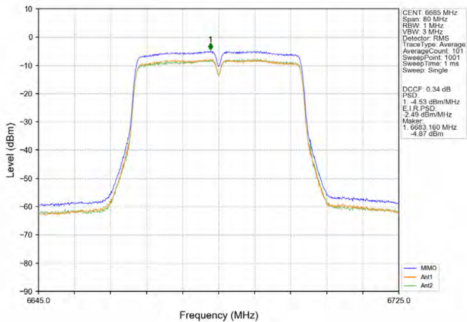
802.11ac(VHT40) MCH_6685MHz_MIMO_NTNV
