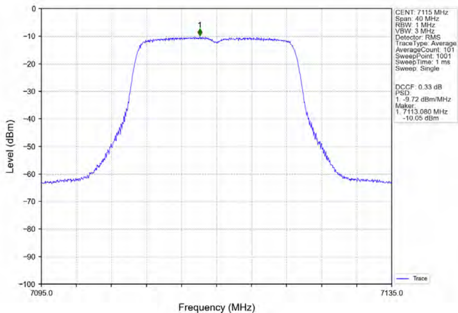
802.11n(HT20) HCH 7115MHz Ant1 NTN
