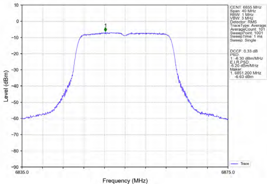
802.11ac(VHT20) HCH_6855MHz_Ant1_NTNV
