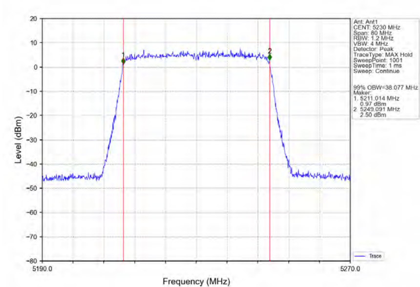
802.11ax(HEW40) HCH 5230MHz RU484 Left Ant1 NTN
