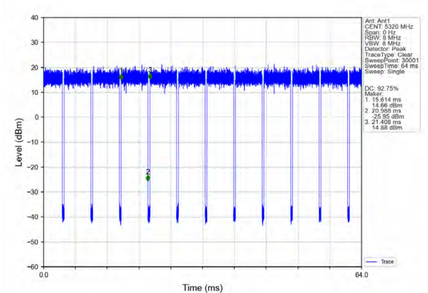
802.11ac(VHT20) HCH_5320MHz_Ant1_NTNV
