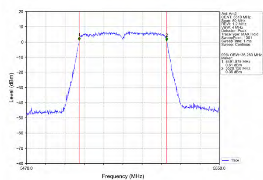
802.11ac(VHT40) LCH_5510MHz_Ant2_NTNV
