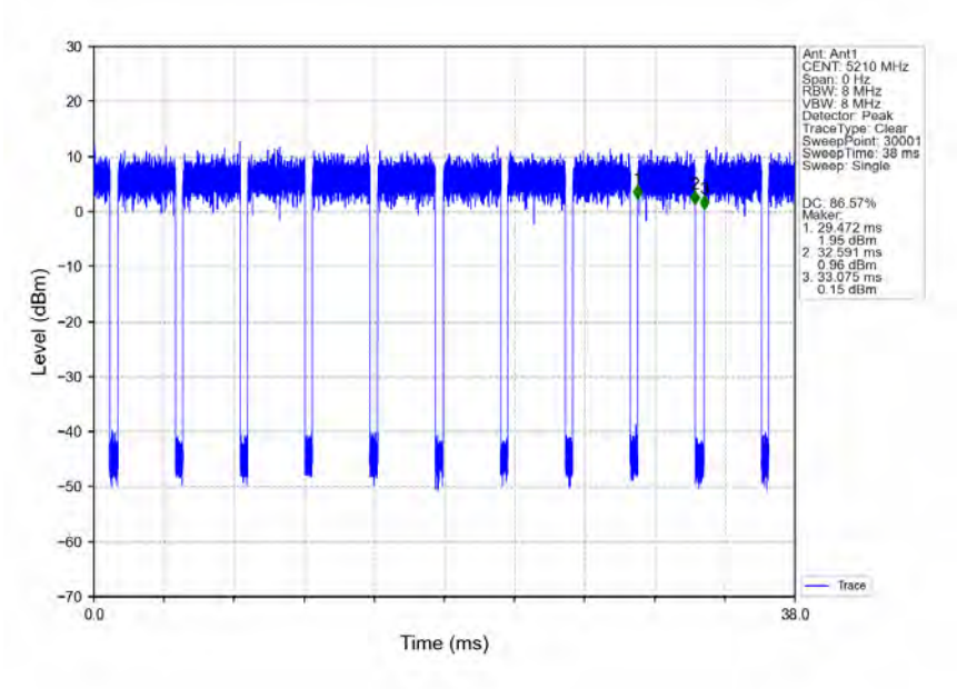
802.11ac(VHT80) MCH 5210MHz Ant1 NTN
