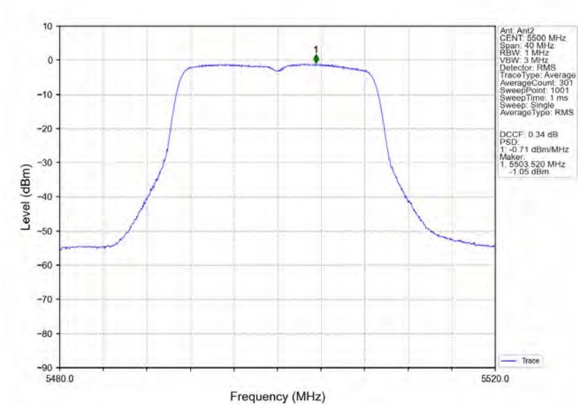
802.11ac(VHT20) LCH_5500MHz_Ant2_NTNV
