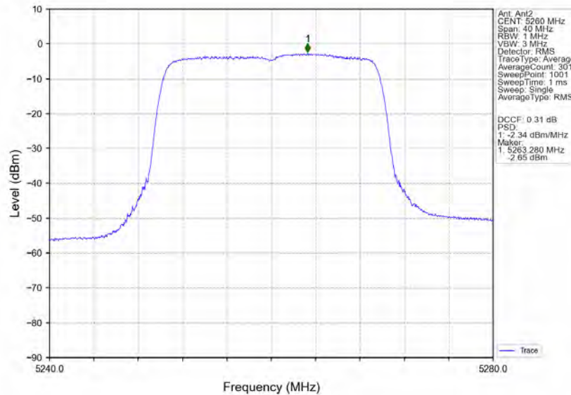
802.11ax(HEW20) LCH 5260MHz RU242 Left MIMO NTNW
