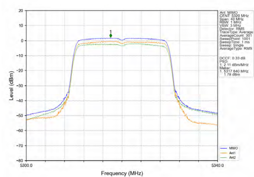
802.11ax(HEW20) HCH 5320MHz RU242 Left MIMO NTNW
