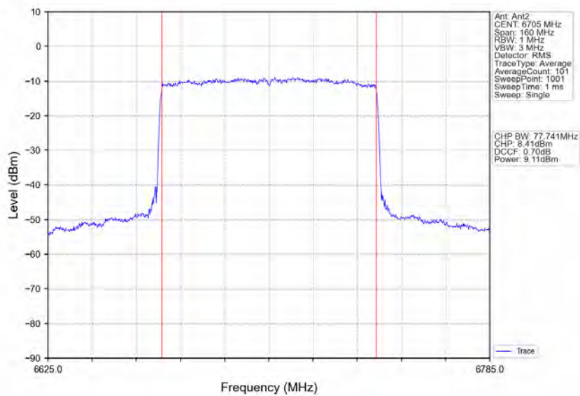
802.11ax(HEW80)_MCH_6705MHz_RU996_Left_Ant2_NTNV
