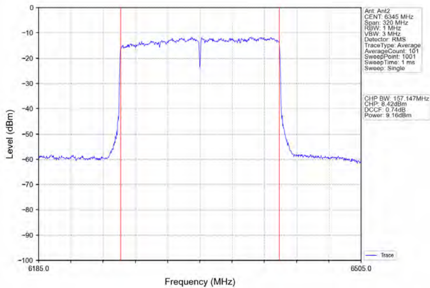
802.11ax(HEW160) HCH_6345MHz_2xRU996_Left_Ant2_NTNV
