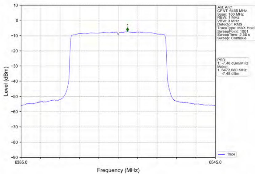
802.11ax(HEW80) LCH 6465MHz RU996 Left Ant1 NTN
