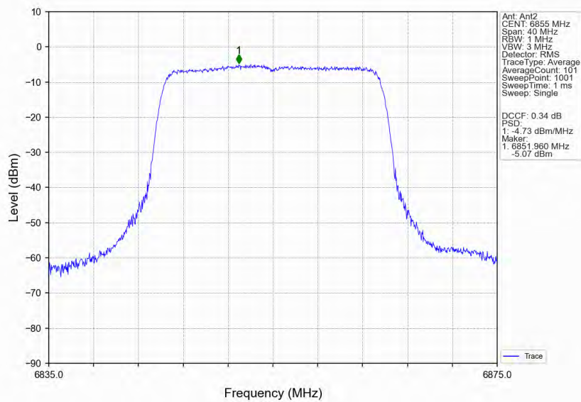
802.11ax(HEW20) HCH 6855MHz RU242 Left Ant2 NTVN
