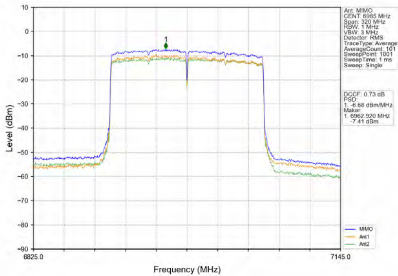
802.11ax(HEW160) MCH 6985MHz 2xRU996 Left MIMO NTVN
