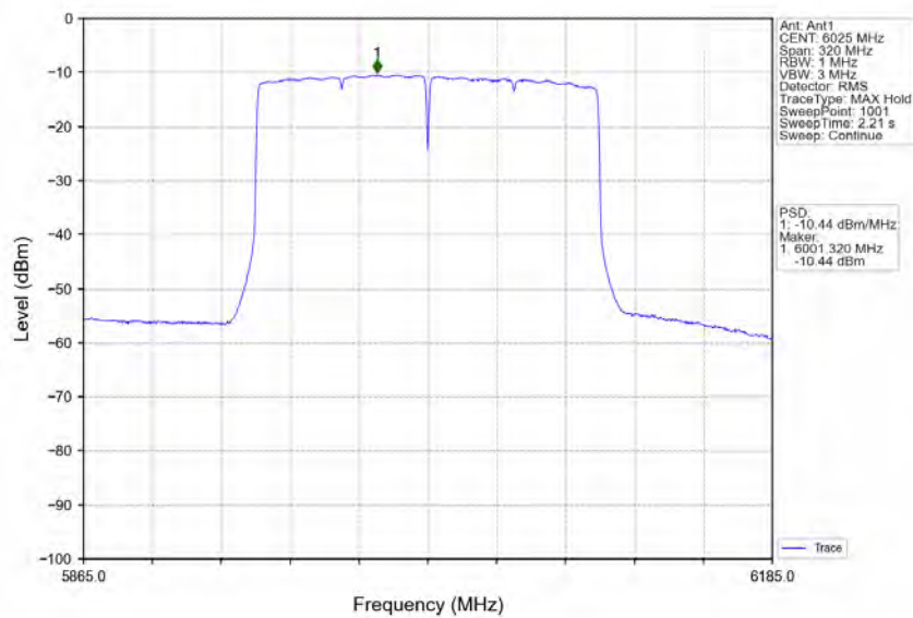
802.11ax(HEW160) LCH 6025MHz 2xRU996 Left Ant1 NTN
