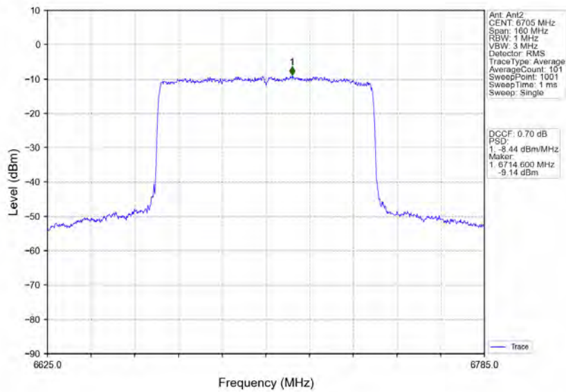
802.11ax(HEW80) MCH 6705MHz RU996 Left MIMO NTN
