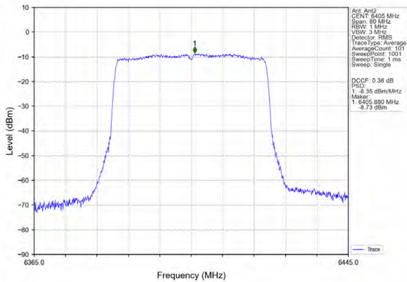
802.11ax(HEW40) HCH 6405MHz RU484 Left MIMO NTN
