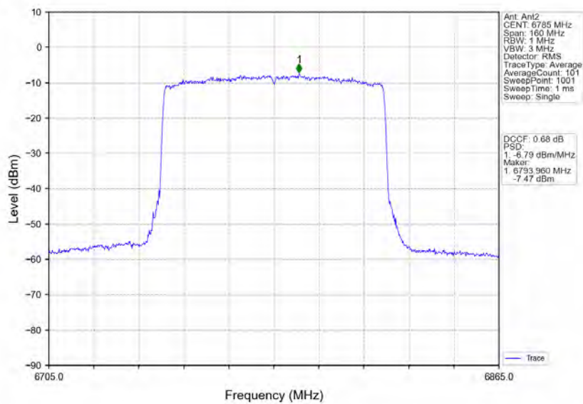
802.11ax(HEW80) HCH 6785MHz RU996 Left Ant2 NTVN
