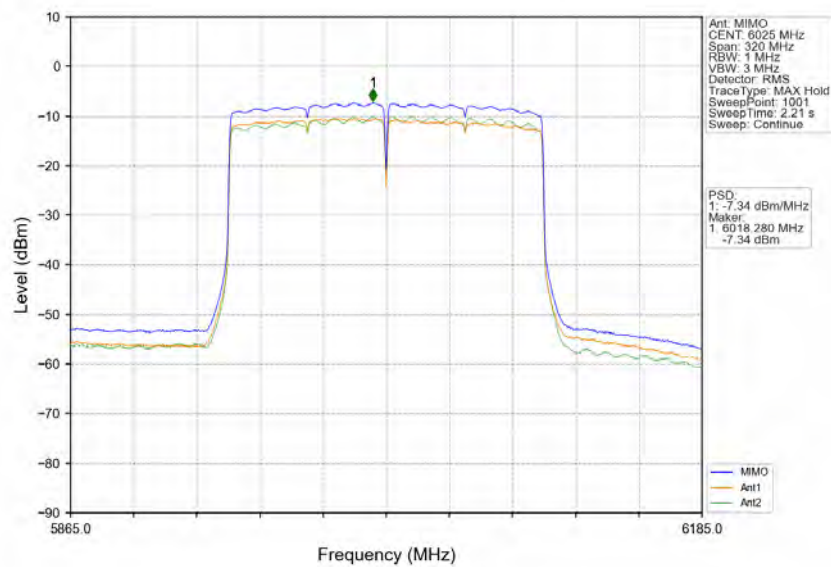
802.11ax(HEW160) LCH 6025MHz 2xRU996 Left MIMO NTN
