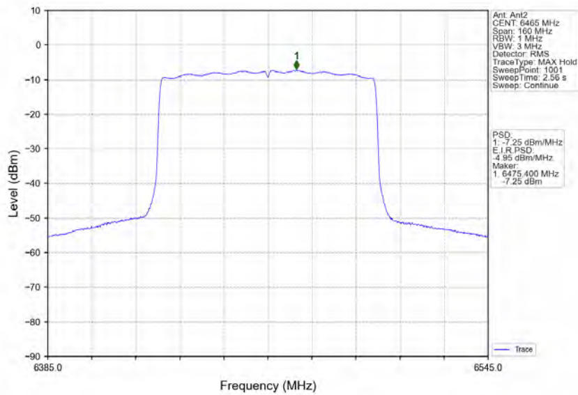
802.11ax(HEW80) LCH_6465MHz_RU996_Left_MIMO_NTNV
