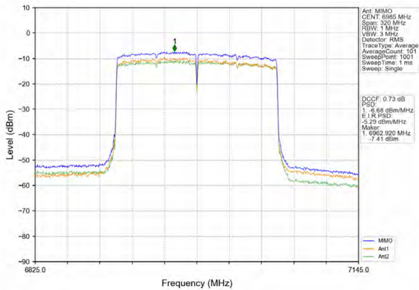
802.11ax(HEW160) MCH 6985MHz 2xRU996 Left MIMO NTV
