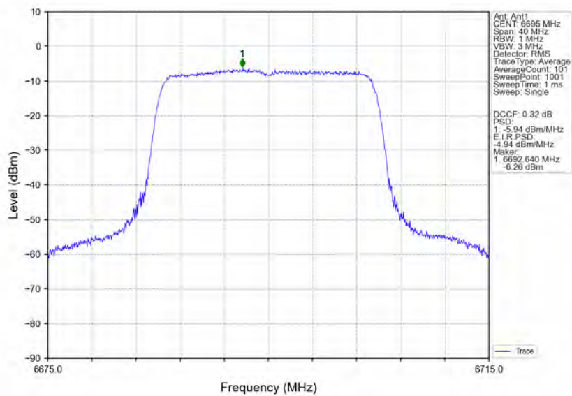
802.11ax(HEW20) MCH 6695MHz RU242 Left Ant1 NTN
