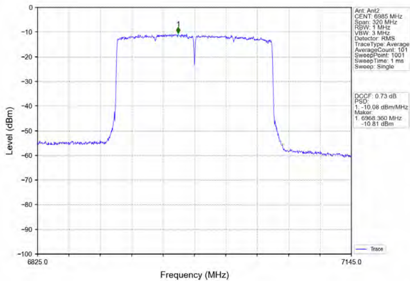
802.11ax(HEW160) MCH_6985MHz_2xRU996_Left_Ant2_NTNV
