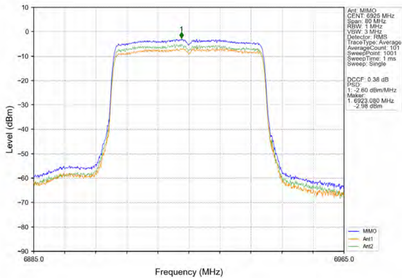
802.11ax(HEW40) LCH 6925MHz RU484 Left MIMO NTN
