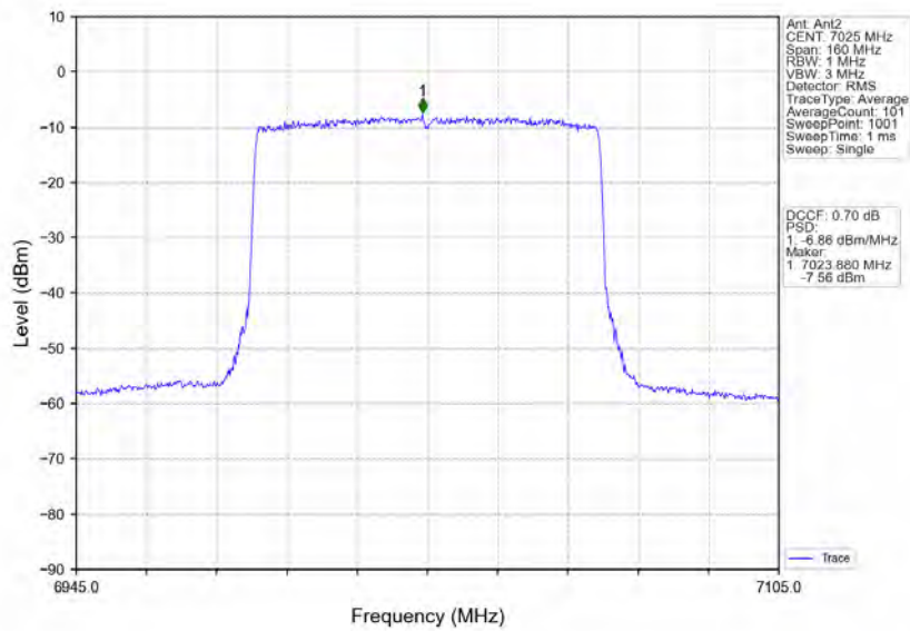
802.11ax(HEW80) HCH 7025MHz RU996 Left MIMO NTN
