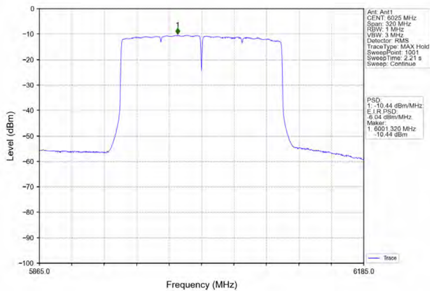
802.11ax(HEW160) LCH 6025MHz 2xRU996 Left Ant1 NTNW
