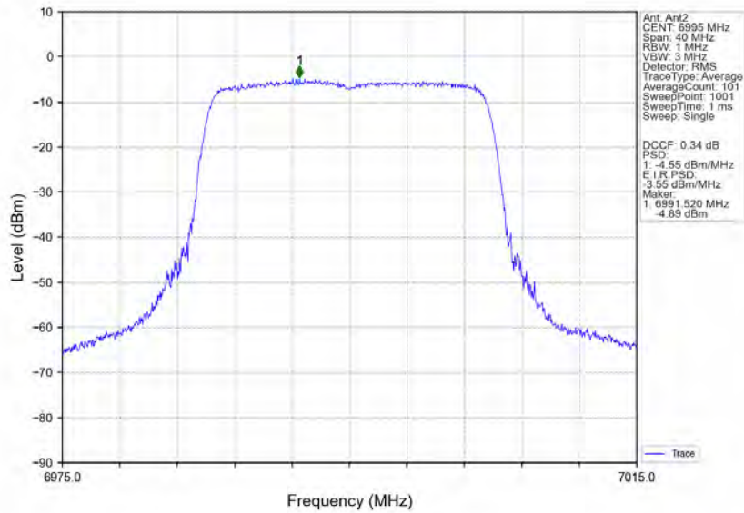
802.11ax(HEW20) MCH 6995MHz RU242 Left MIMO NTN
