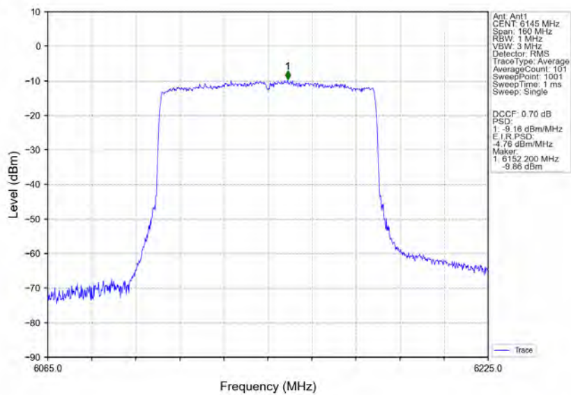
802.11ax(HEW80) MCH 6145MHz RU996 Left Ant1 NTN
