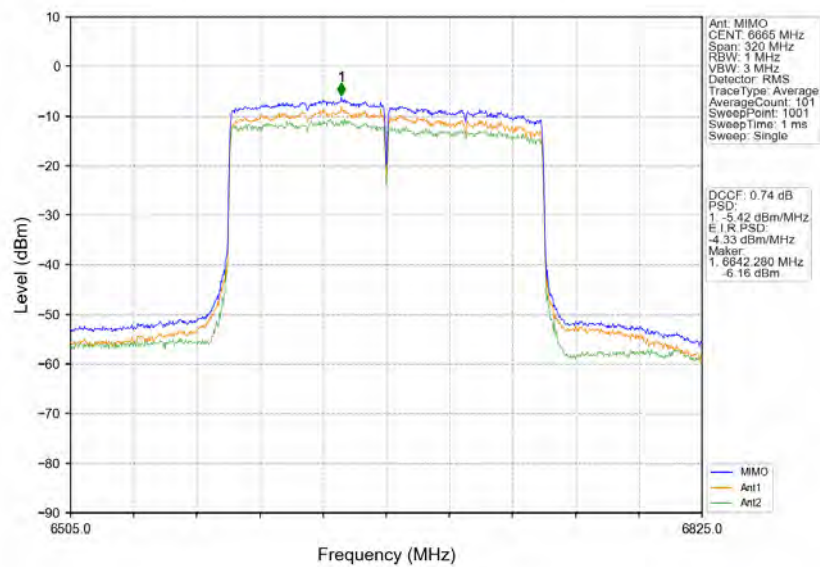
802.11ax(HEW160) MCH 6665MHz 2xRU996 Left MIMO NTV
