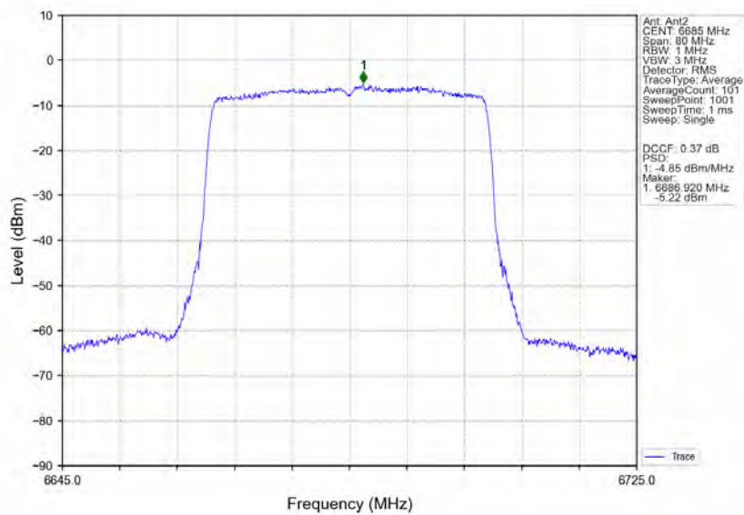
802.11ax(HEW40)_MCH_6685MHz_RU484_Left_Ant2_NTNV
