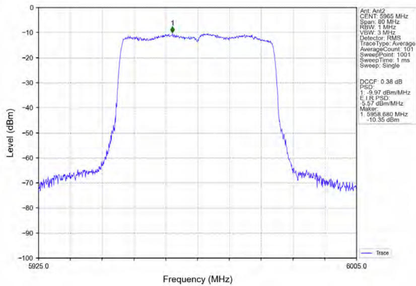
802.11ax(HEW40) LCH 5965MHz RU484 Left MIMO NTN
