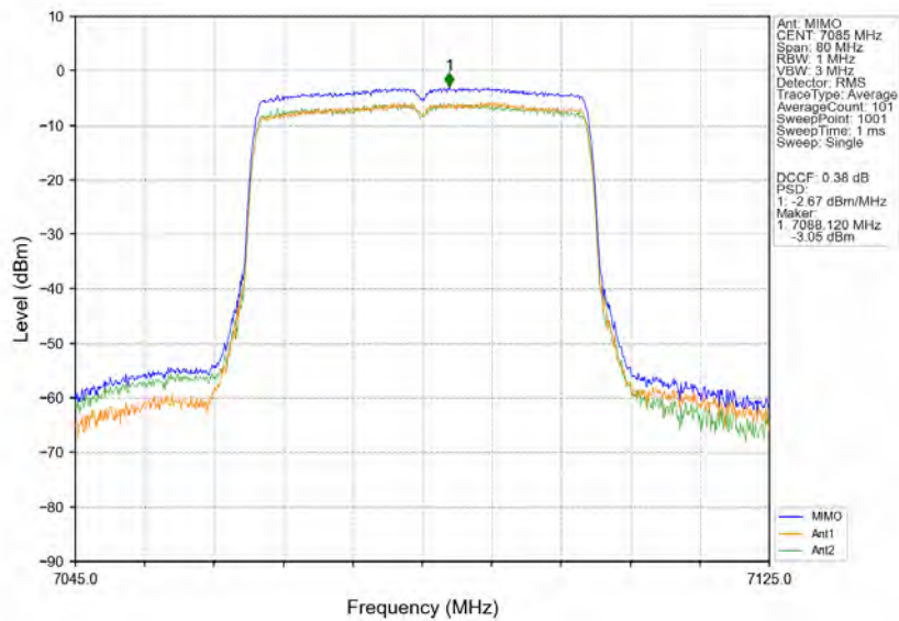
802.11ax(HEW40) HCH 7085MHz RU484 Left MIMO NTN
