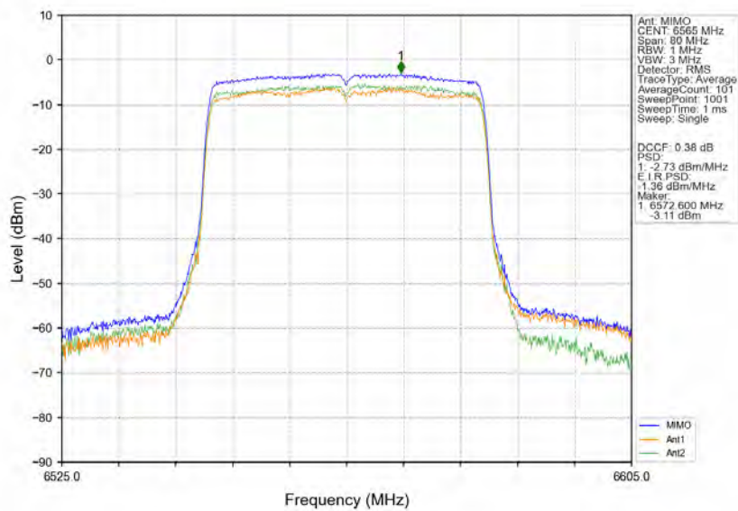
802.11ax(HEW40) LCH_6565MHz RU484 Left MIMO NTN
