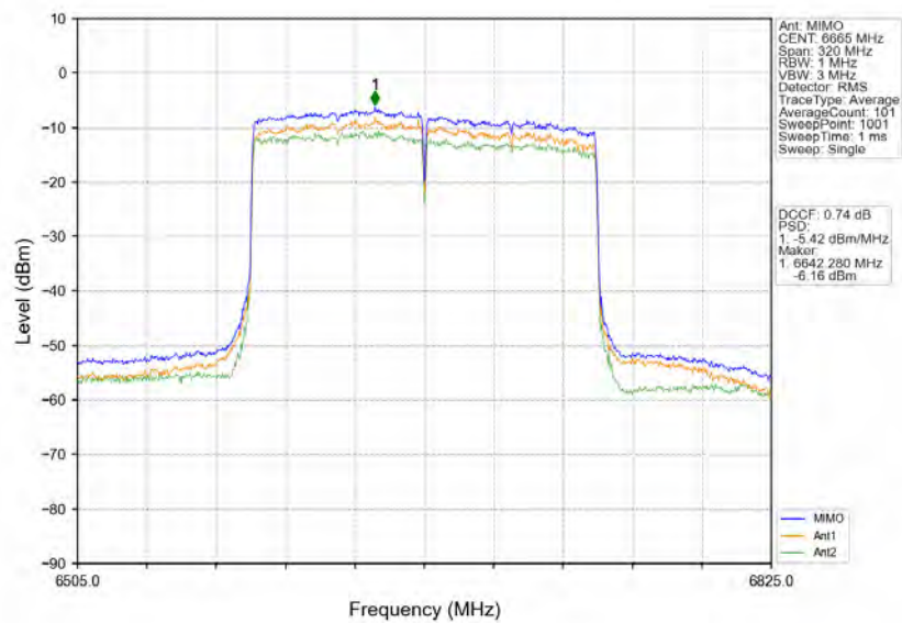
802.11ax(HEW160) MCH_6665MHz_2xRU996_Left_MIMO_NTNV
