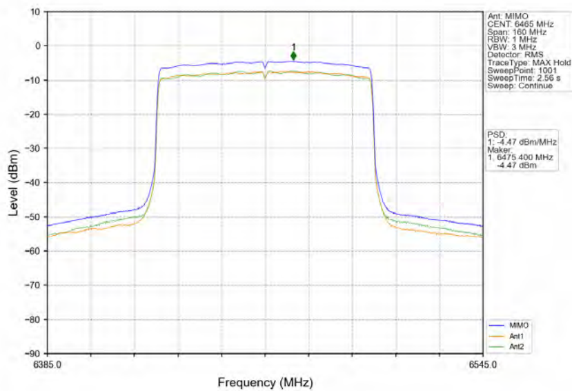
802.11ax(HEW80) LCH_6465MHz RU996 Left MIMO NTN
