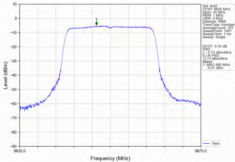
802.11ax(HEW20)_HCH_6855MHz_RU242_Left_Ant2_NTNV
