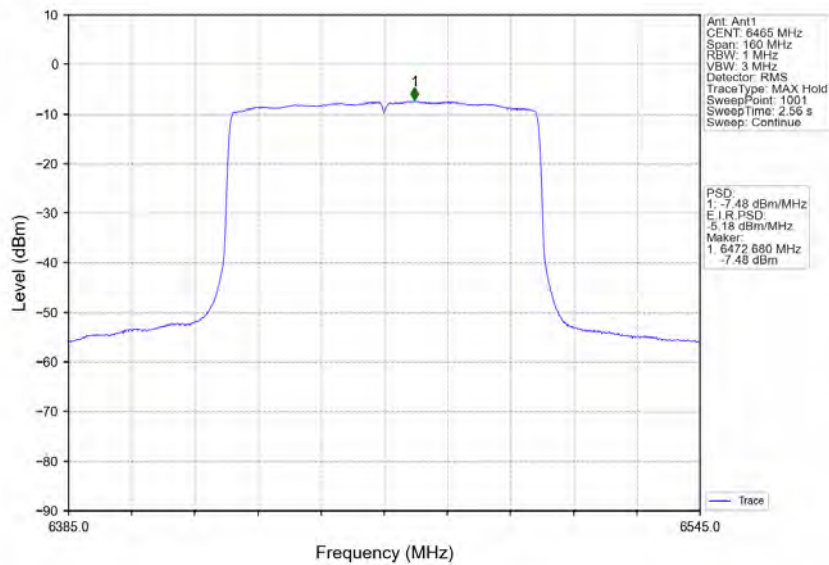
802.11ax(HEW80) LCH 6465MHz RU996 Left Ant1 NTN
