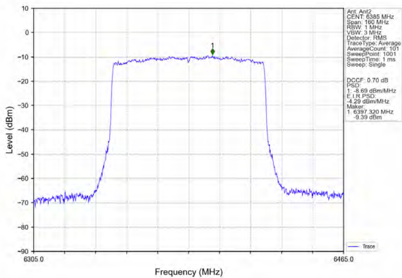
802.11ax(HEW80) HCH 6385MHz RU996 Left Ant2 NTVN
