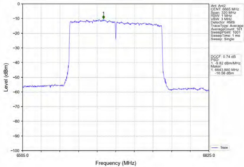
802.11ax(HEW160) MCH_6665MHz_2xRU996_Left_MIMO_NTNV
