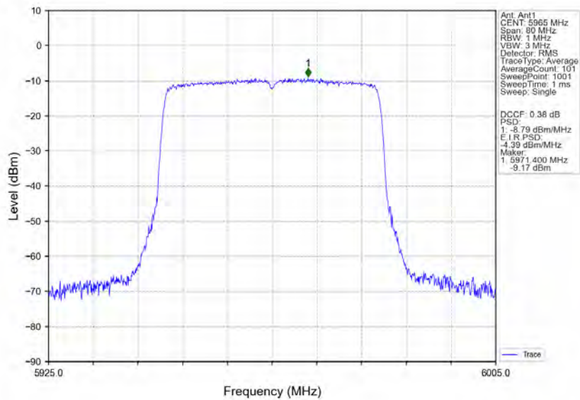
802.11ax(HEW40)_LCH_5965MHz_RU484_Left_Ant1_NTNV
