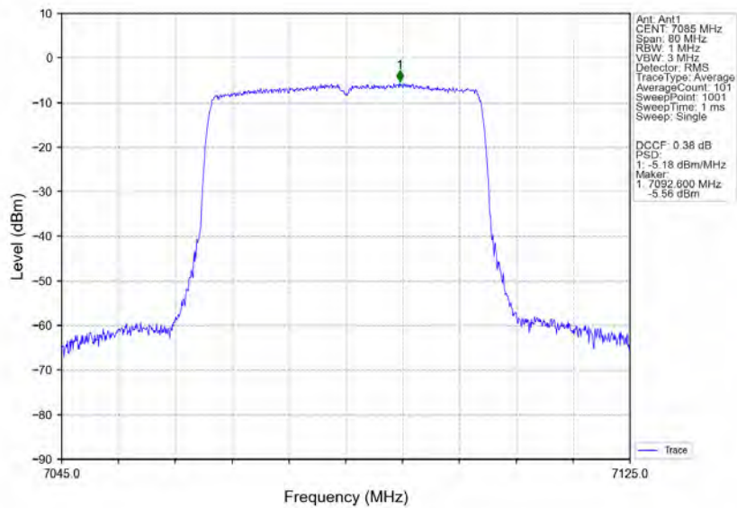
802.11ax(HEW40)_HCH_7085MHz_RU484_Left_Ant1_NTNV
