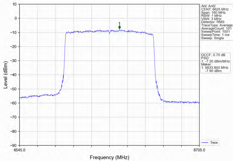
802.11ax(HEW80)_LCH_6625MHz_RU996_Left_Ant2_NTNV
