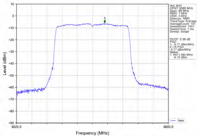
802.11ax(HEW40)_LCH_6565MHz_RU484_Left_Ant1_NTNV
