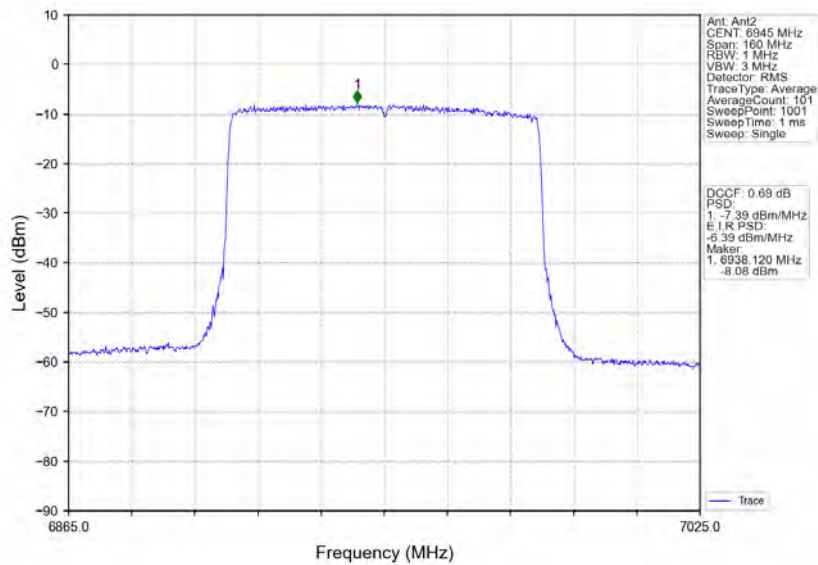
802.11ax(HEW80)_LCH_6945MHz_RU996_Left_Ant2_NTNV
