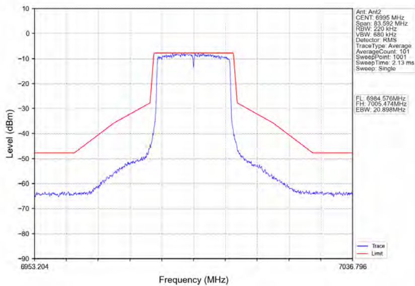
802.11ax(HEW20) MCH 6995MHz RU242 Left Ant2 NTVN
