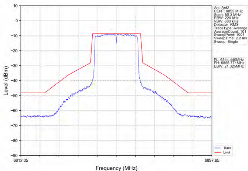
802.11ax(HEW20)_HCH_6855MHz_RU242_Left_Ant2_NTNV
