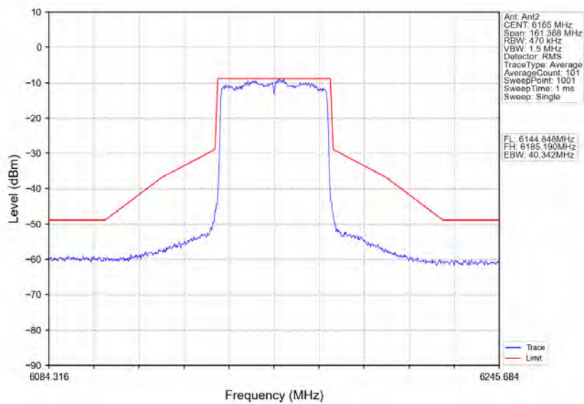
802.11ax(HEW40) MCH 6165MHz RU484 Left Ant2 NTVN
