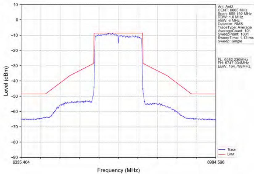
802.11ax(HEW160) MCH_6665MHz_2xRU996_Left_Ant2_NTNV
