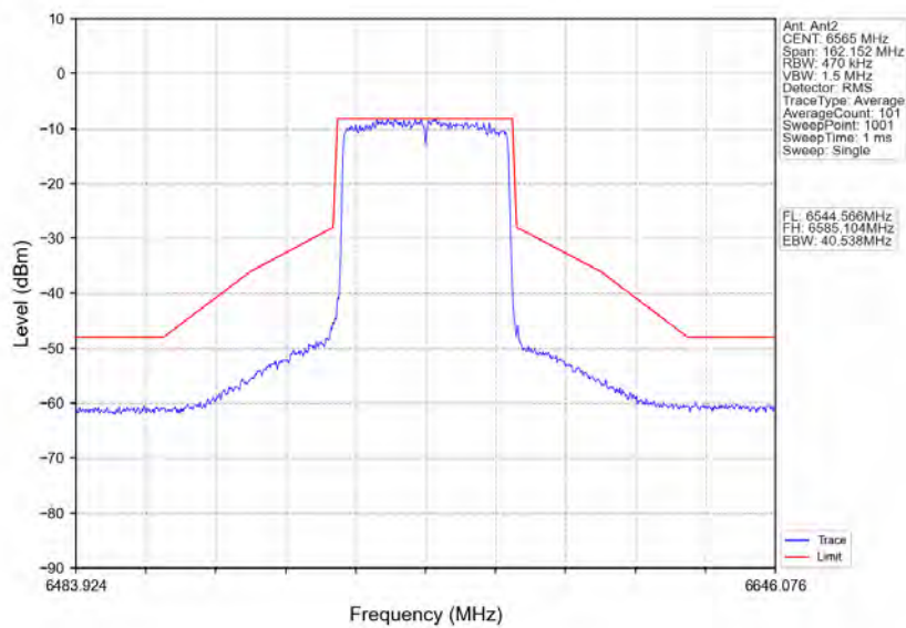
802.11ax(HEW40)_LCH_6565MHz_RU484_Left_Ant2_NTNV
