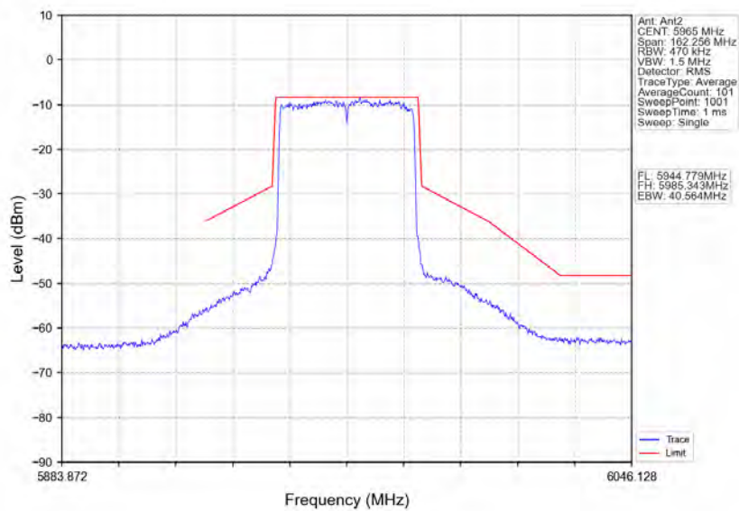
802.11ax(HEW40)_LCH_5965MHz_RU484_Left_Ant2_NTNV
