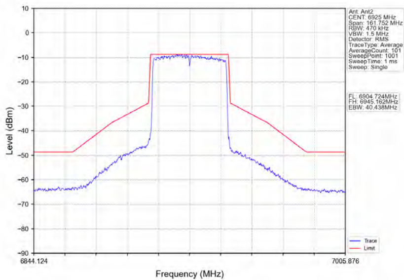
802.11ax(HEW40)_LCH_6925MHz_RU484_Left_Ant2_NTNV
