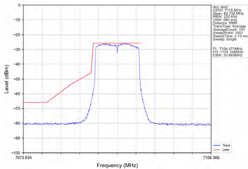
802.11ax(HEW20) HCH 7115MHz RU242 Left Ant2 NTVN
