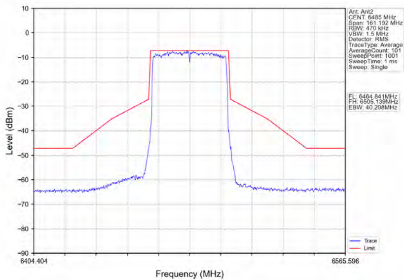
802.11ax(HEW40) MCH 6485MHz RU484 Left Ant2 NTVN
