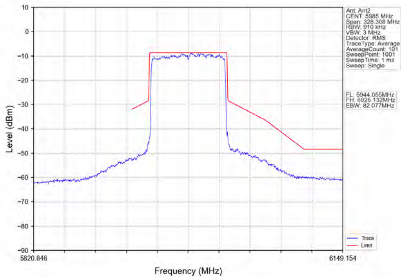
802.11ax(HEW80)_LCH_5985MHz_RU996_Left_Ant2_NTNV
