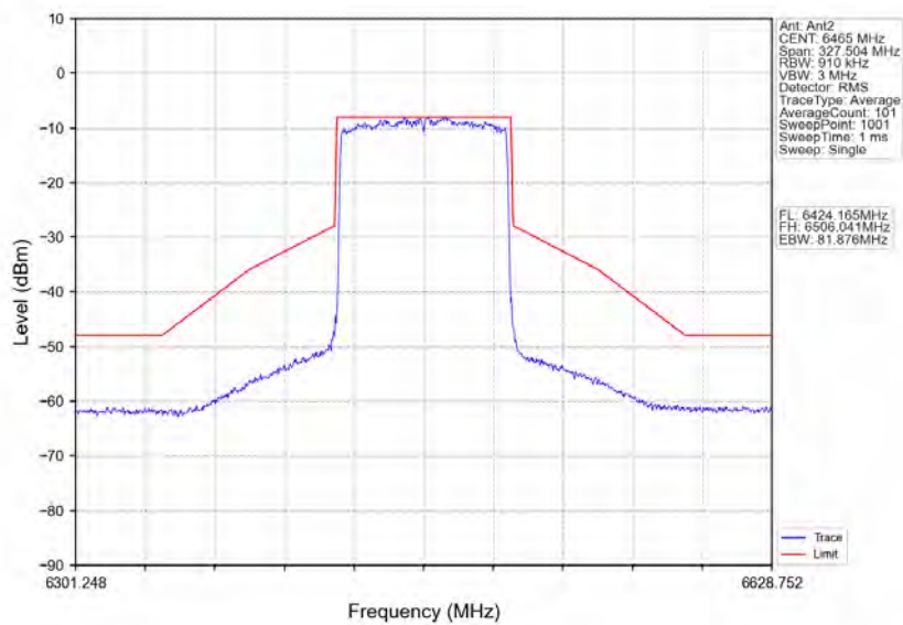
802.11ax(HEW80)_LCH_6465MHz_RU996_Left_Ant2_NTNV
