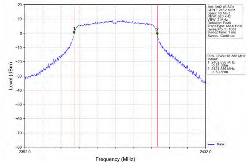
802.11n(HT20)_LCH_2412MHz_Ant2 (SISO)_NTNV
