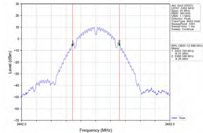
802.11b_HCH_2462MHz_Ant2 (SISO)_NTNV
