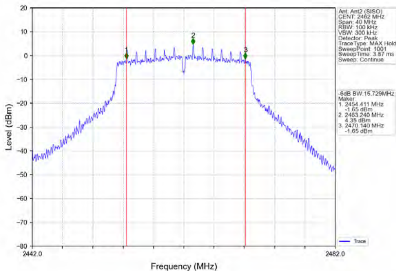
802.11n(HT20)_HCH_2462MHz_Ant2 (SISO)_NTNV
