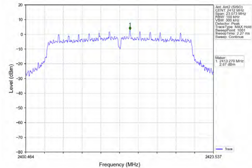
802.11n(HT20)_LCH_2412MHz_Ant2 (SISO)_NTNV
