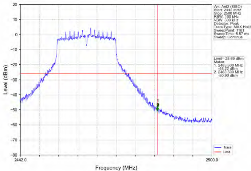
802.11n(HT20)_HCH_2462MHz_Ant2 (SISO)_NTNV
