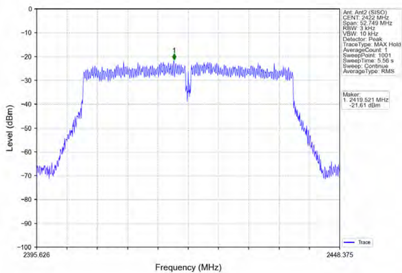
802.11n(HT40)_LCH_2422MHz_Ant2 (SISO)_NTNV
