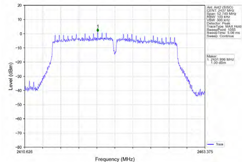
802.11n(HT40)_MCH_2437MHz_Ant2 (SISO)_NTNV
