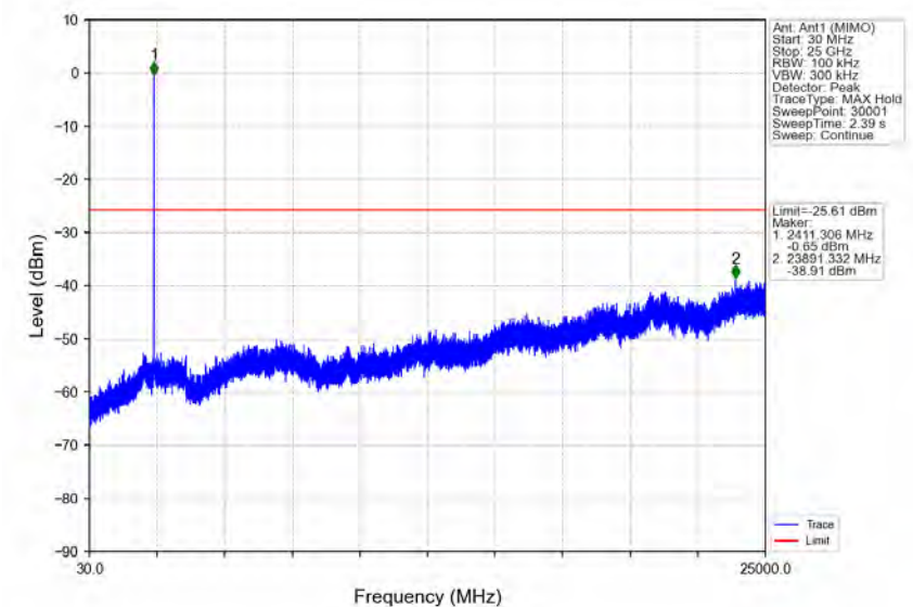
802.11n(HT20)_LCH_2412MHz_Ant1 (MIMO)_NTNV
