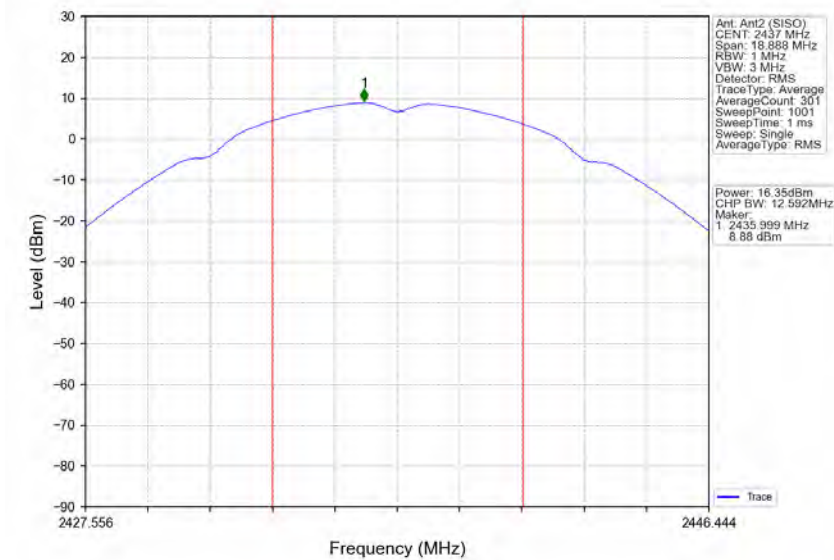
802.11b_MCH_2437MHz_Ant2 (SISO)_NTNV
