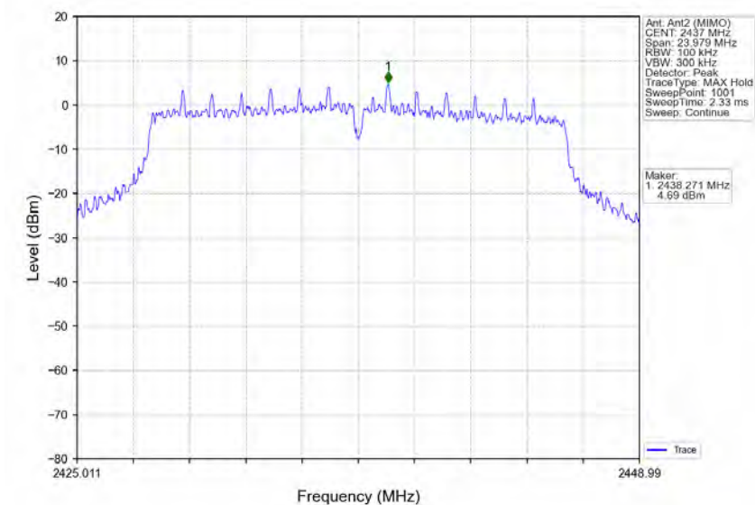
802.11n(HT20)_MCH_2437MHz_Ant2 (MIMO)_NTNV
