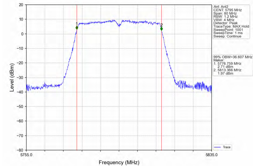
802.11n(HT40)_HCH_5795MHz_Ant2_NTNV
