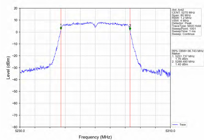
802.11n(HT40)_LCH_5270MHz_Ant2_NTNV
