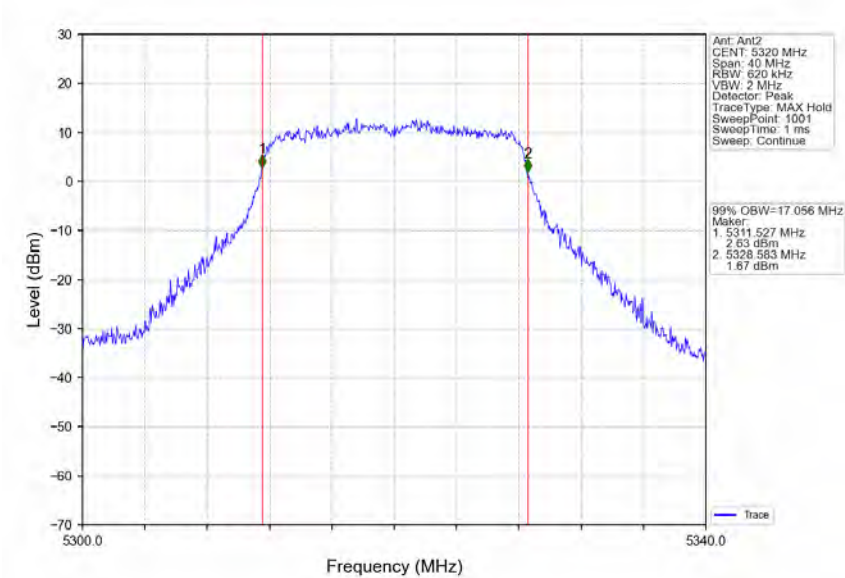
802.11a_HCH_5320MHz_Ant2_NTNV
