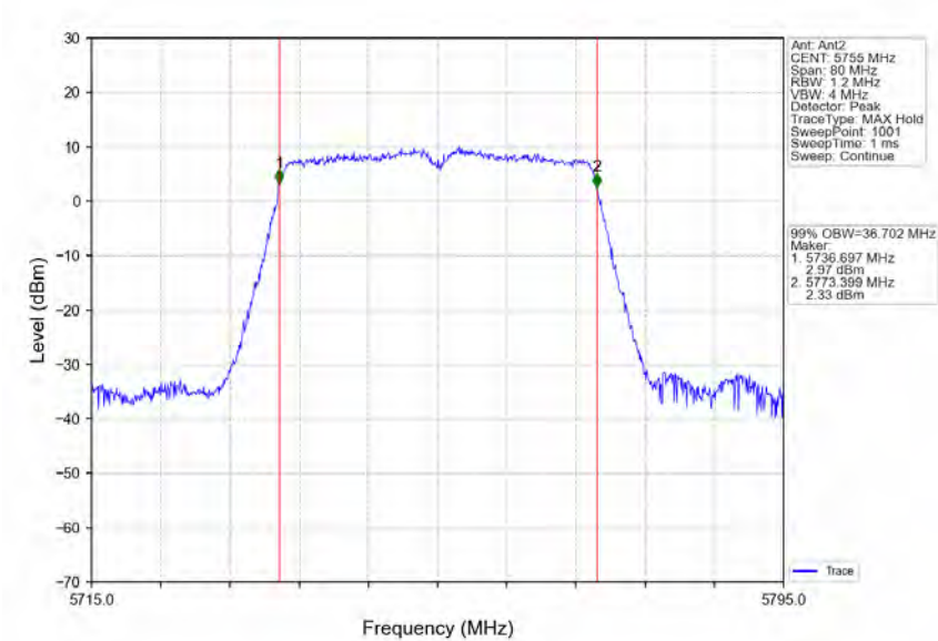
802.11n(HT40)_LCH_5755MHz_Ant2_NTNV
