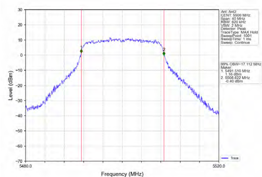
802.11a_LCH_5500MHz_Ant2_NTNV
