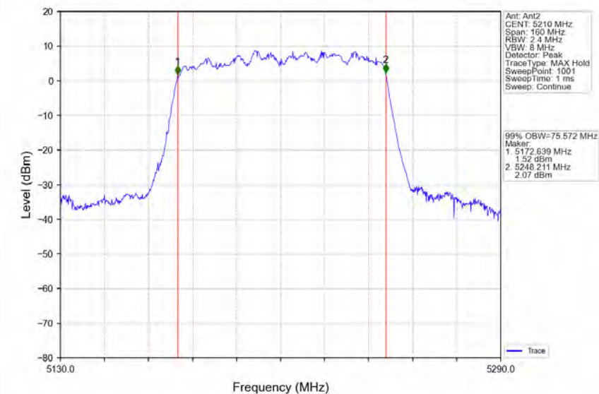
802.11ac(VHT80)_MCH_5210MHz_Ant2_NTNV
