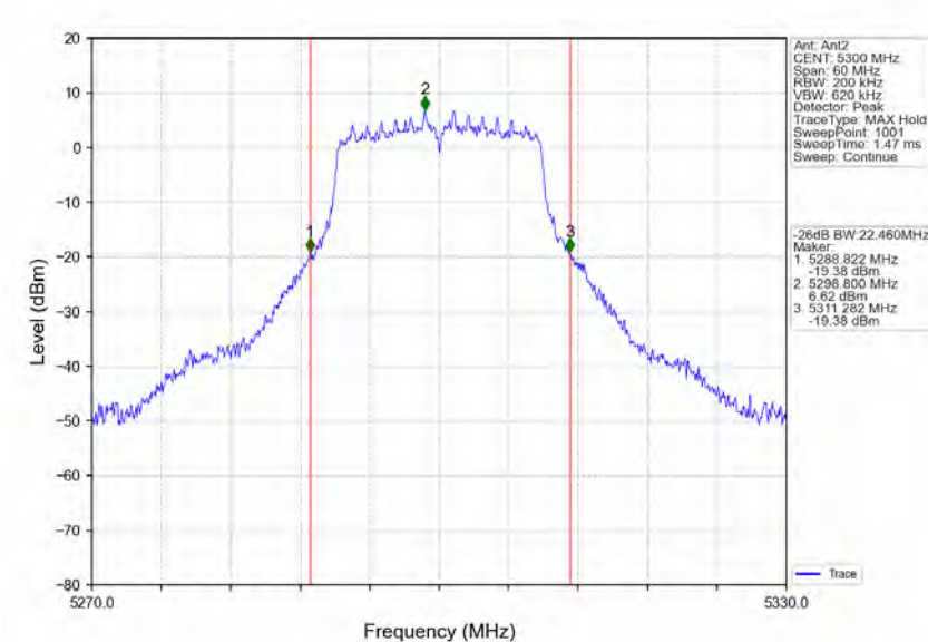
802.11n(HT20)_MCH_5300MHz_Ant2_NTNV
