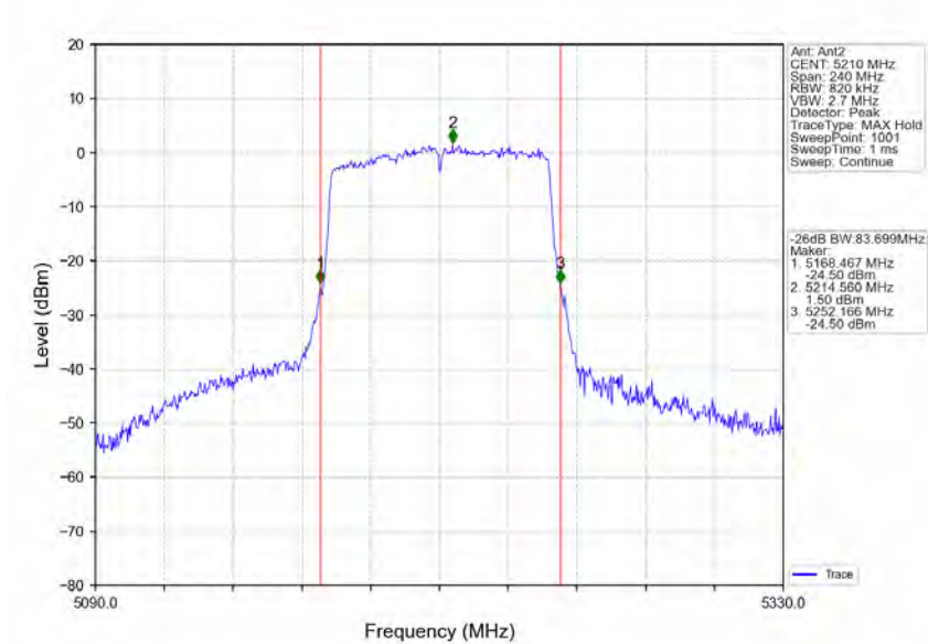
802.11ac(VHT80)_MCH_5210MHz_Ant2_NTNV
