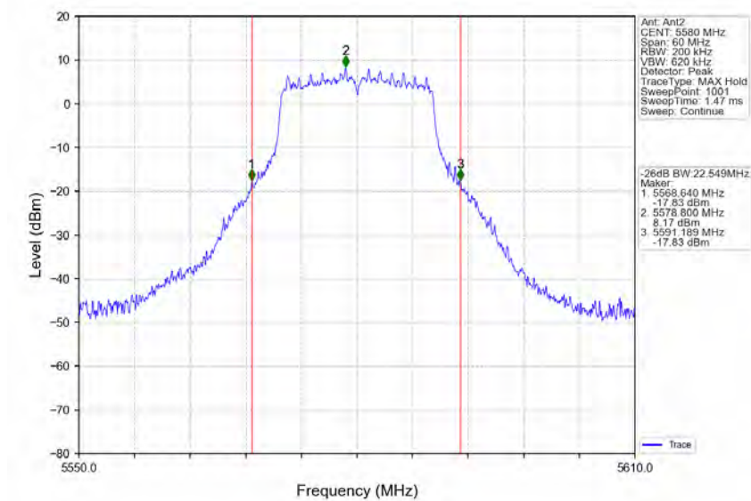
802.11a_MCH_5580MHz_Ant2_NTNV
