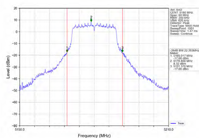
802.11n(HT20)_LCH_5180MHz_Ant2_NTNV
