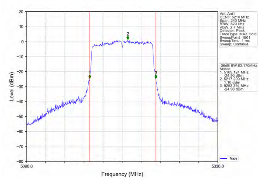
802.11ac(VHT80)_MCH_5210MHz_Ant1_NTNV
