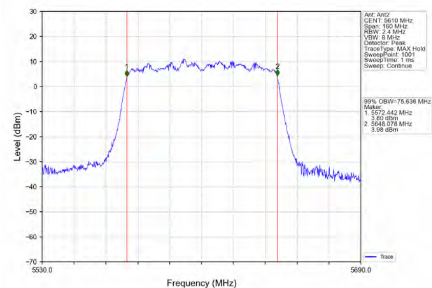
802.11ac(VHT80)_HCH_5610MHz_Ant2_NTNV
