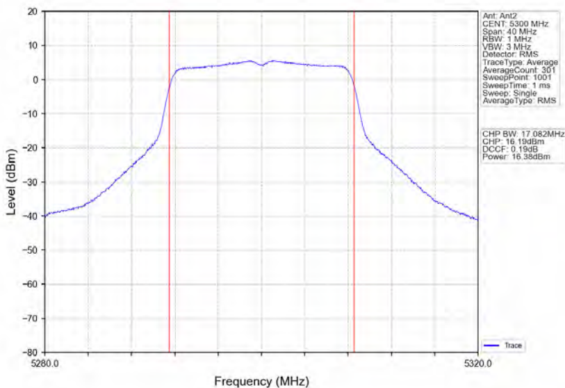
802.11a_MCH_5300MHz_Ant2_NTNV
