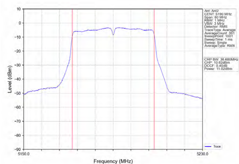
802.11n(HT40)_LCH_5190MHz_Ant2_NTNV
