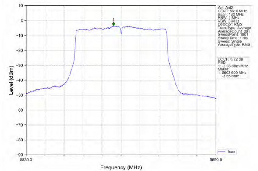
802.11ac(VHT80)_HCH_5610MHz_Ant2_NTNV
