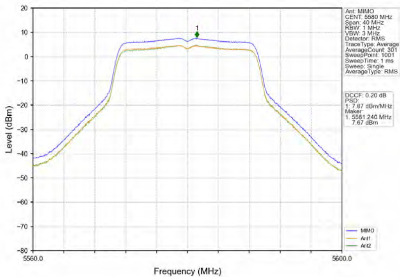
802.11n(HT20)_MCH_5580MHz_MIMO_NTNV
