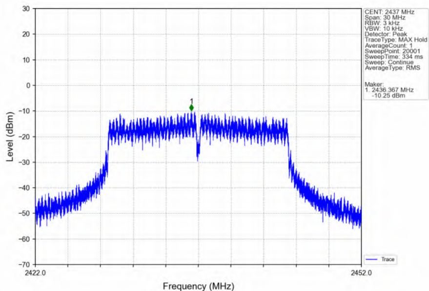
802.11g_MCH_2437MHz_Ant3 (SISO)_NTNV
