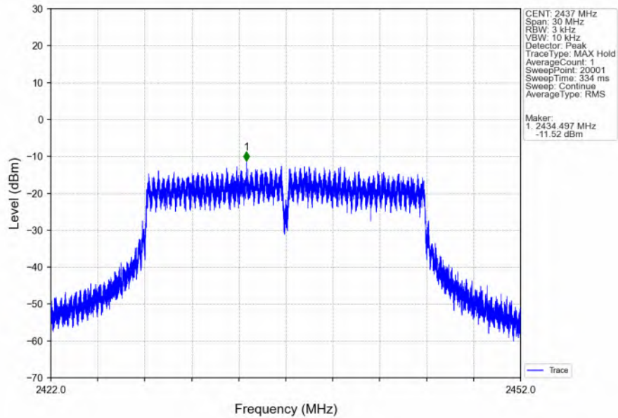
802.11n(HT20)_MCH_2437MHz_MIMO_NTNV
