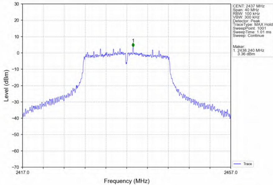
802.11g_MCH_2437MHz_Ant3 (SISO)_NTNV
