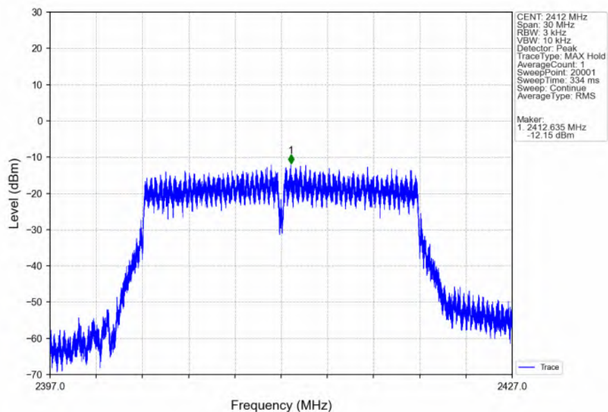
802.11n(HT20)_LCH_2412MHz_Ant3 (MIMO)_NTNV
