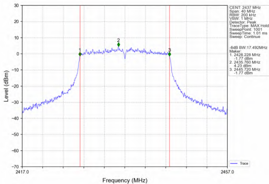
802.11n(HT20)_MCH_2437MHz_Ant2 (MIMO)_NTNV
