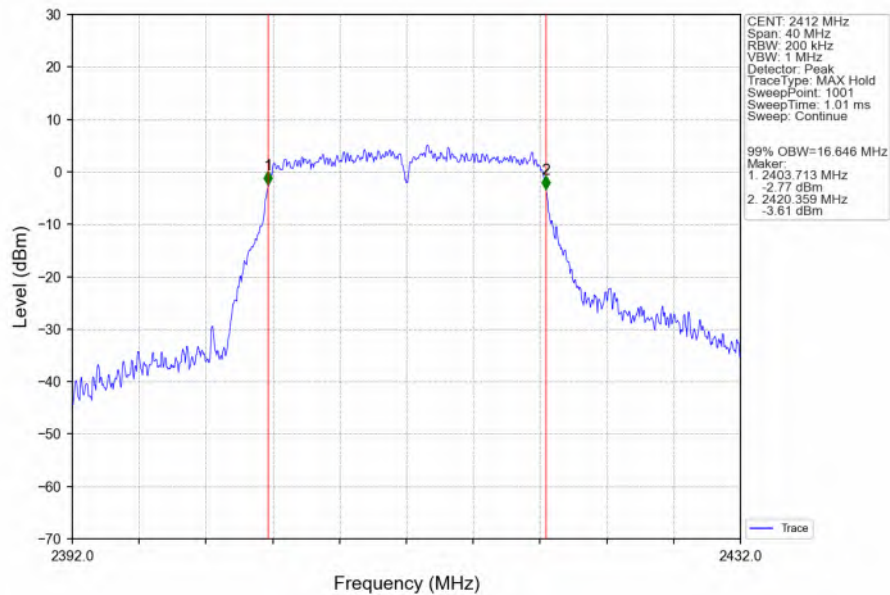
802.11g_LCH_2412MHz_Ant2 (SISO)_NTNV
