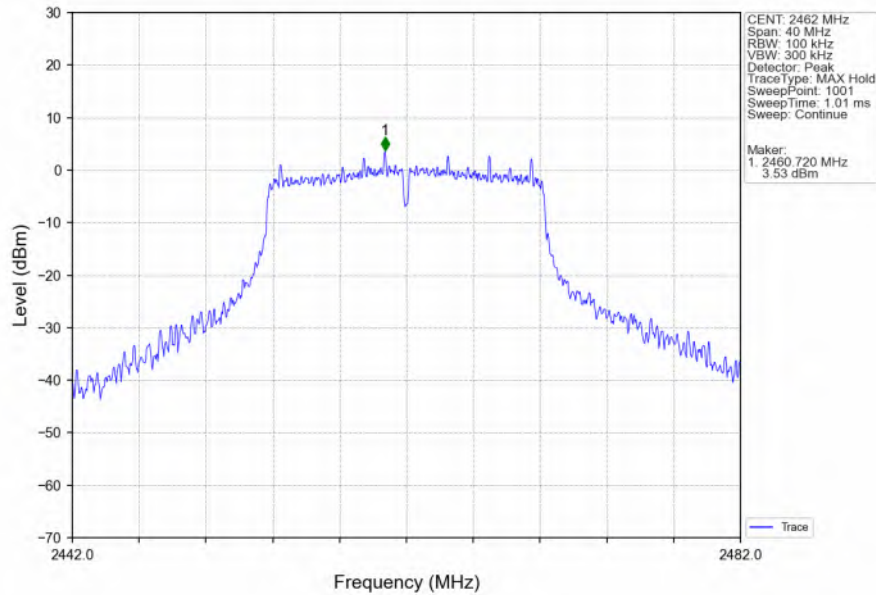
802.11g_HCH_2462MHz_Ant3 (SISO)_NTNV
