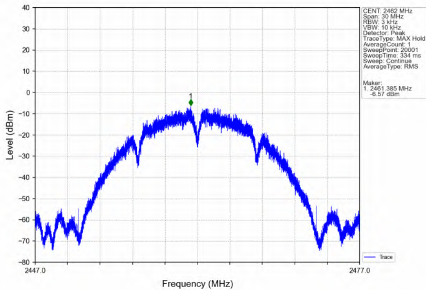
802.11b_HCH_2462MHz_Ant3 (SISO)_NTNV
