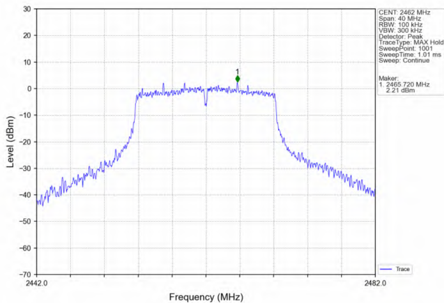
802.11g_HCH_2462MHz_Ant3 (SISO)_NTNV
