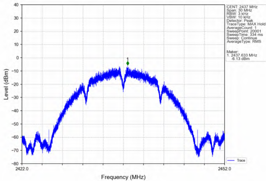
802.11b_MCH_2437MHz_Ant3 (SISO)_NTNV
