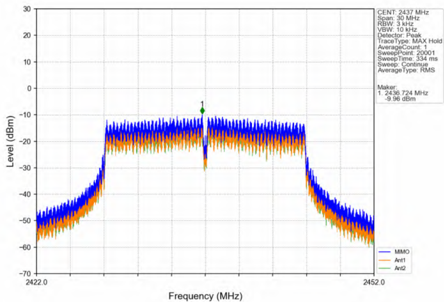
802.11n(HT20)_MCH_2437MHz_MIMO_NTNV
