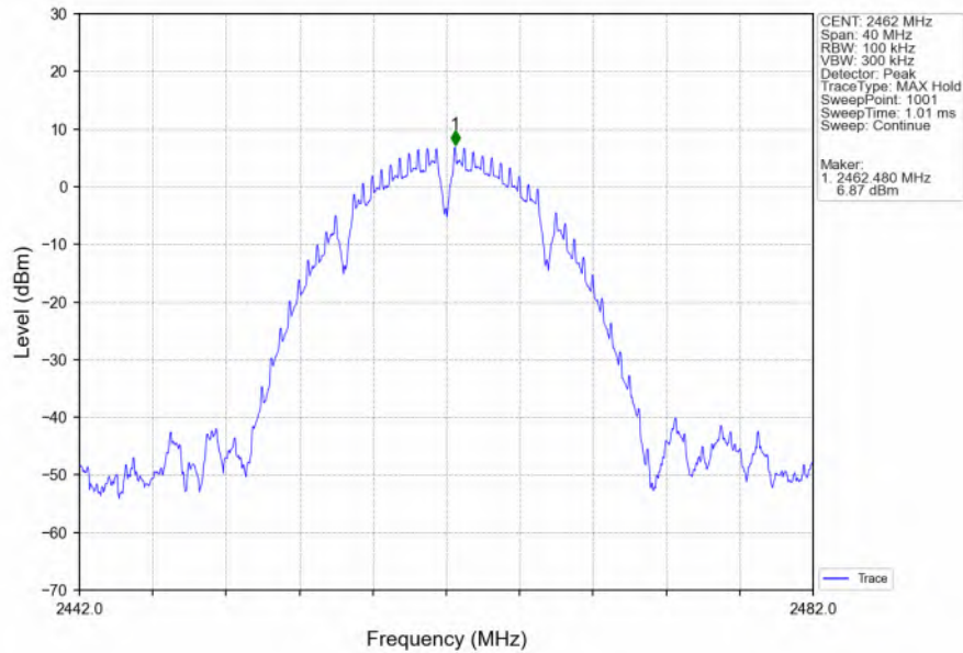
802.11b_HCH_2462MHz_Ant3 (SISO)_NTNV
