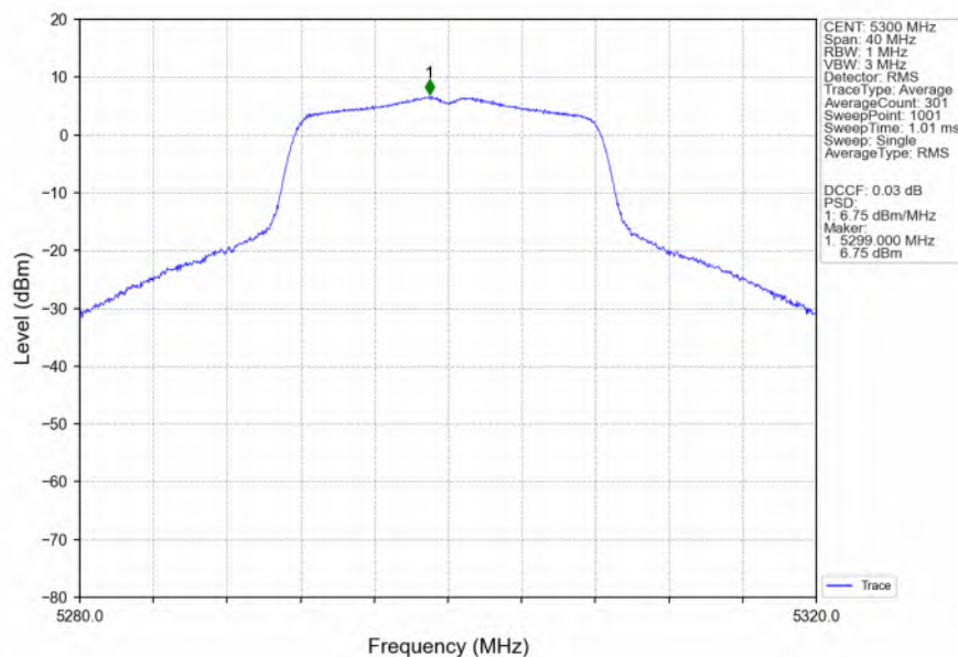
802.11a_MCH_5300MHz_Ant3_NTNV
