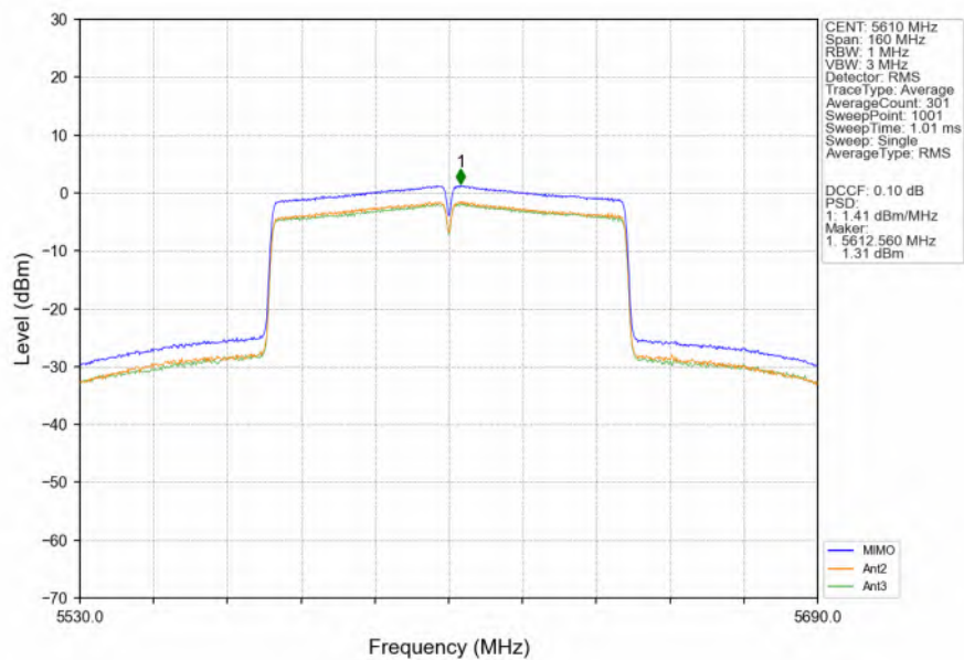
802.11ac(VHT80)_HCH_5610MHz_MIMO_NTNV
