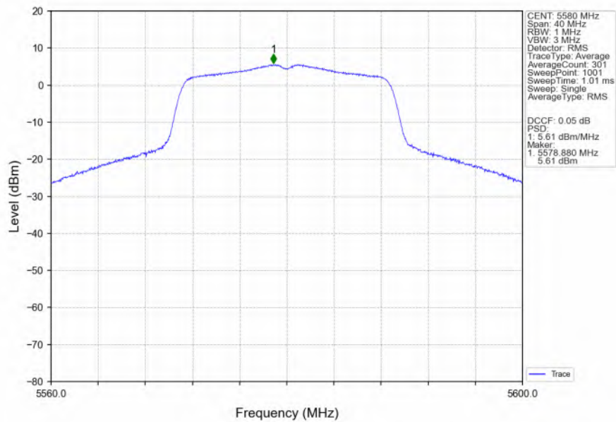
802.11n(HT20)_MCH_5580MHz_MIMO_NTNV
