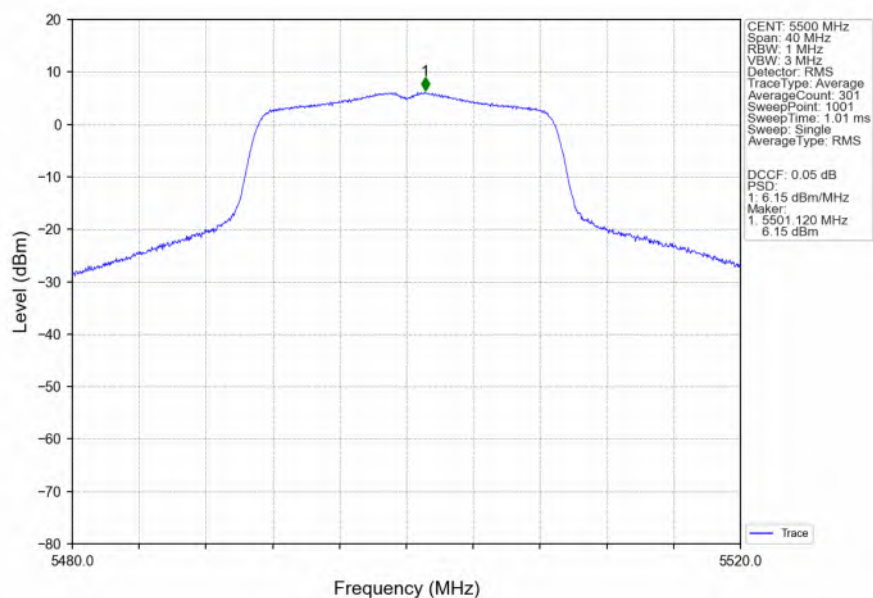
802.11n(HT20)_LCH_5500MHz_Ant3_NTNV
