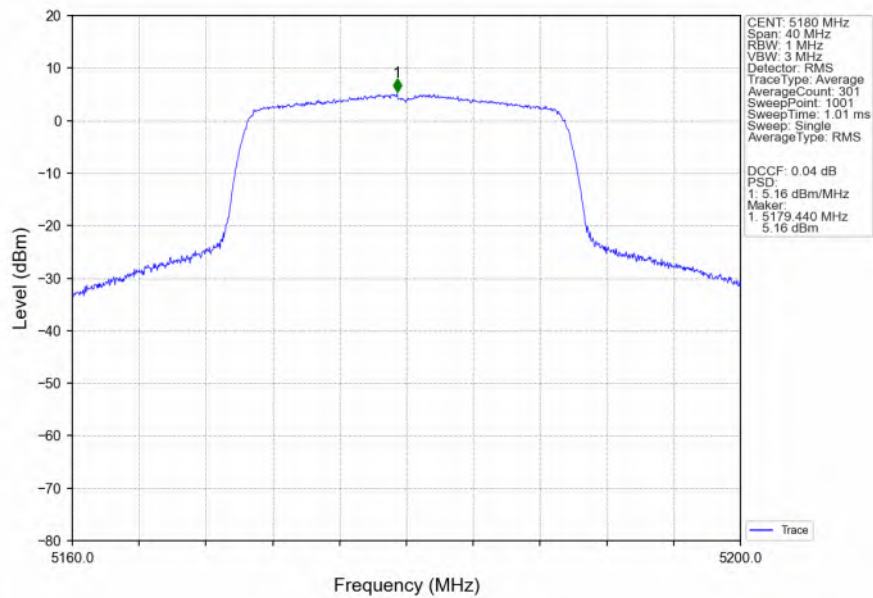
802.11ax(HEW20) LCH 5180MHz SU / Ant3 NTN
