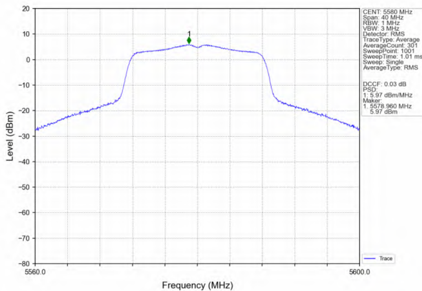
802.11a_MCH_5580MHz_Ant3_NTNV
