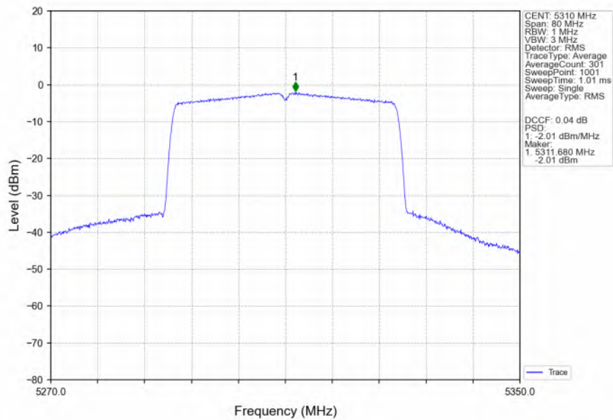
802.11ax(HEW40) HCH 5310MHz SU / Ant3 NTN
