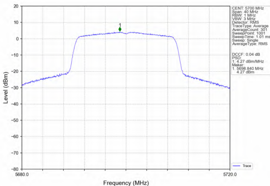
802.11ax(HEW20) HCH 5700MHz SU / Ant3 NTN
