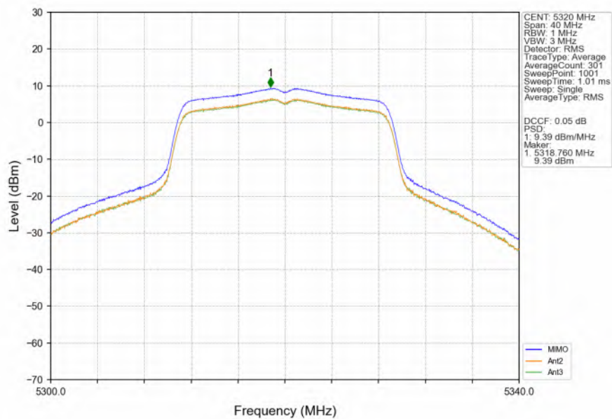
802.11n(HT20)_HCH_5320MHz_MIMO_NTNV
