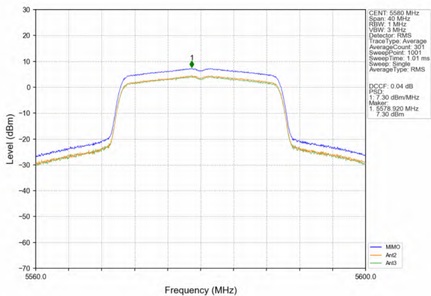
802.11ax(HEW20) MCH 5580MHz SU / MIMO NTN
