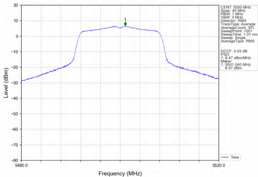
802.11a_LCH_5500MHz_Ant3_NTNV
