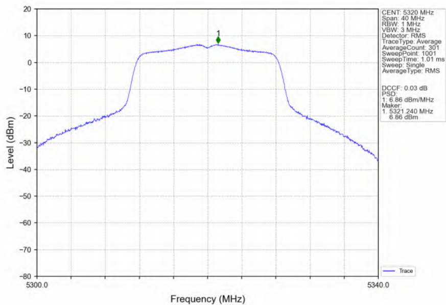
802.11a_HCH_5320MHz_Ant3_NTNV
