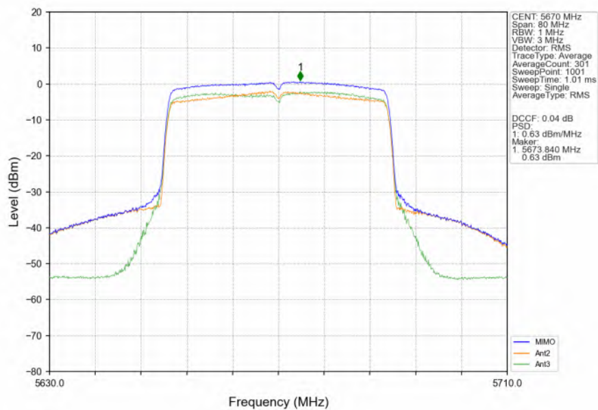
802.11ax(HEW40) HCH 5670MHz SU / MIMO NTN
