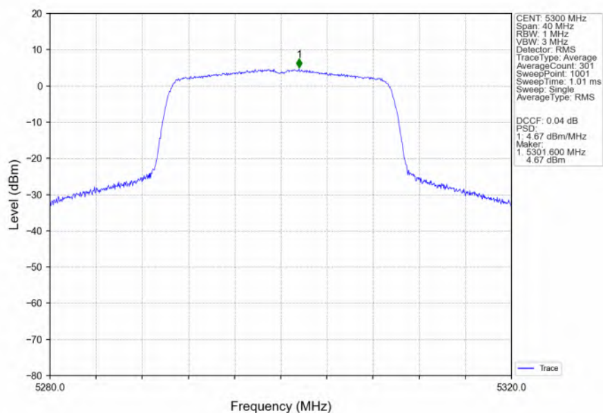
802.11ax(HEW20) MCH 5300MHz SU / Ant3 NTN
