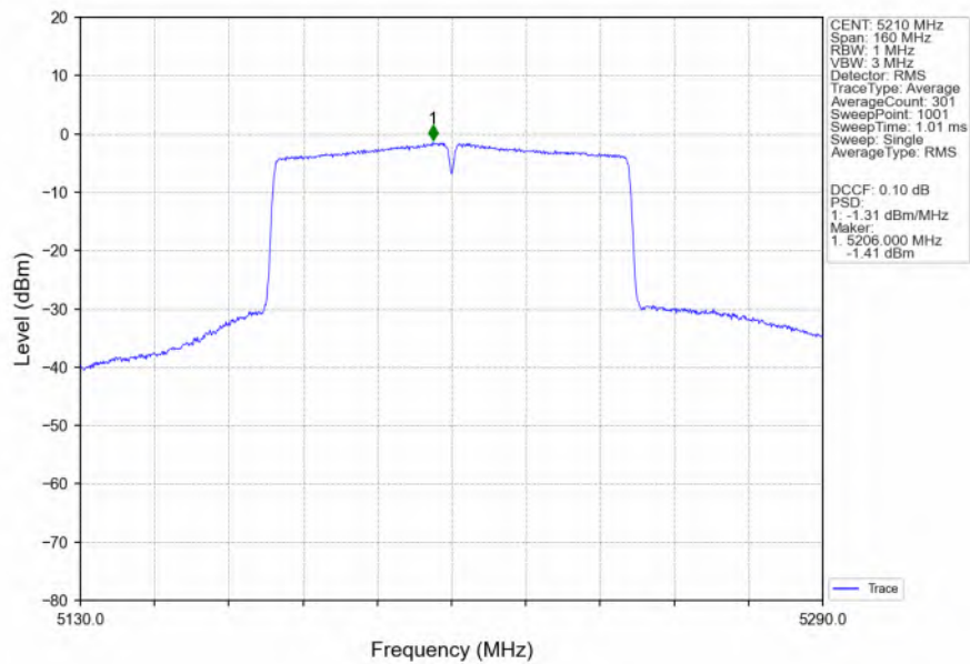
802.11ac(VHT80)_MCH_5210MHz_Ant3_NTNV
