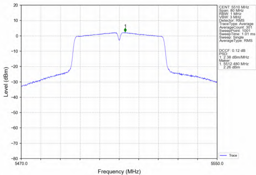
802.11n(HT40)_LCH_5510MHz_Ant2_NTNV
