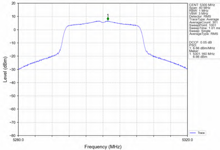
802.11n(HT20)_MCH_5300MHz_Ant3_NTNV
