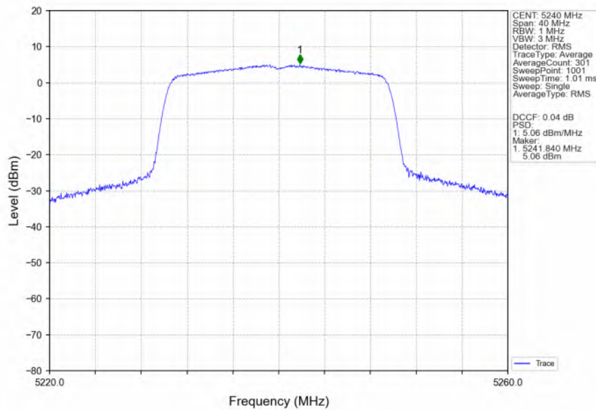
802.11ax(HEW20) HCH 5240MHz SU / Ant3 NTN
