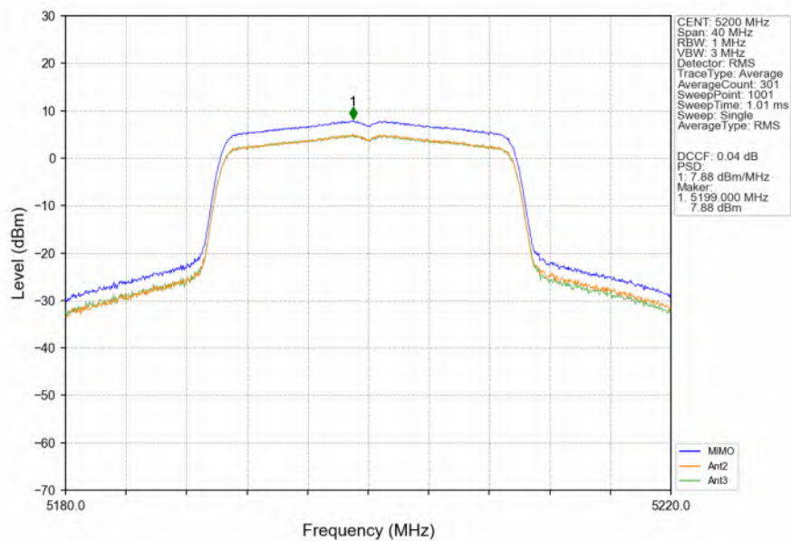
802.11ax(HEW20) MCH 5200MHz SU / MIMO NTN
