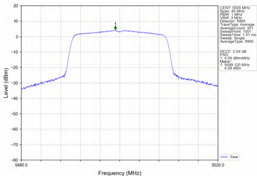
802.11ax(HEW20) LCH 5500MHz SU / Ant3 NTN
