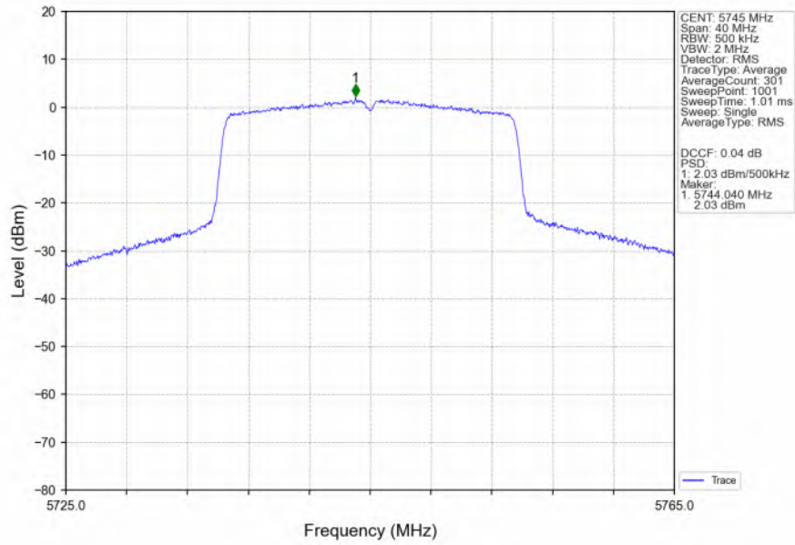
802.11ax(HEW20) LCH 5745MHz SU / Ant3 NTN
