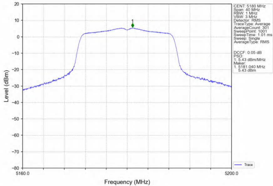
802.11n(HT20)_LCH_5180MHz_Ant3_NTNV
