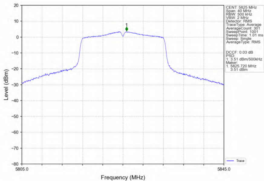
802.11a_HCH_5825MHz_Ant3_NTNV
