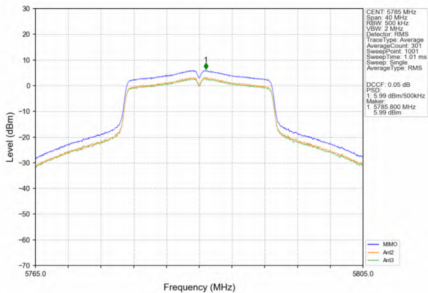
802.11n(HT20)_MCH_5785MHz_MIMO_NTNV
