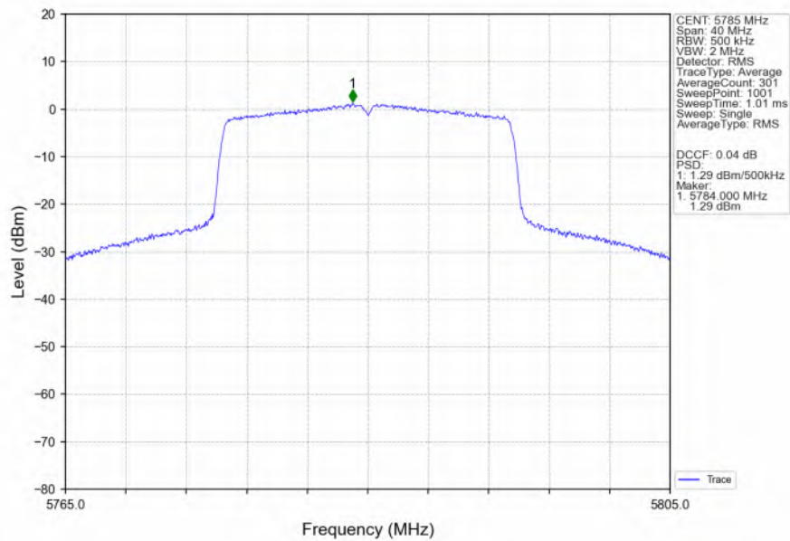
802.11ax(HEW20) MCH 5785MHz SU / MIMO NTN
