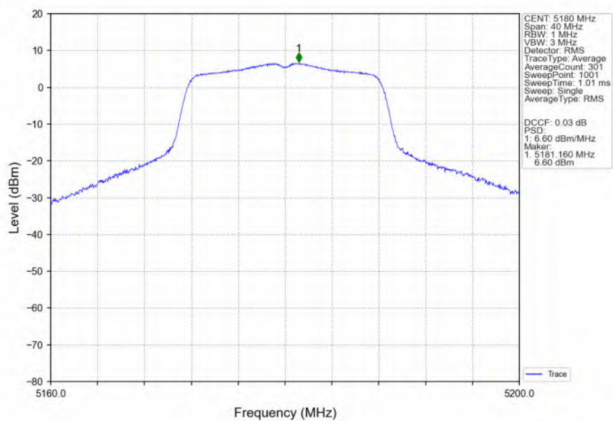
802.11a_LCH_5180MHz_Ant3_NTNV
