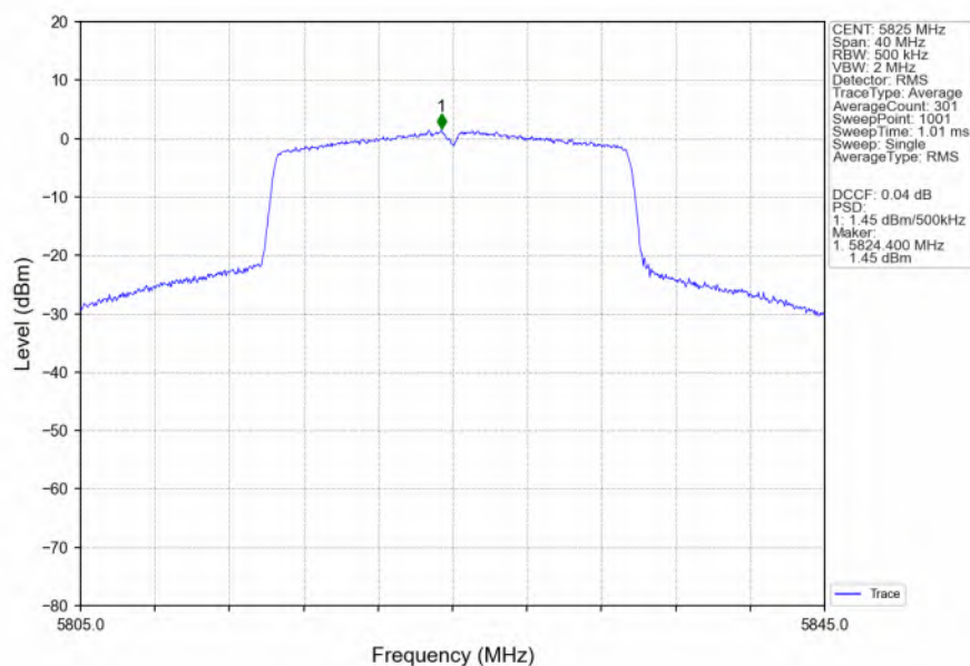
802.11ax(HEW20) HCH 5825MHz SU / Ant3 NTN
