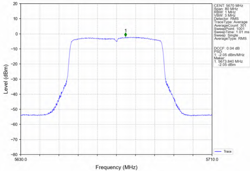
802.11ax(HEW40) HCH 5670MHz SU / MIMO NTN
