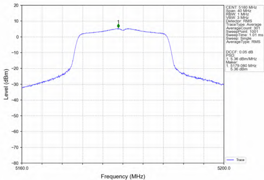
802.11n(HT20)_LCH_5180MHz_Ant3_NTNV
