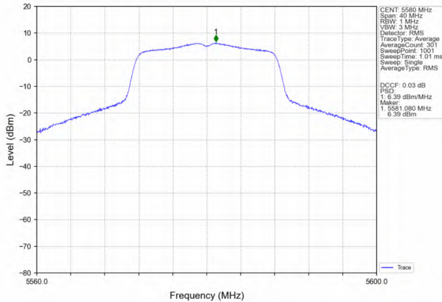
802.11a_MCH_5580MHz_Ant3_NTNV
