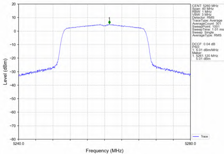
802.11ax(HEW20) LCH 5260MHz SU / MIMO NTN
