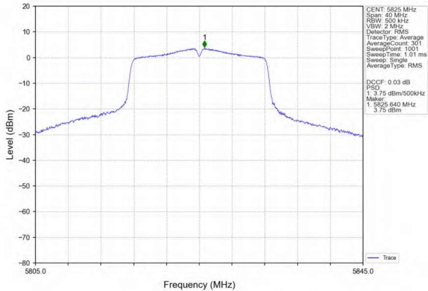
802.11a_HCH_5825MHz_Ant3_NTNV
