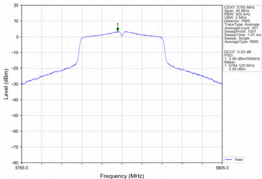
802.11a_MCH_5785MHz_Ant3_NTNV
