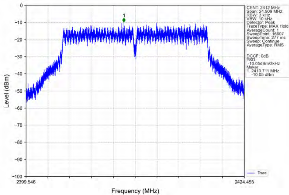
802.11n(HT20)_LCH_2412MHz_ANT3 (MIMO)_NTNV
