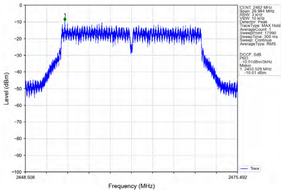
802.11n(HT20)_HCH_2462MHz_ANT3 (MIMO)_NTNV
