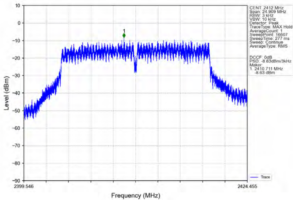
802.11n(HT20)_LCH_2412MHz_ANT3 (MIMO)_NTNV
