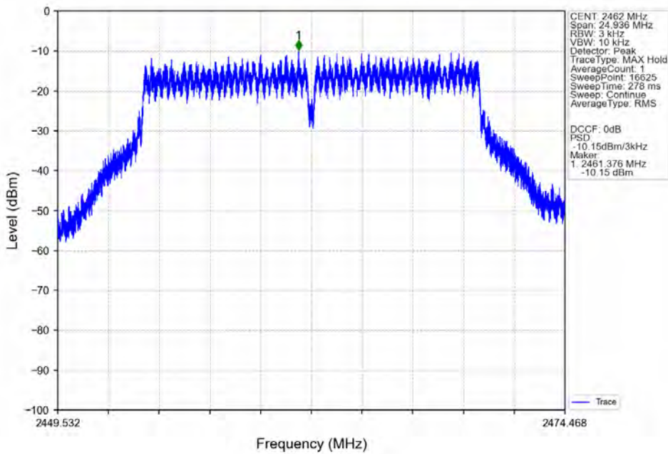
802.11g_HCH_2462MHz_ANT3 (SISO)_NTNV
