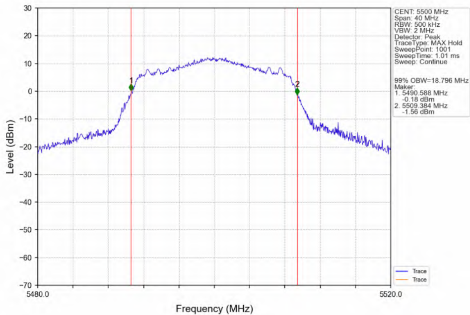
802.11n(HT20)_LCH_5500MHz_ANT3_NTNV
