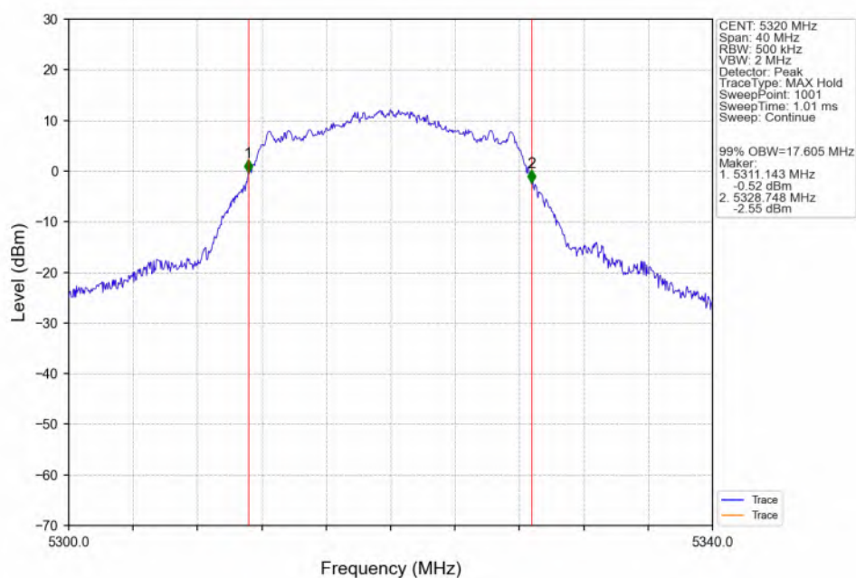
802.11a_HCH_5320MHz_ANT3_NTNV
