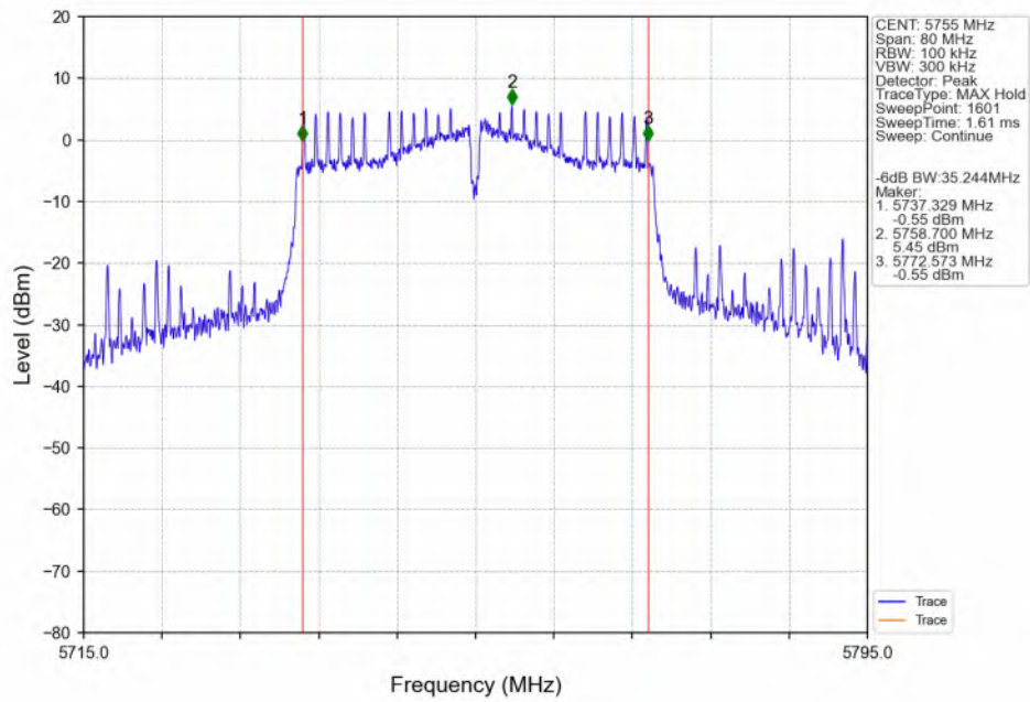
802.11n(HT40)_LCH_5755MHz_ANT3_NTNV
