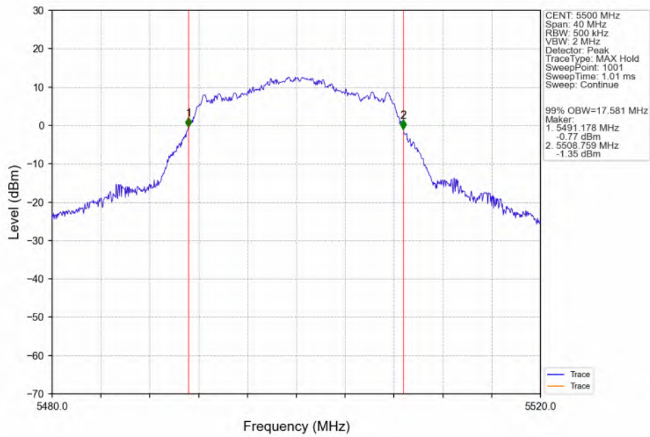
802.11a_LCH_5500MHz_ANT3_NTNV
