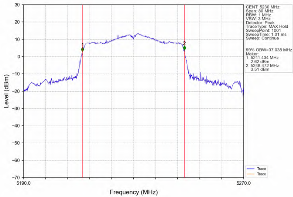
802.11n(HT40)_HCH_5230MHz_ANT3_NTNV
