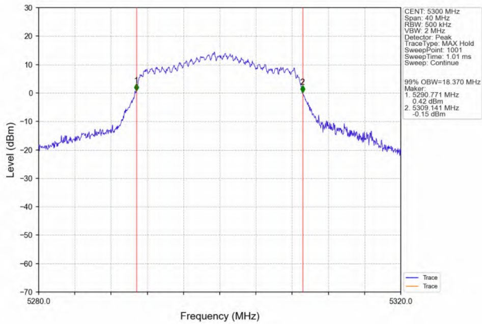
802.11n(HT20)_MCH_5300MHz_ANT3_NTNV
