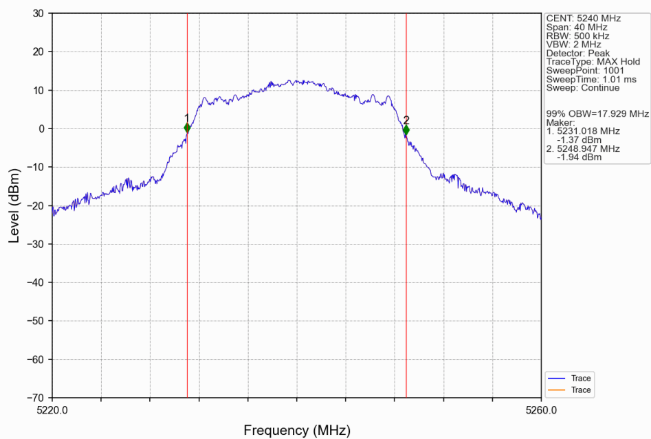
802.11a_HCH_5240MHz_ANT3_NTNV
