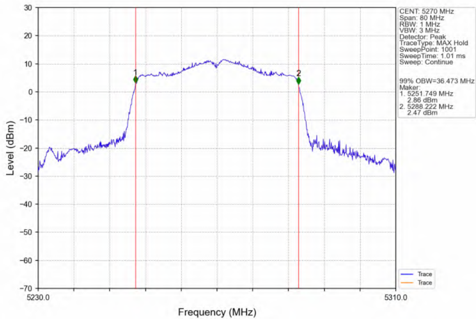
802.11ax(HEW40)_LCH_5270MHz_SU / _ANT3_NTNV
