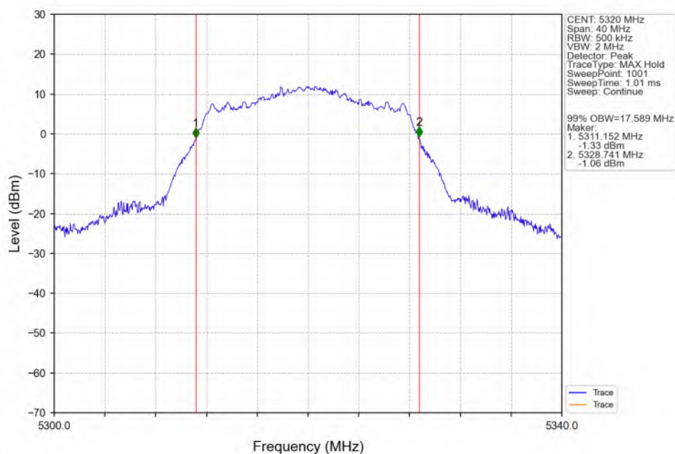
802.11a_HCH_5320MHz_ANT3_NTNV
