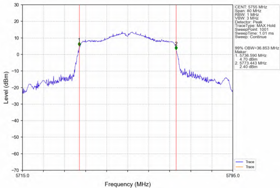
802.11n(HT40)_LCH_5755MHz_ANT3_NTNV
