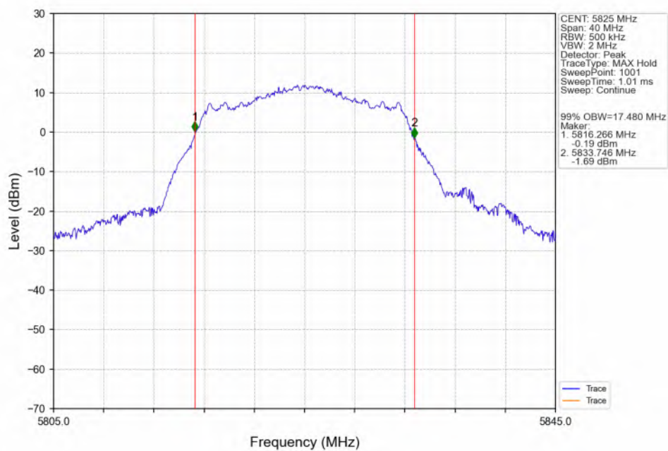
802.11a_HCH_5825MHz_ANT3_NTNV
