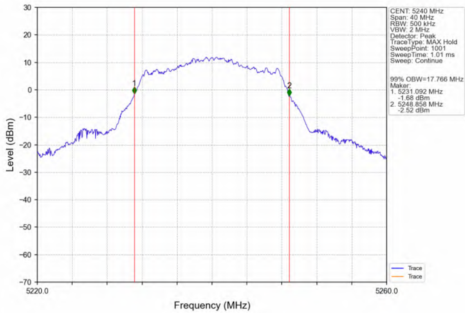
802.11a_HCH_5240MHz_ANT3_NTNV
