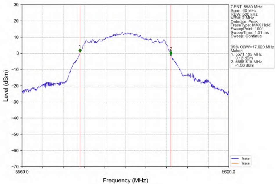
802.11a_MCH_5580MHz_ANT3_NTNV
