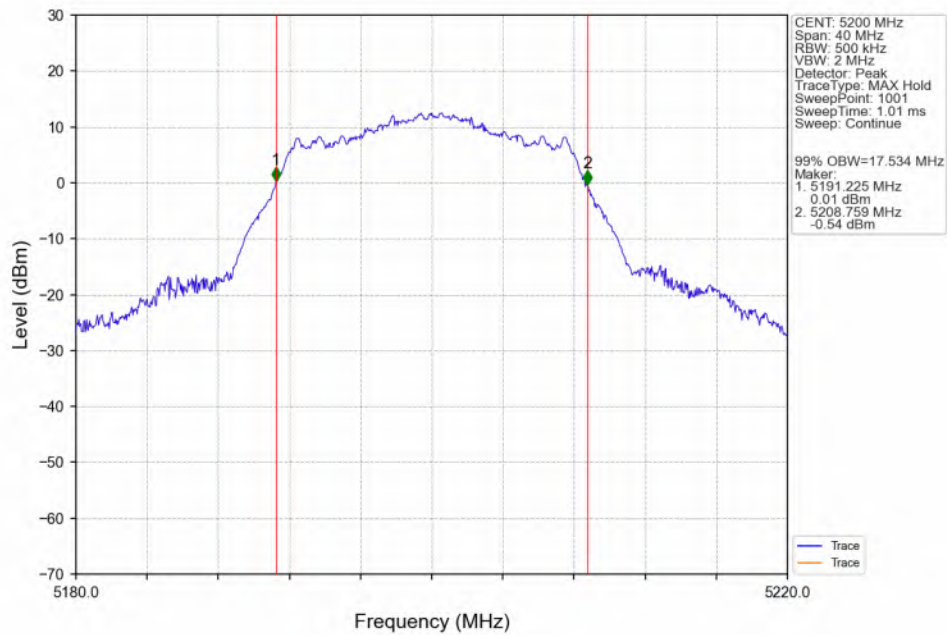
802.11a_MCH_5200MHz_ANT3_NTNV
