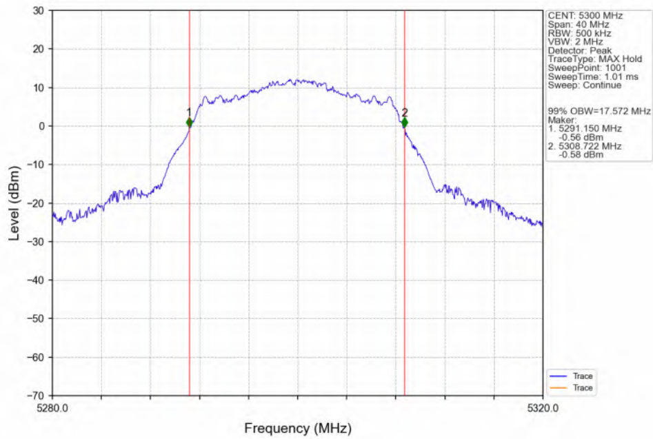
802.11a_MCH_5300MHz_ANT3_NTNV
