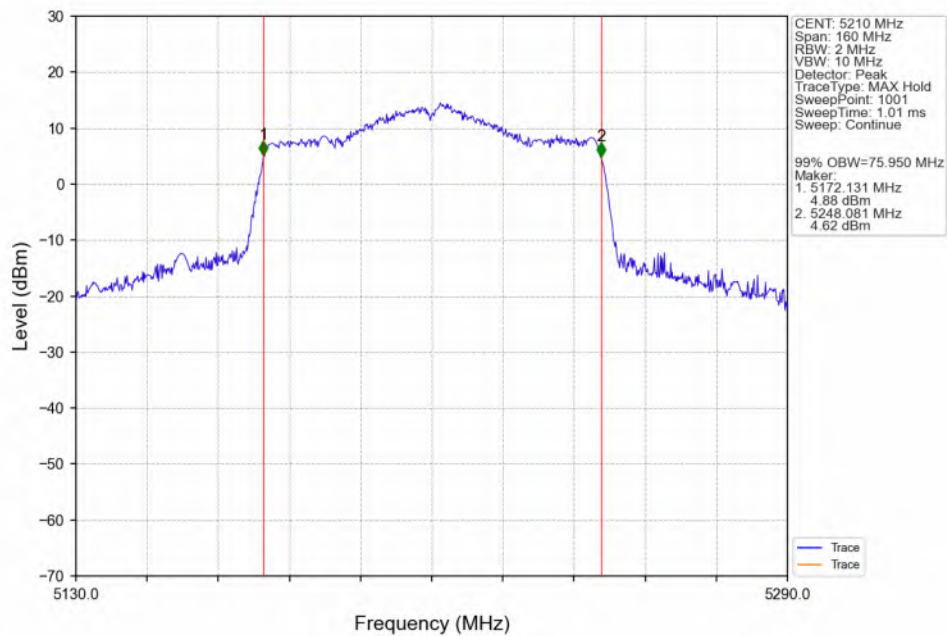
802.11ac(VHT80)_MCH_5210MHz_ANT3_NTNV
