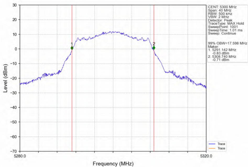
802.11a_MCH_5300MHz_ANT3_NTNV
