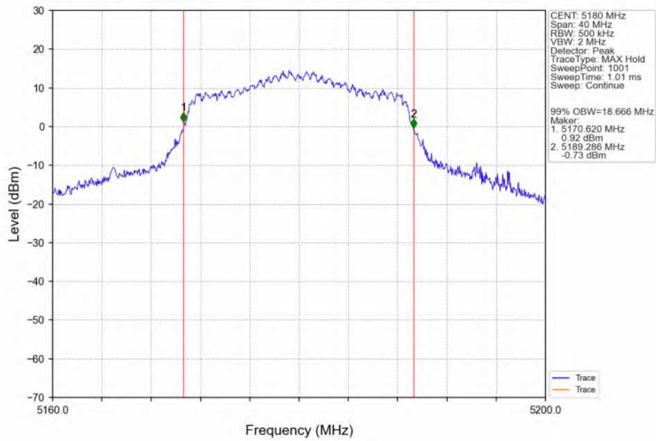
802.11n(HT20)_LCH_5180MHz_ANT3_NTNV
