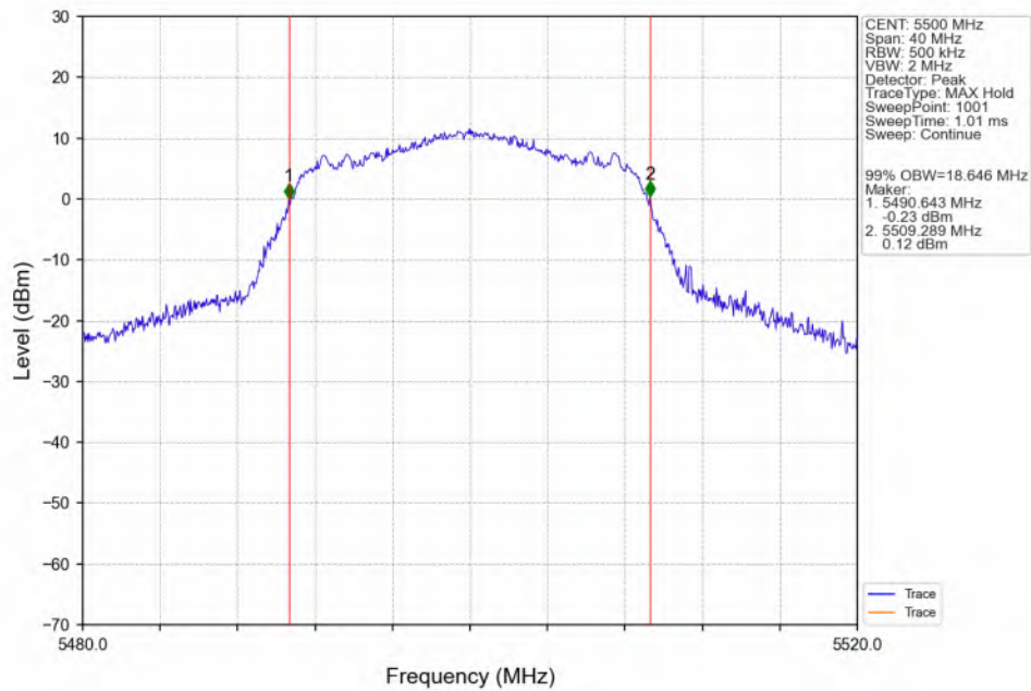
802.11ax(HEW20)_LCH_5500MHz_SU / _ANT3_NTNV
