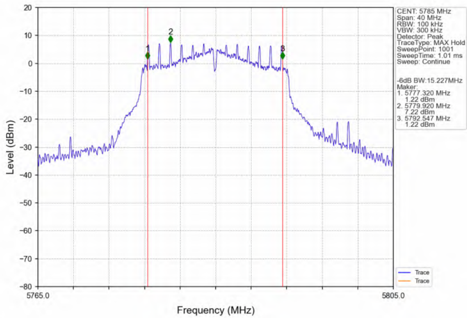
802.11a_MCH_5785MHz_ANT3_NTNV
