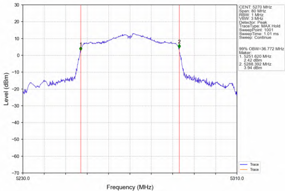
802.11n(HT40)_LCH_5270MHz_ANT3_NTNV
