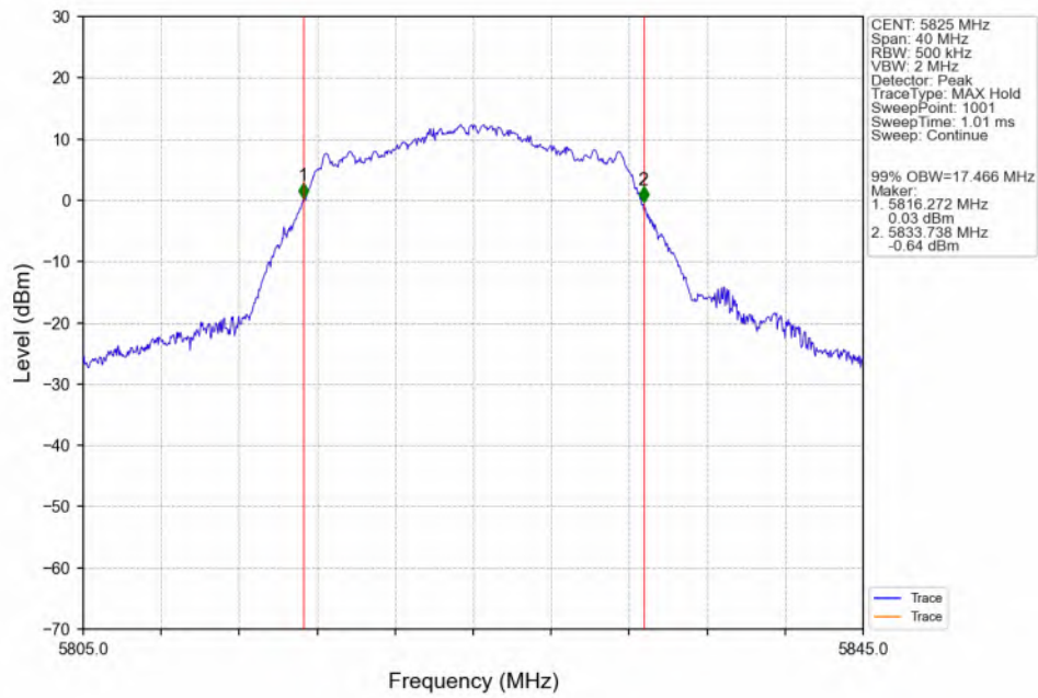
802.11a_HCH_5825MHz_ANT3_NTNV
