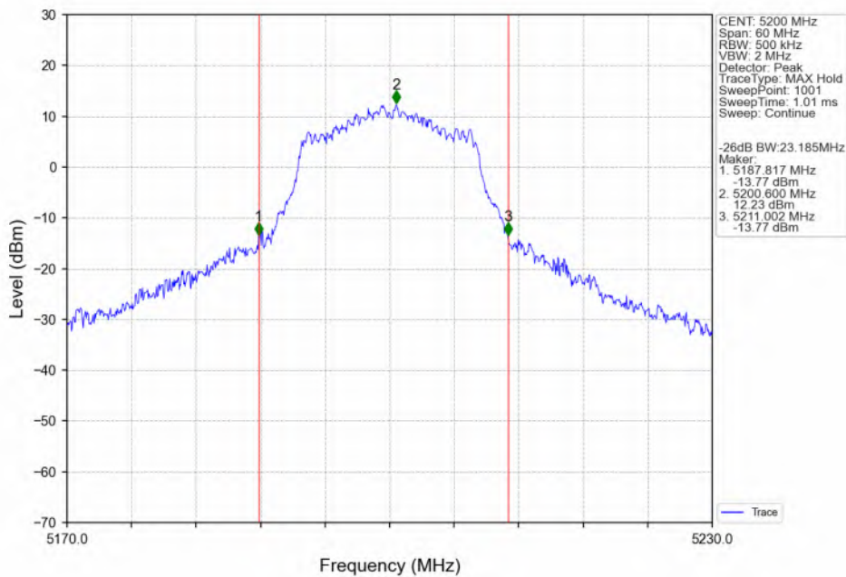
802.11a_MCH_5200MHz_ANT3_NTNV
