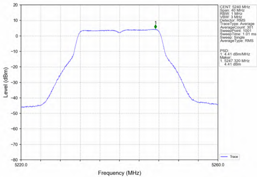
802.11a_HCH_5240MHz_ANT3_NTNV
