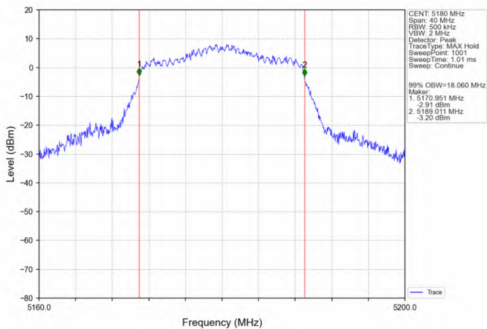
802.11n(HT20)_LCH_5180MHz_ANT3_NTNV
