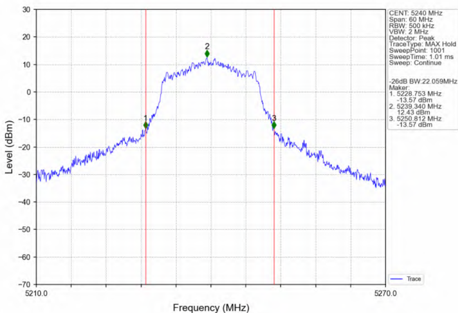
802.11a_HCH_5240MHz_ANT3_NTNV
