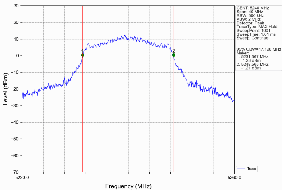
802.11a_HCH_5240MHz_ANT3_NTNV
