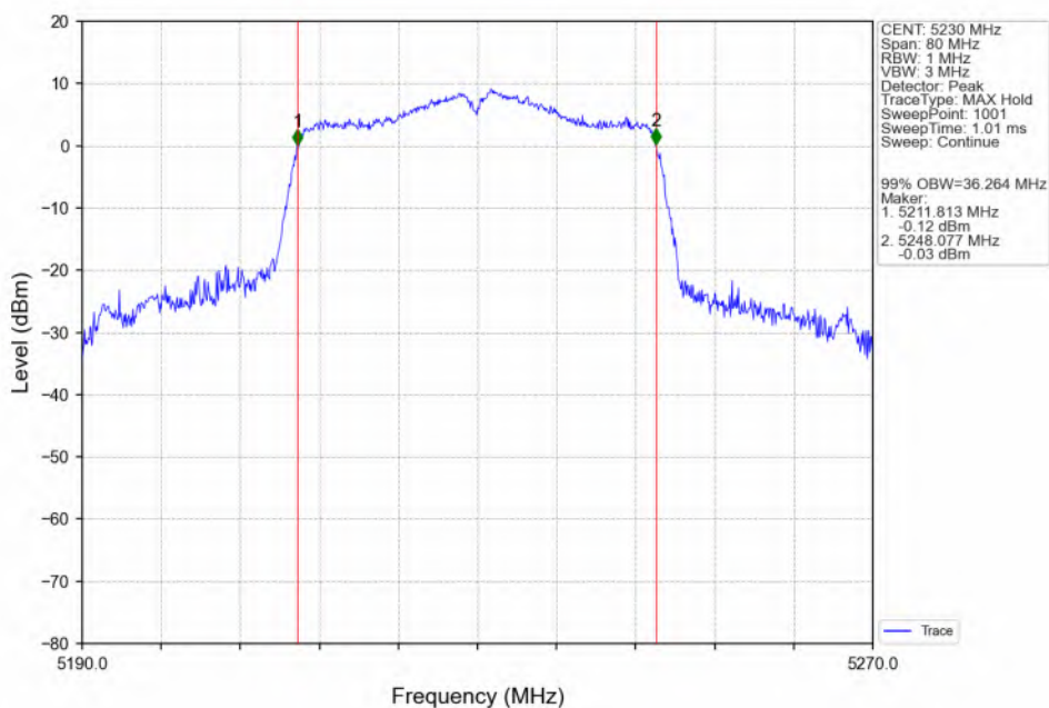
802.11n(HT40)_HCH_5230MHz_ANT3_NTNV
