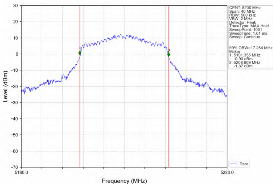
802.11a_MCH_5200MHz_ANT3_NTNV
