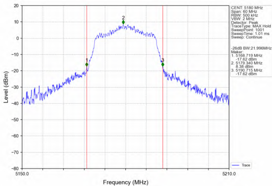
802.11n(HT20)_LCH_5180MHz_ANT3_NTNV
