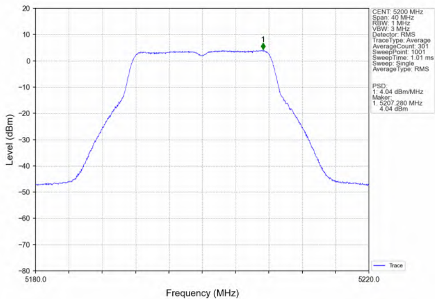
802.11a_MCH_5200MHz_ANT3_NTNV
