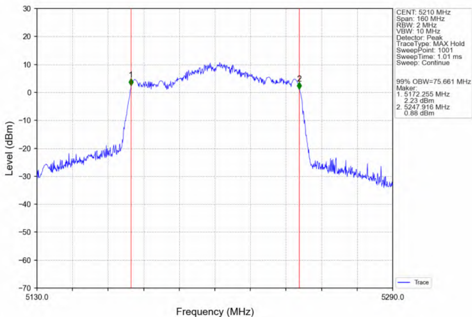
802.11ac(VHT80)_MCH_5210MHz_ANT3_NTNV
