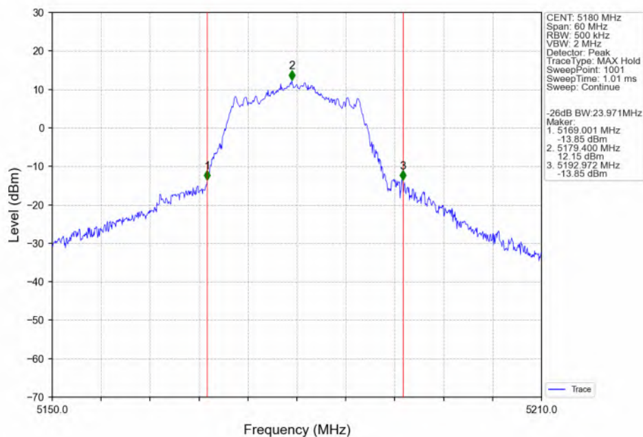
802.11a_LCH_5180MHz_ANT3_NTNV
