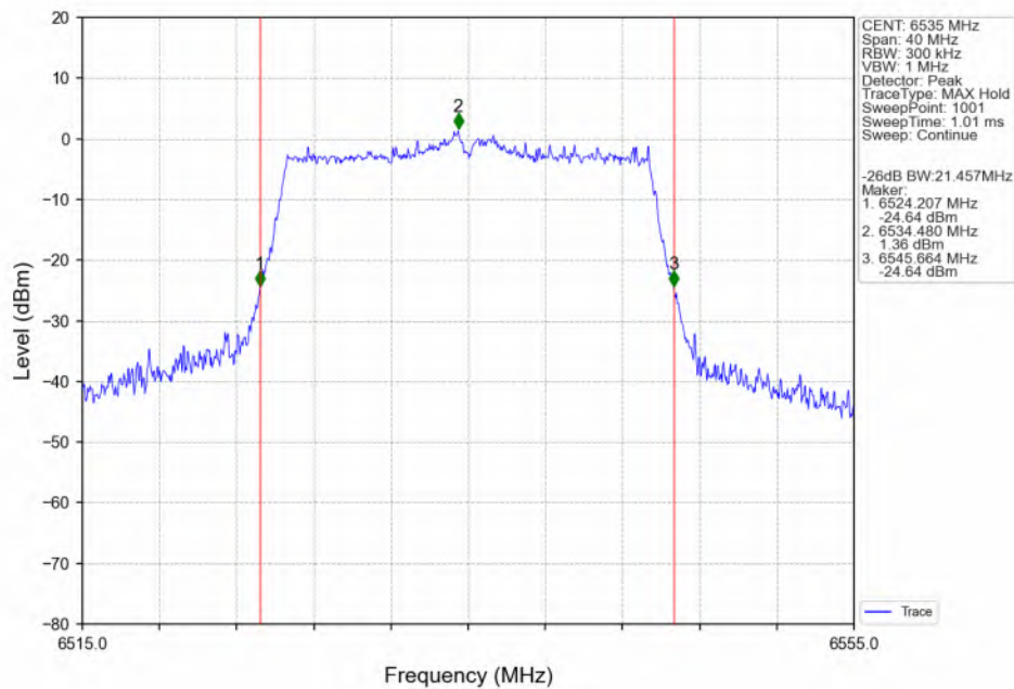
802.11ax(HEW20) LCH 6535MHz SU / ANT3 NTN
