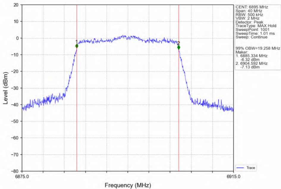
802.11ax(HEW20) LCH 6895MHz SU / ANT3 NTN
