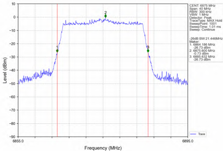
802.11ax(HEW20) HCH 6875MHz SU / ANT3 NTN
