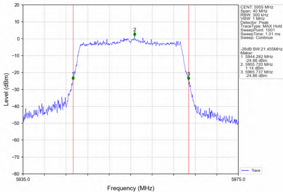
802.11ax(HEW20) LCH 5955MHz SU / ANT3 NTN
