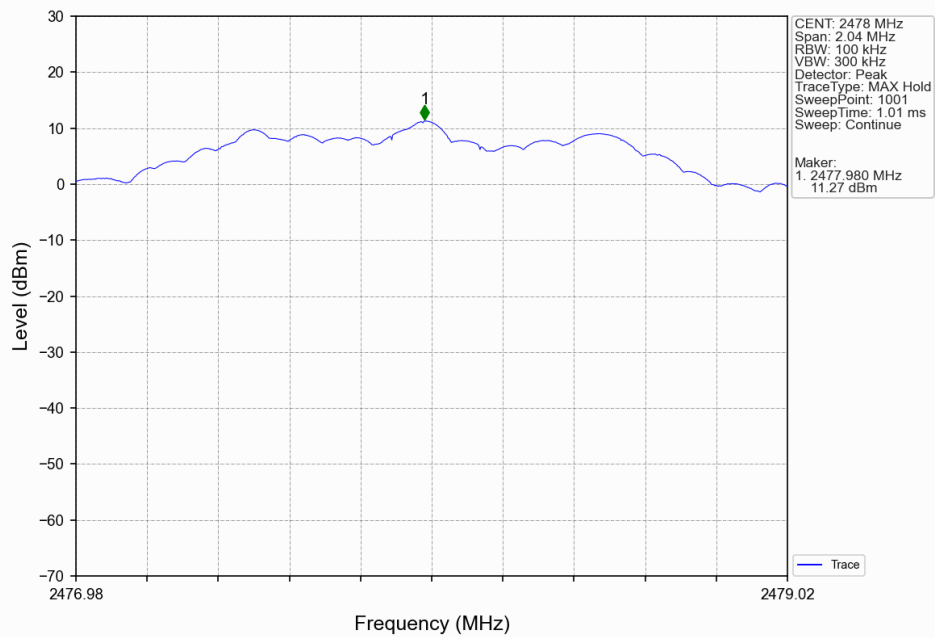
2M_HCH_2478MHz_Ant2_NTNV
