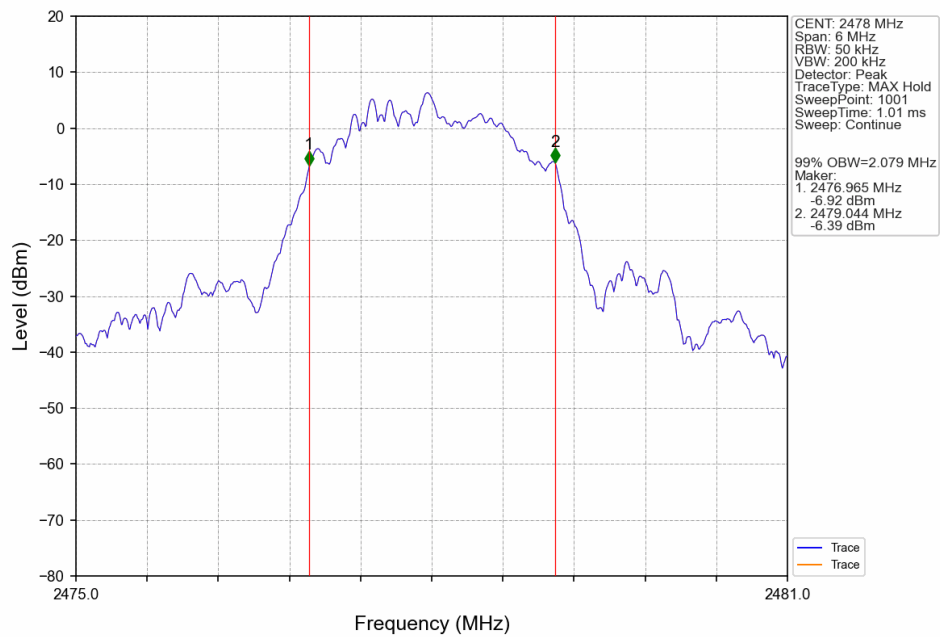
2M_HCH_2478MHz_Ant2_NTNV
