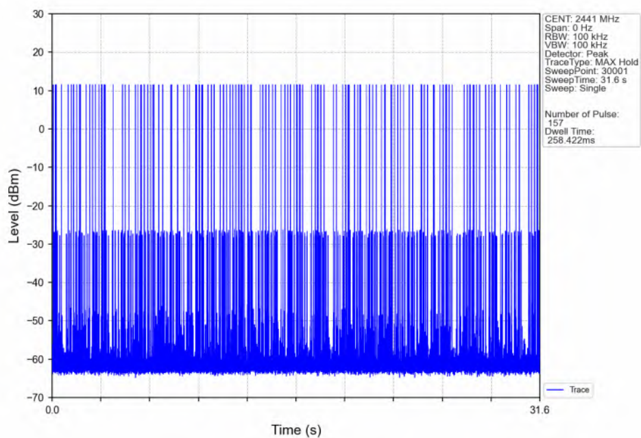
Pi/4DQPSK_2DH3_HOPP_Ant2_NTNV
