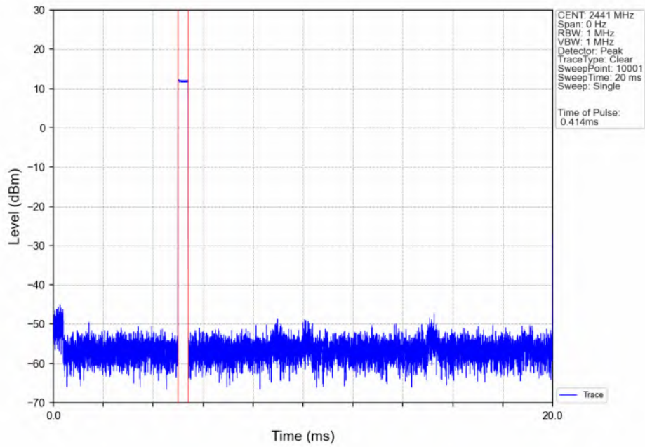
8DPSK_3DH1_HOPP_Ant2_NTNV
