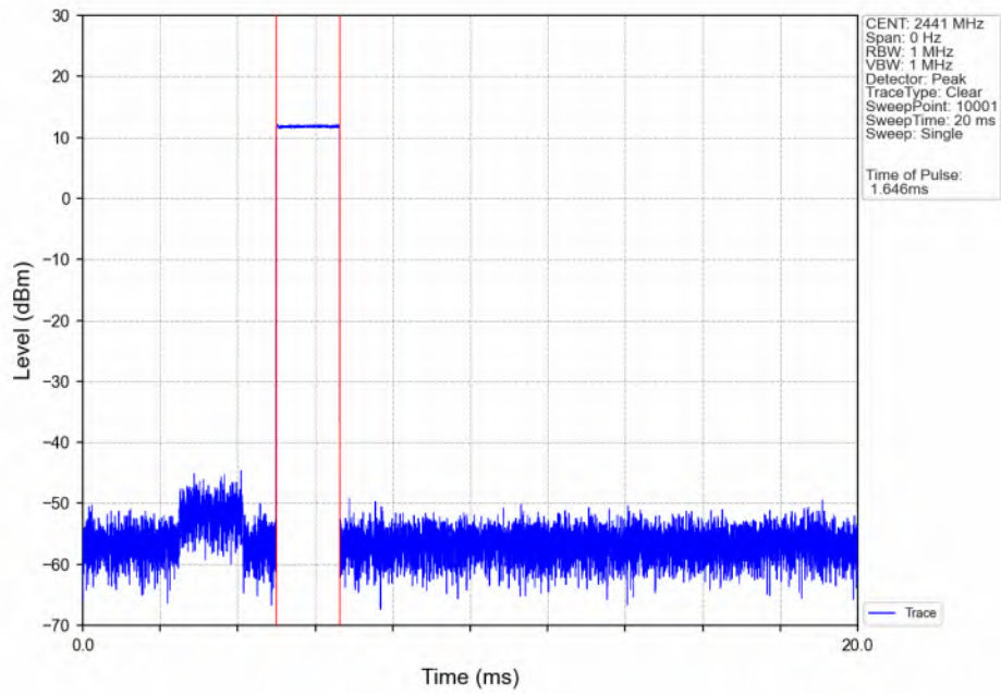
8DPSK_3DH3_HOPP_Ant2_NTNV
