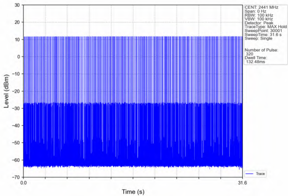
8DPSK_3DH1_HOPP_Ant2_NTNV
