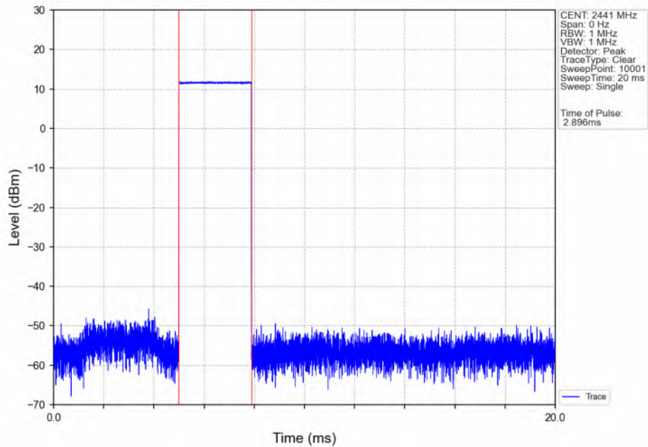
GFSK_DH5_HOPP_Ant2_NTNV
