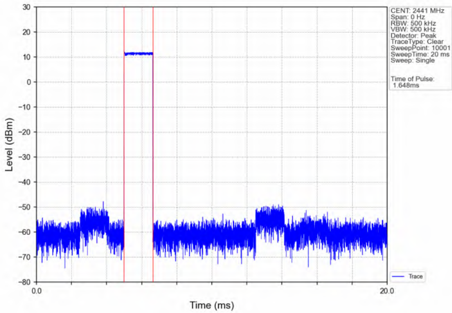
GFSK_DH3_HOPP_Ant2_NTNV
