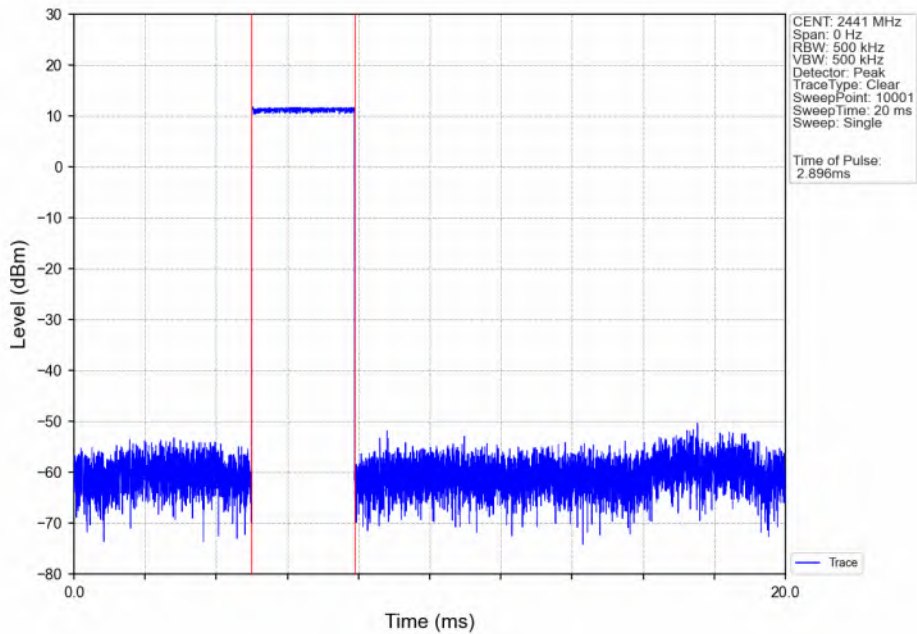
Pi/4DQPSK_2DH5_HOPP_Ant2_NTNV
