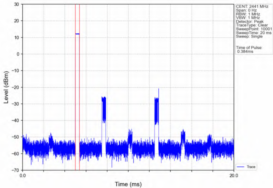
Pi/4DQPSK_2DH1_HOPP_Ant2_NTNV
