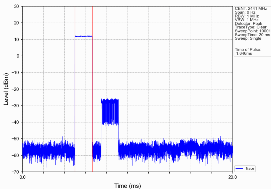
Pi/4DQPSK_2DH3_HOPP_Ant2_NTNV
