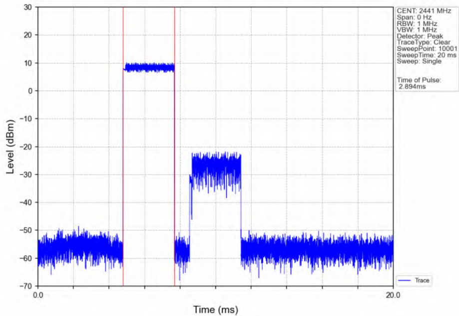
8DPSK_3DH5_HOPP_Ant2_NTNV
