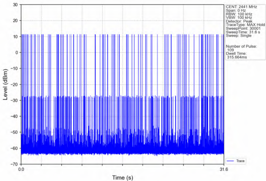
Pi/4DQPSK_2DH5_HOPP_Ant2_NTNV
