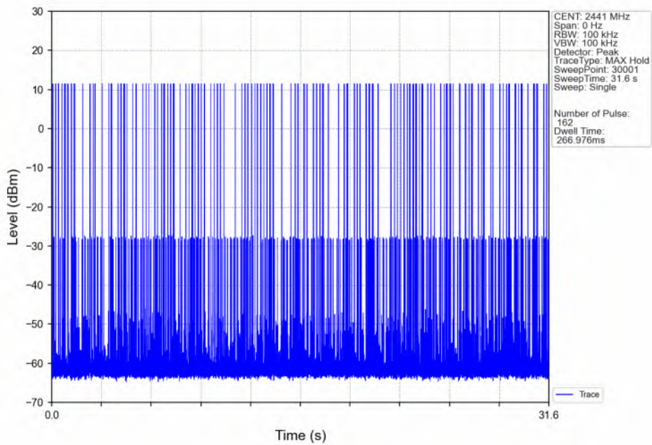
GFSK_DH3_HOPP_Ant2_NTNV
