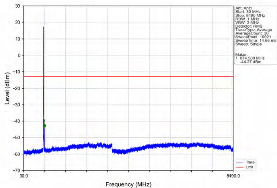
Band5_10MHz_QPSK_LCH_829MHz_RB_1_0_NTNV
