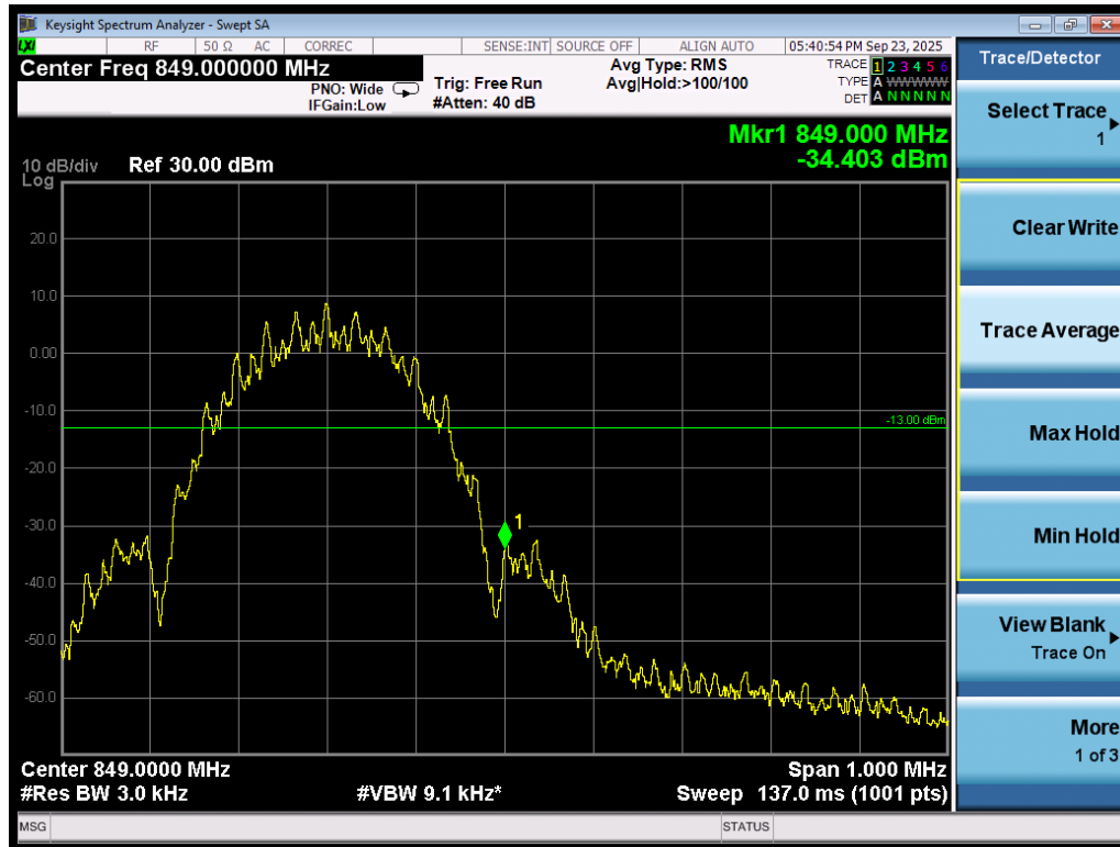
Band edge\GSM850\EGPRS\H
