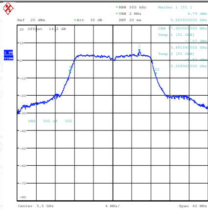
11A-Ant1-5500
