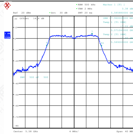
11A-Ant1-5580
