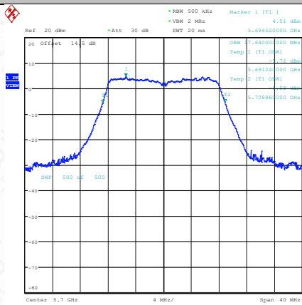
11A-Ant1-5700
