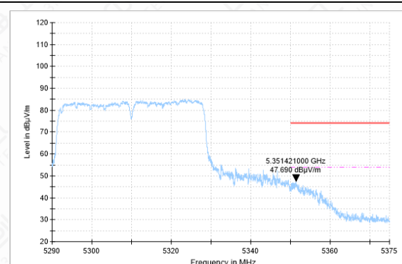
Bandedge-11AC(40M)-CH62-AV
