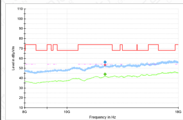
RSE-11AC-CH100-8GHz-18GHz
