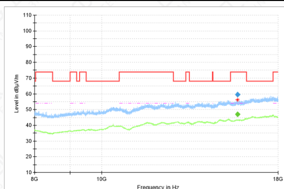
RSE-11N-CH40-8GHz-18GHz
