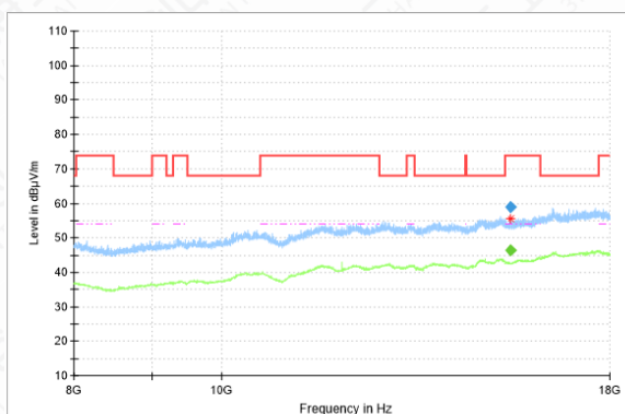
RSE-11N(40M)-CH62-8GHz-18GHz
