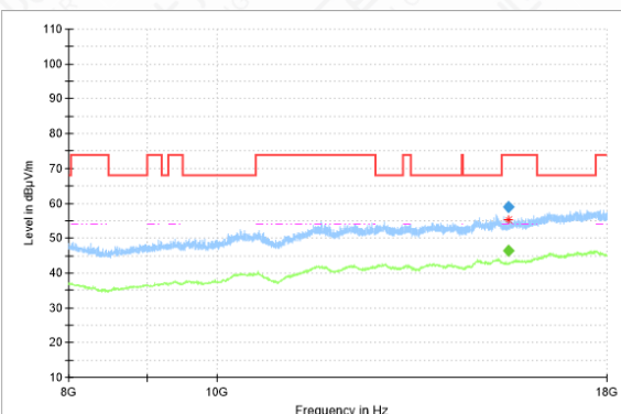
RSE-11N(40M)-CH134-8GHz-18GHz
