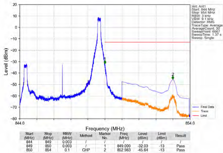
Band5_5MHz_QPSK_HCH_846.5MHz_RB_1_24_NTNV
