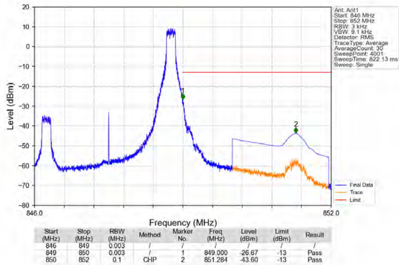
Band5_3MHz_QPSK_HCH_847.5MHz_RB_1_14_NTNV
