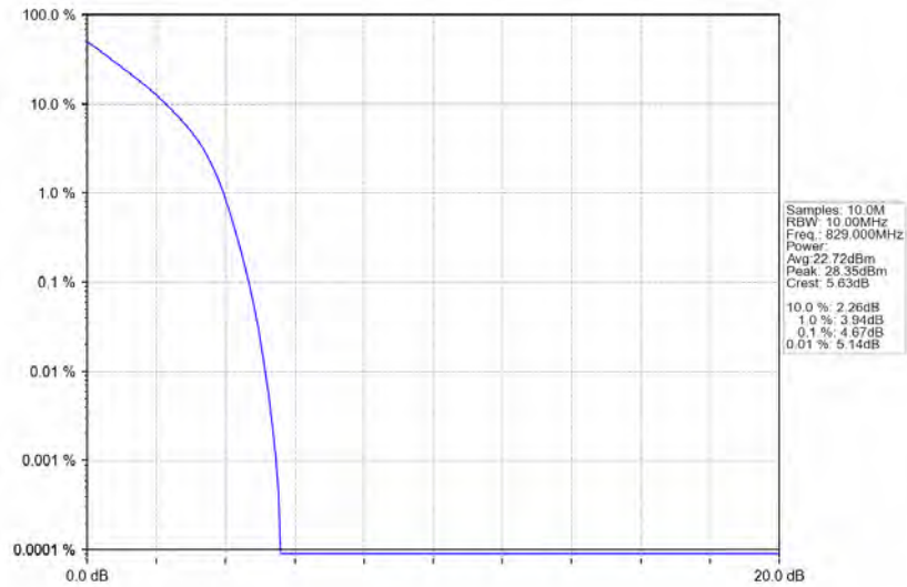
Band5_10MHz_QPSK_LCH_829MHz_RB_50_0_NTNV
