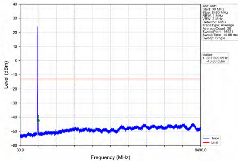
Band5_10MHz_QPSK_HCH_844MHz_RB_1_49_NTNV
