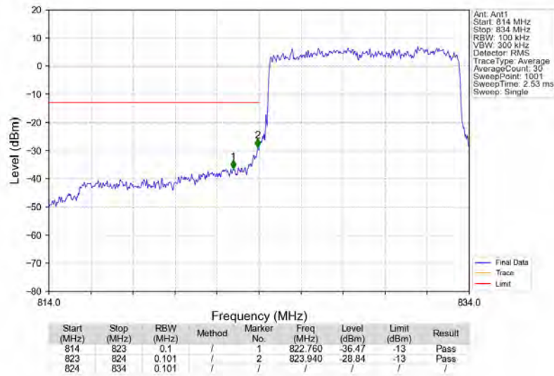
Band5_10MHz_QPSK_LCH_829MHz_RB_50_0_NTNV
