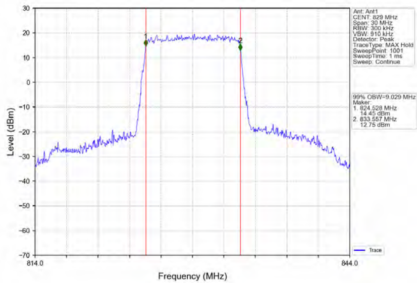
Band5_10MHz_QPSK_LCH_829MHz_RB_50_0_NTNV
