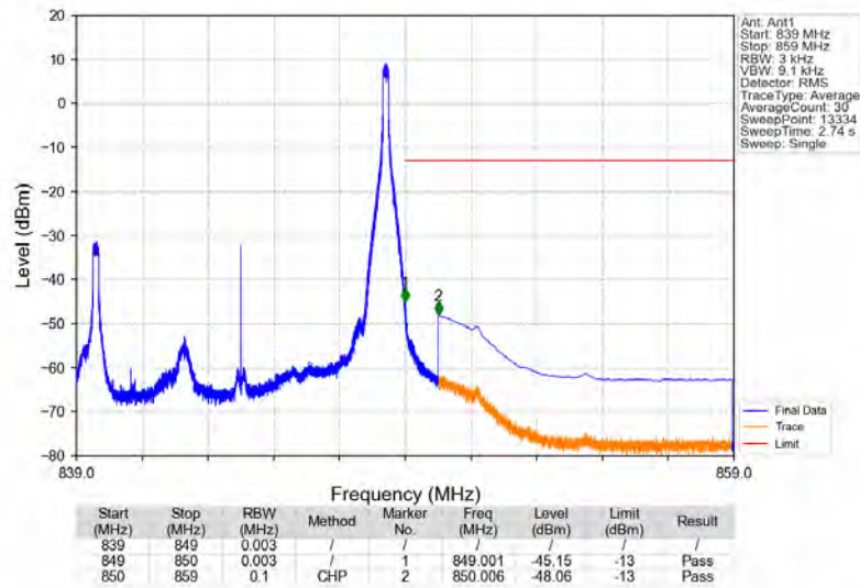
Band5_10MHz_QPSK_HCH_844MHz_RB_1_49_NTNV
