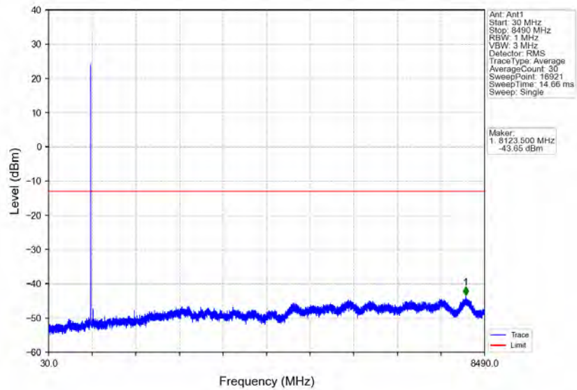
Band5_3MHz_QPSK_HCH_847.5MHz_RB_1_14_NTNV
